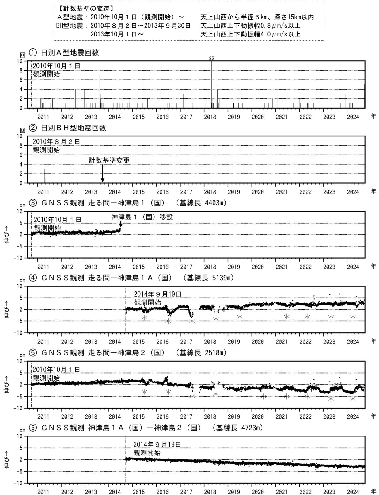
図2 神津島 火山活動経過図(2010年8月2日～2024年9月30日)
