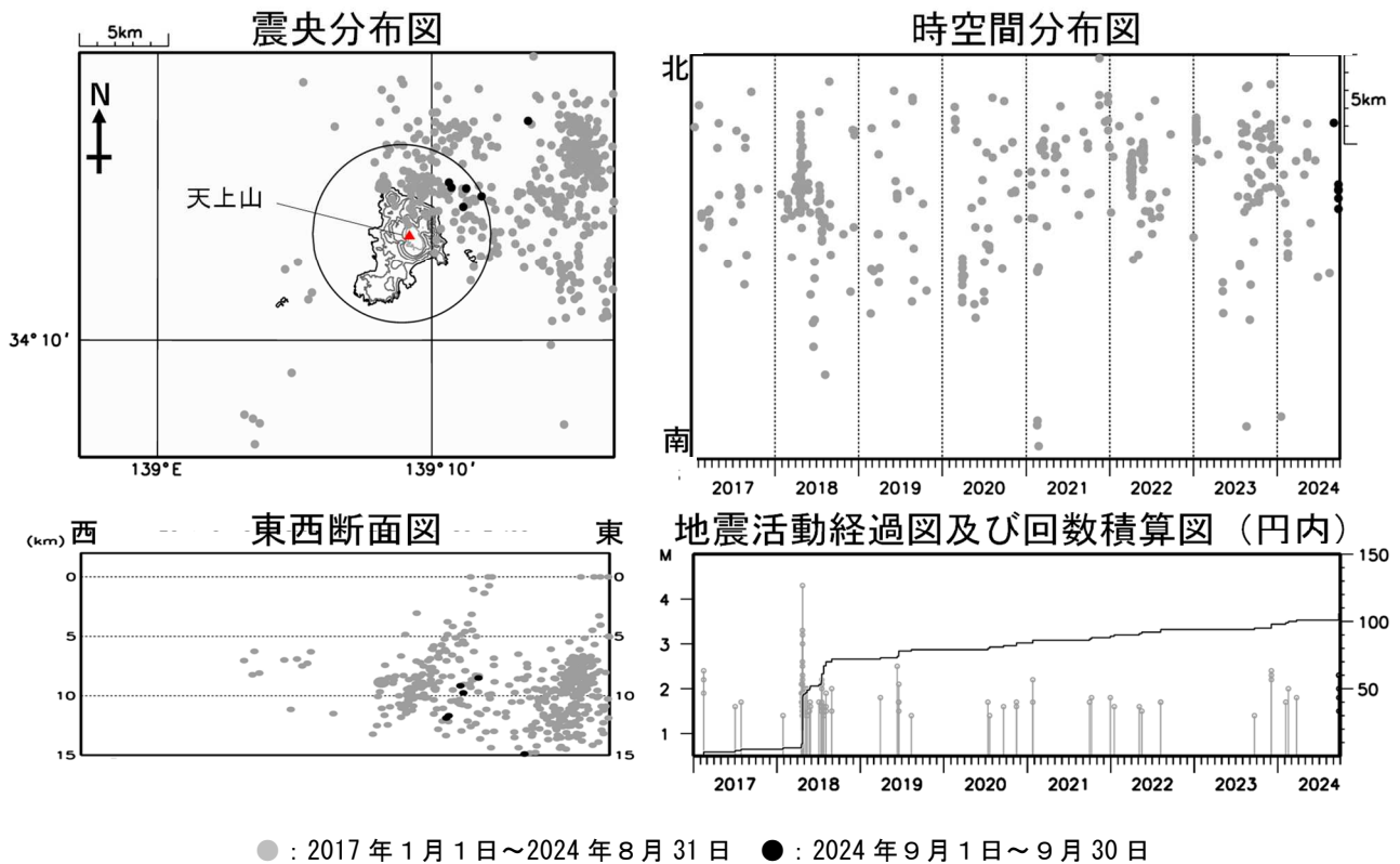
図3 神津島 広域地震観測網による山体・周辺の地震活動（2017年1月1日～2024年9月30日）
