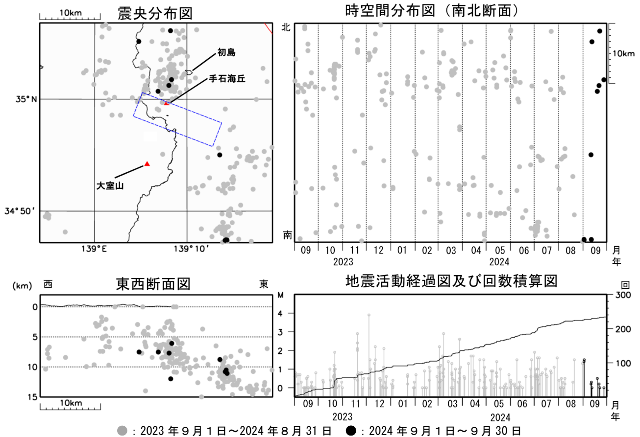
図2 伊豆東部火山群 広域地震観測網による震源分布図（2023 年 9 月 1 日～2024 年 9 月 30 日） □ の領域は群発地震活動の発生する可能性がある範囲（火口が出現する可能性のある範囲）を示しています。 https://www.data.jma.go.jp/vois/data/tokyo/STOCK/level/PDF/level_316.pdf 広域地震観測網により震源決定したもので、深さは全て海面以下として決定しています。 M（マグニチュード）は地震の規模を表し、M0.0 以上を表示しています。 図中の震源要素は一部暫定値が含まれており、後日変更することがあります。 この図では、関係機関の地震波形を一元的に処理し、地震観測点の標高を考慮する等した手法で得られた震源を用いています。
