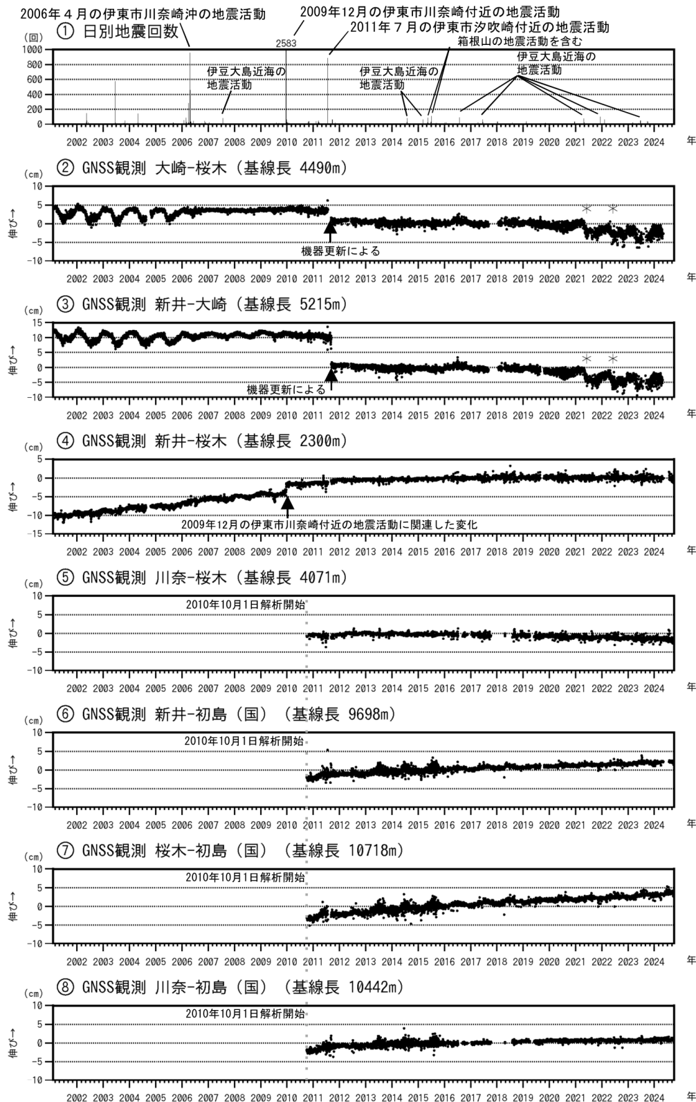
図3 伊豆東部火山群 火山活動経過図（2001年2月1日～2024年9月30日）
