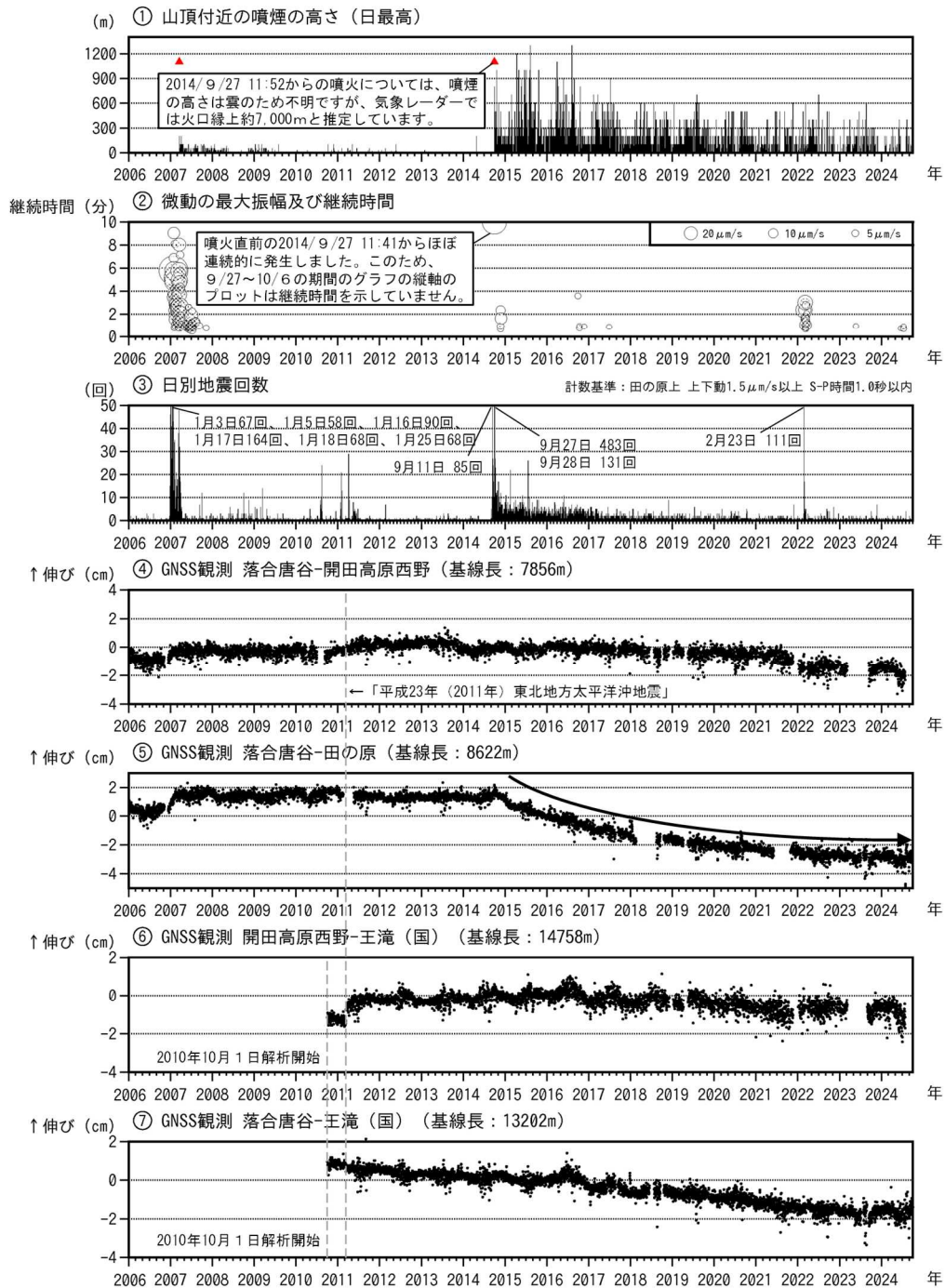
図1 御嶽山 長期間の火山活動経過図（2006年1月1日～2024年9月30日）
