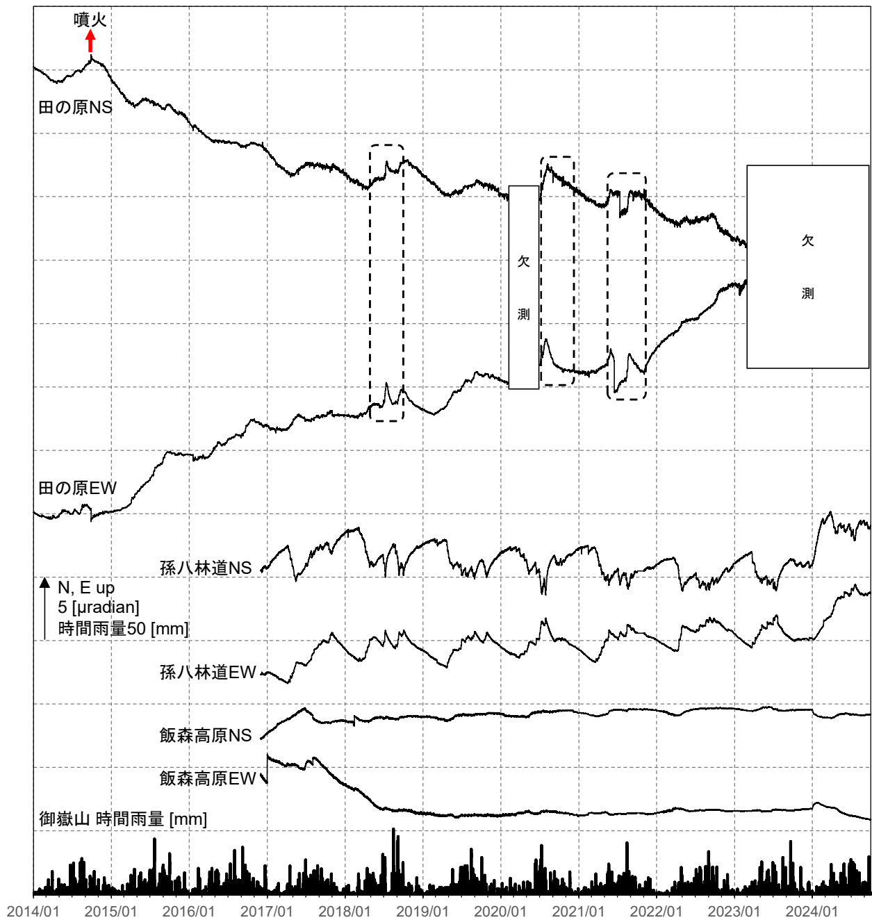
図6 御嶽山 傾斜変動（2014年1月1日～2024年9月30日）
