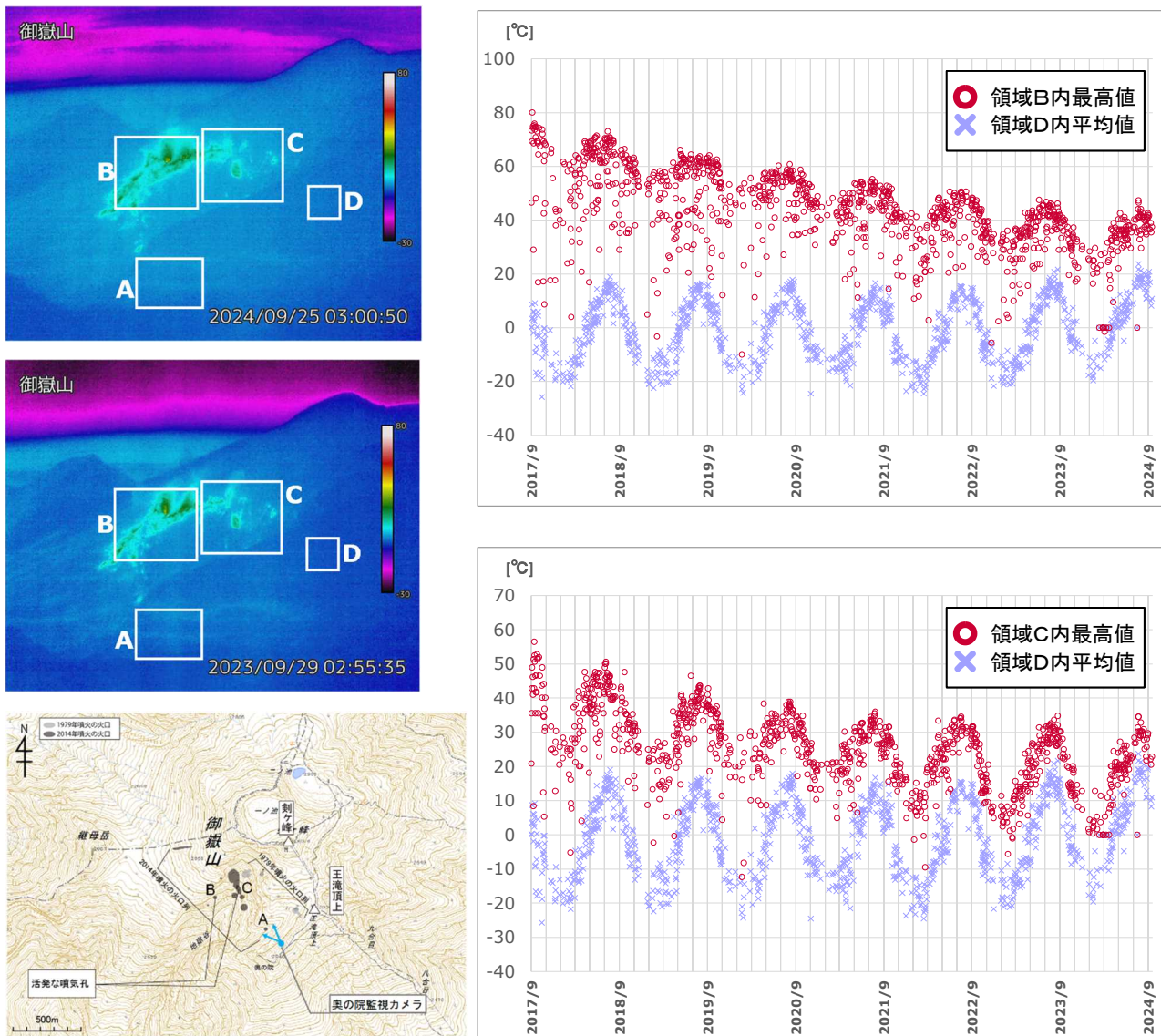
図3 御嶽山 奥の院赤外熱映像カメラによる剣ヶ峰南西側における最高温度の推移 (2017年9月13日～2024年9月30日)
