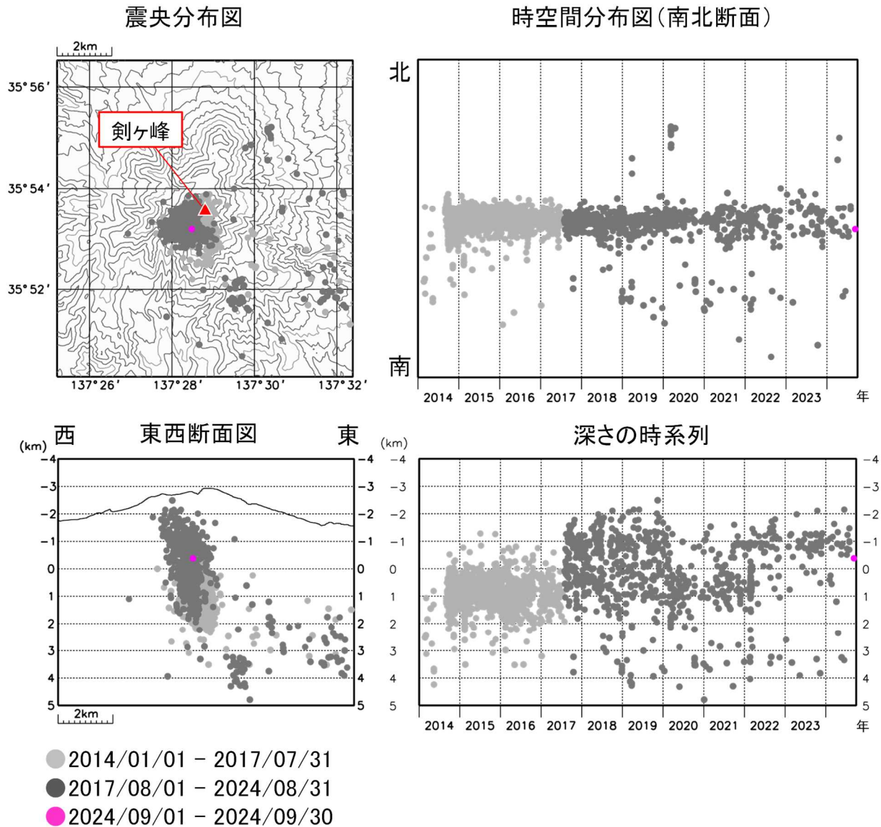
図4 御嶽山 震源分布図（2014年1月1日～2024年9月30日）
