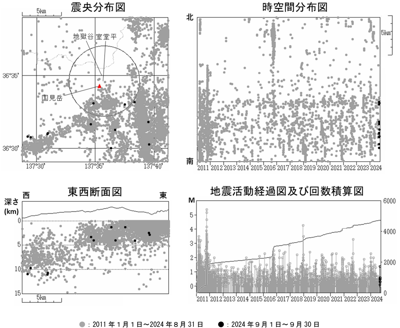
図2 弥陀ヶ原 広域地震観測網による山体・周辺の地震活動（2011 年 1 月 1 日～2024 年 9 月 30 日） 震央分布図中の円は弥陀ヶ原の計数対象地震（室堂平で S-P 時間 1 秒以内）のおよその範囲を示しています。 広域地震観測網により震源決定したもので、深さは全て海面以下として決定しています。 図中の震源要素は一部暫定値が含まれており、後日変更することがあります。 この図では、関係機関の地震波形を一元的に処理し、地震観測点の標高を考慮する等した手法で得られた震源を用いています（ただし、2020 年 8 月以前の地震については火山活動評価のための参考震源です）。
