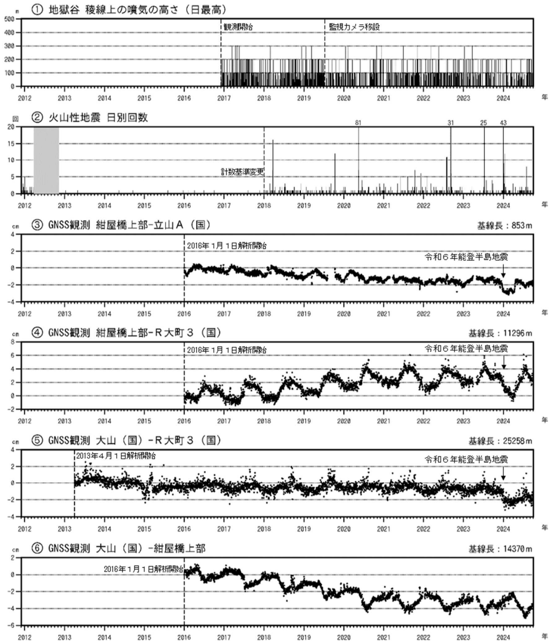
図3 弥陀ヶ原 火山活動経過図（2011年12月1日～2024年9月30日）
