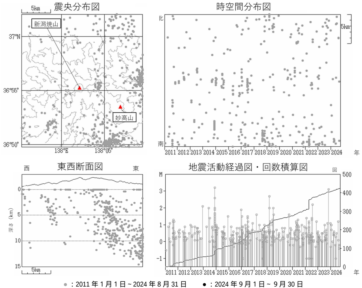
図8 新潟焼山 広域地震観測網による山体・周辺の地震活動（2011年1月1日～2024年9月30日） 広域地震観測網により震源決定したもので、深さは全て海面以下として決定しています。 図中の震源要素は一部暫定値が含まれており、後日変更することがあります。 この図では、関係機関の地震波形を一元的に処理し、地震観測点の標高を考慮する等した手法で得られた震源を用いています（ただし、2020年8月以前の地震については火山活動評価のための参考震源です）。
