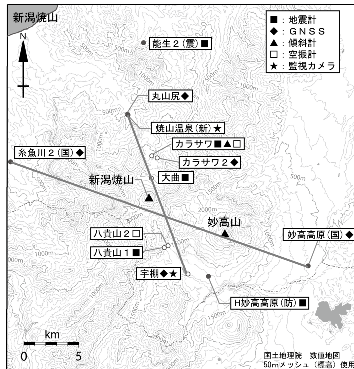
図11 新潟焼山 観測点配置図 GNSS 基線 は図6の に対応しています。
