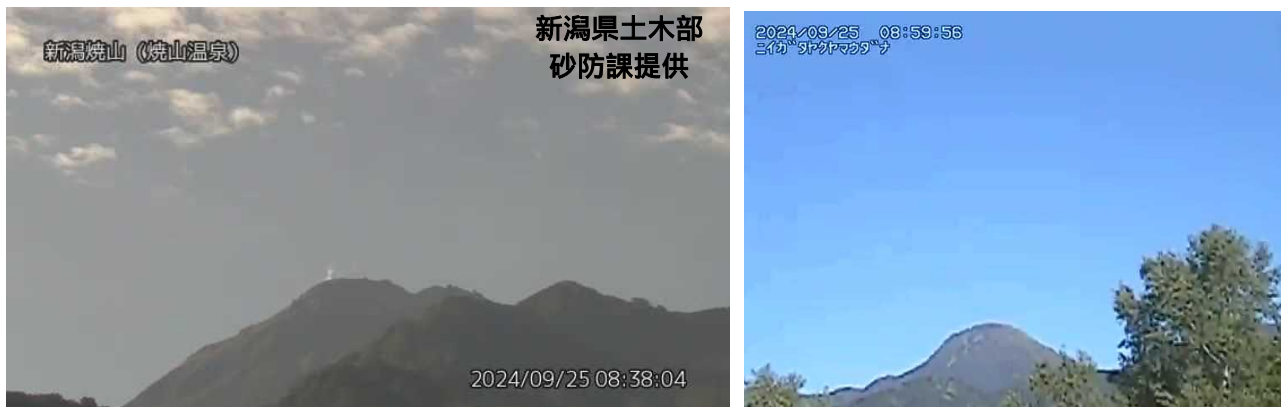
図1 新潟焼山 山頂部の噴煙の状況 （左：焼山温泉監視カメラ（9月25日） 右：宇棚監視カメラ（9月25日）による）
