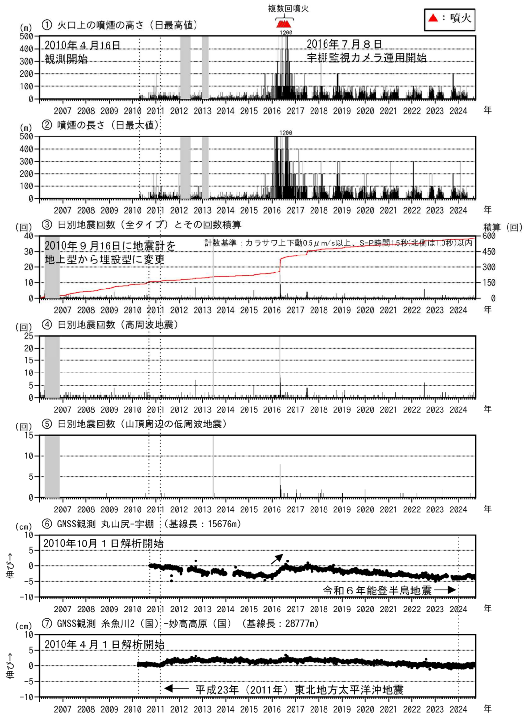
図6 新潟焼山 火山活動経過図（2006年1月1日～2024年9月30日）
