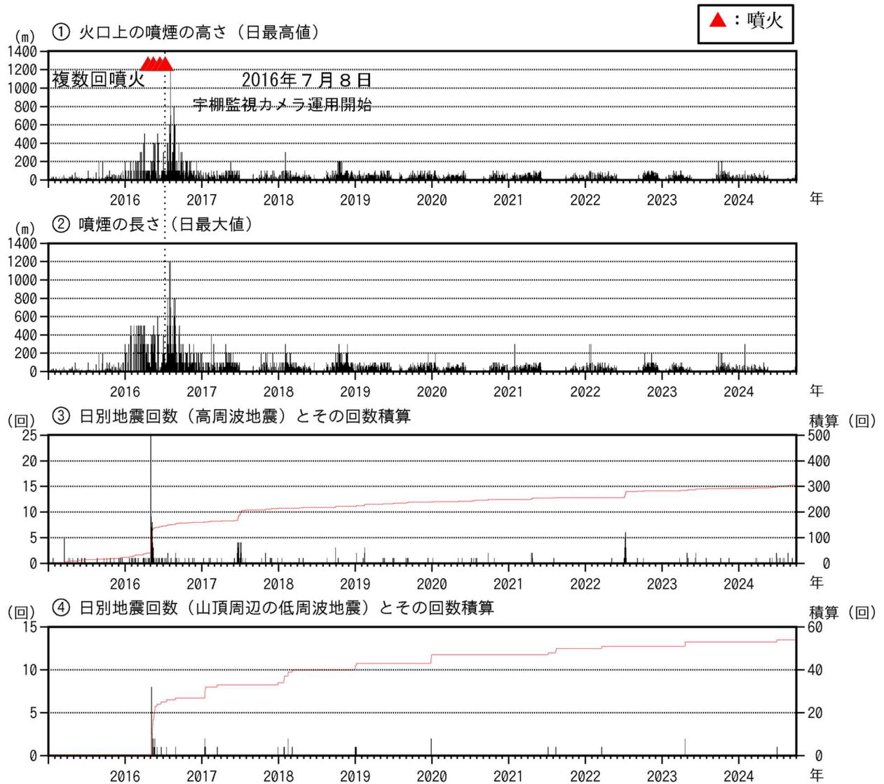
図7 新潟焼山 火山活動経過図（短期）（2015年1月1日～2024年9月30日）
