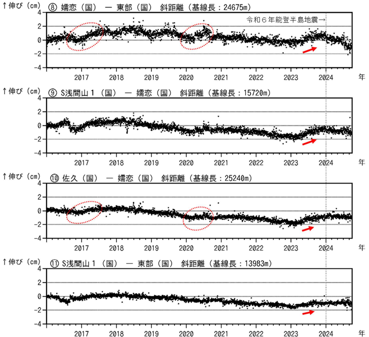
図7-2 浅間山 GNSS 連続観測結果(2016年1月1日～2024年9月30日)
