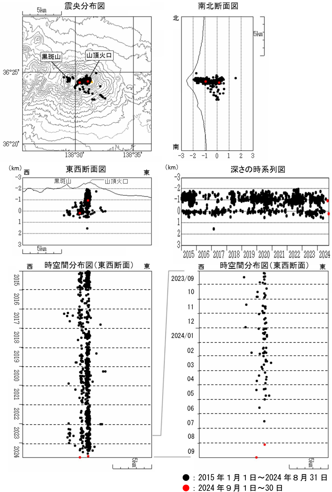
図5 浅間山 震源分布図（2015 年 1 月 1 日～2024 年 9 月 30 日）
