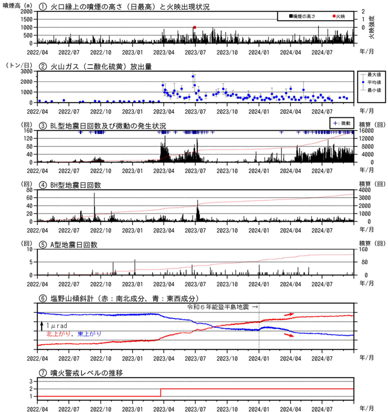
図2 浅間山 短期火山活動経過図（2022年4月1日～2024年9月30日）
