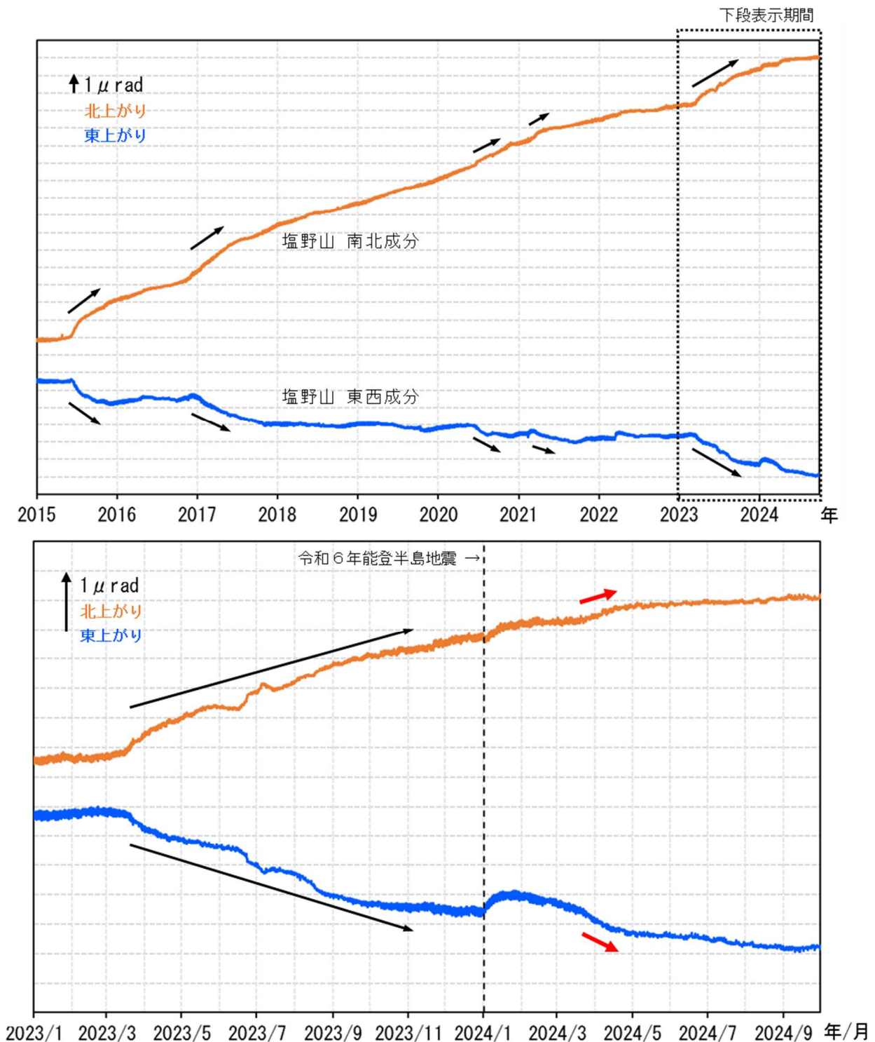
図6 浅間山 塩野山観測点における傾斜データ（2015年1月1日～2024年9月30日）
