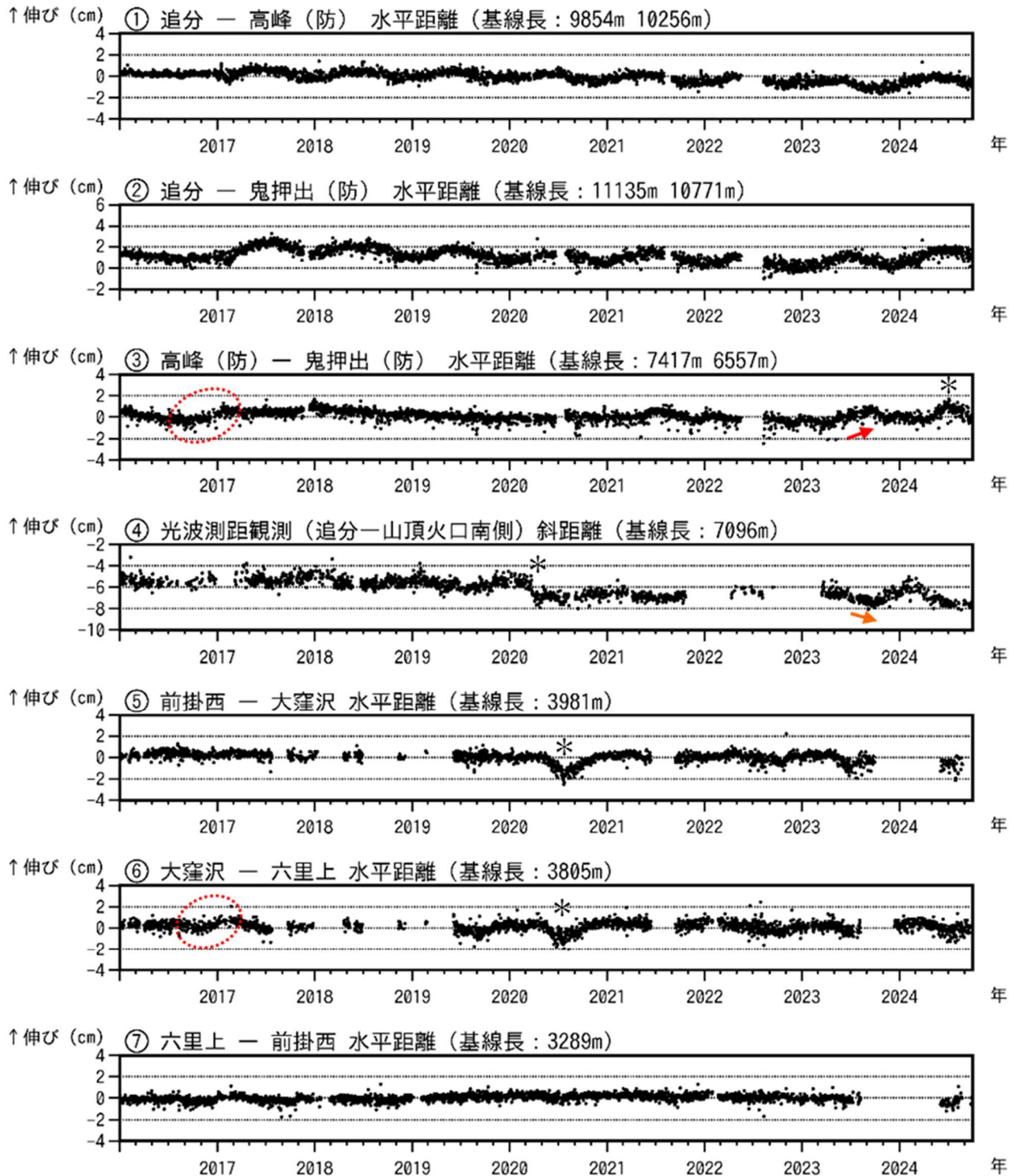
図7-1 浅間山 GNSS 連続観測及び光波測距観測結果(2016年1月1日～2024年9月30日)
