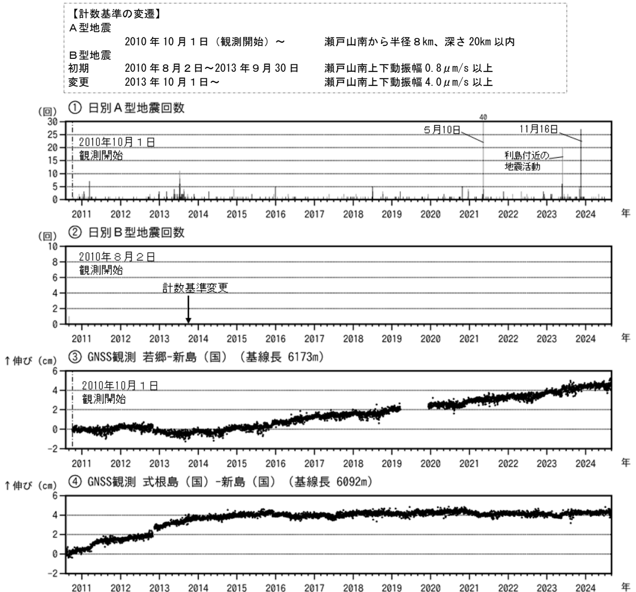
図2 新島 火山活動経過図(2010年8月2日～2024年8月31日)
