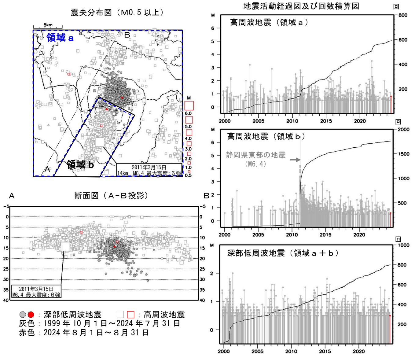
図3 富士山 広域地震観測網による山体及び周辺の地震活動（1999年10月1日～2024年8月31日）
