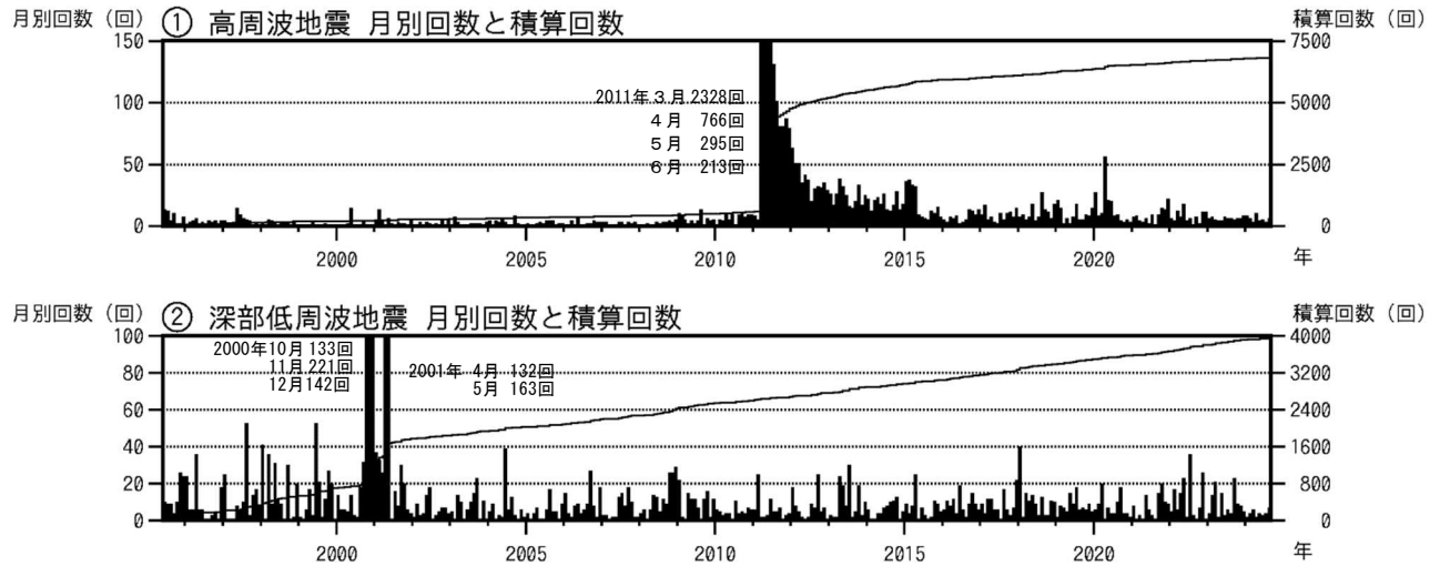
図2 富士山 月別地震回数（1995年6月1日～2024年8月31日）
