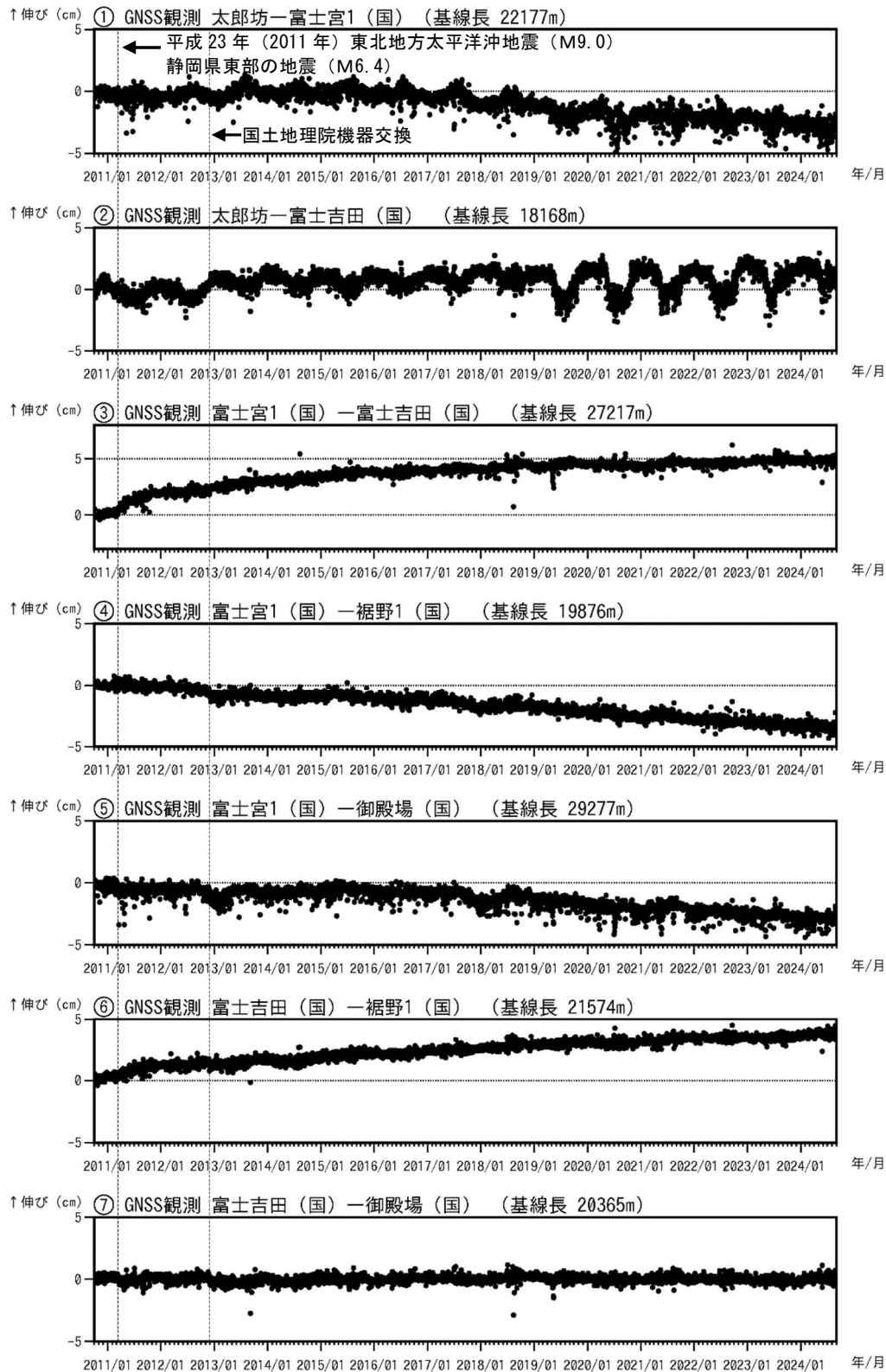
図4 富士山 GNSS 連続観測による基線長変化（2010年10月1日～2024年8月31日） （国）：国土地理院 「平成23年（2011年）東北地方太平洋沖地震」及び2011年3月15日に発生した静岡県東部の地震（M6.4）によるステップ状の変化を補正しています。 ①～⑦は図5のGNSS基線①～⑦に対応しています。
