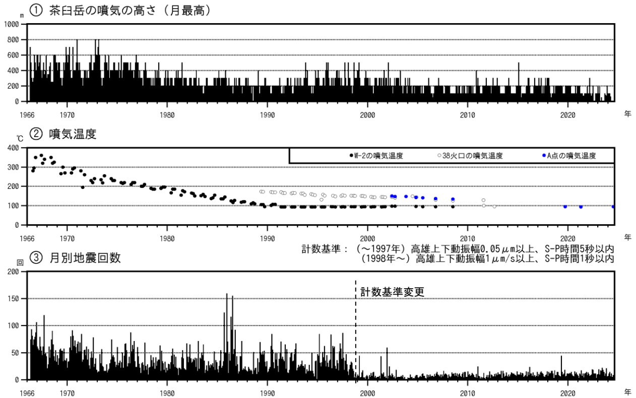
図3-1 那須岳 火山活動経過図（1966年6月～2024年8月）
