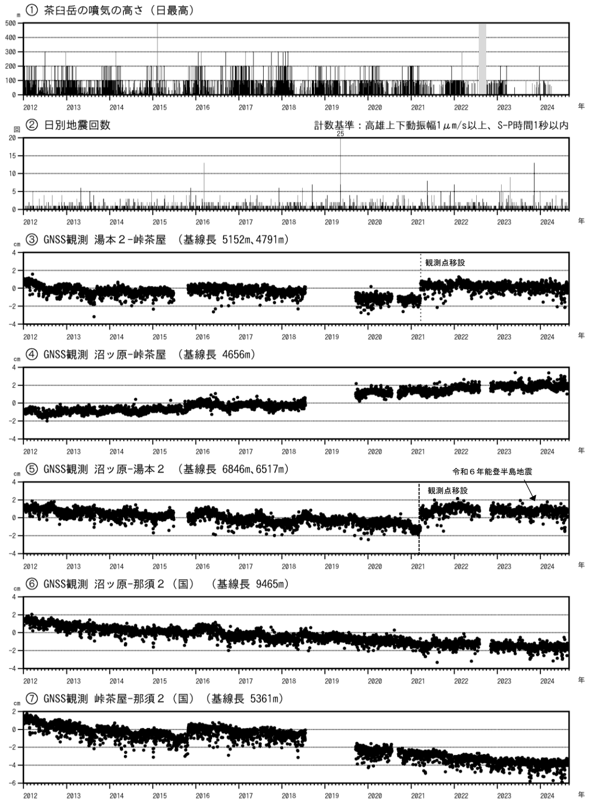
図4 那須岳 火山活動経過図（2012年1月1日～2024年8月31日）
