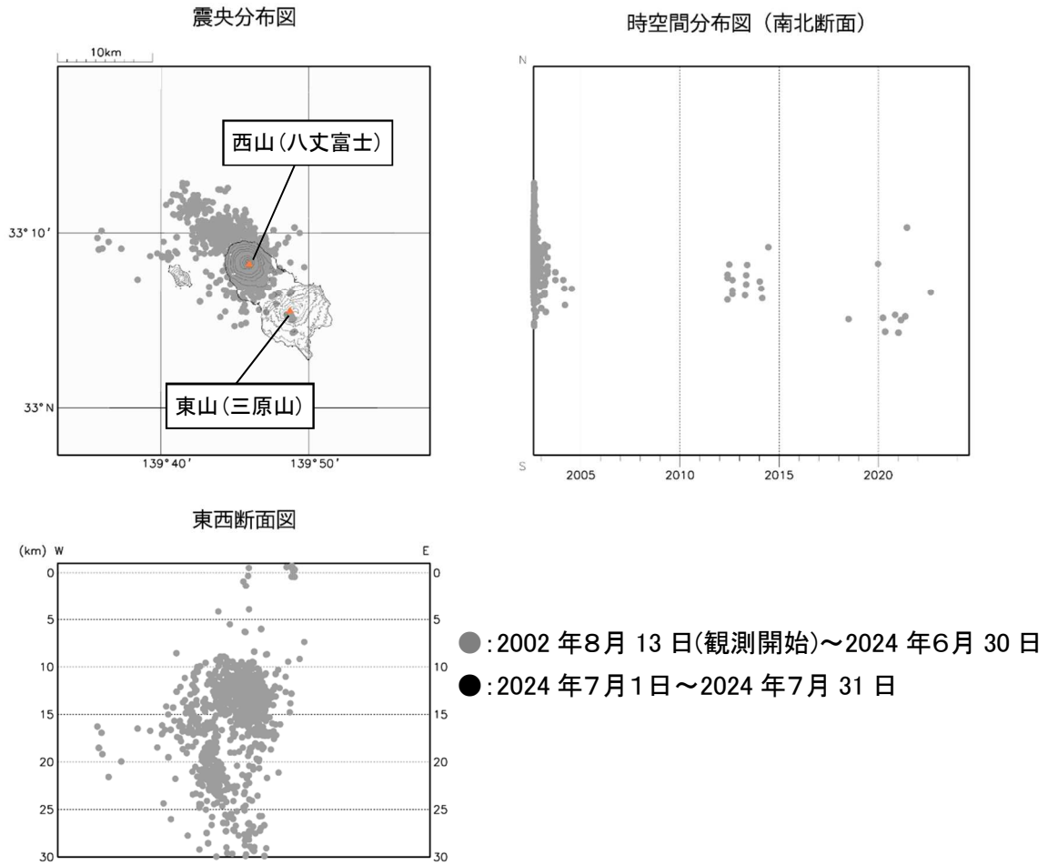
図3 八丈島 震源分布図（2002 年 8 月 13 日～2024 年 7 月 31 日）
