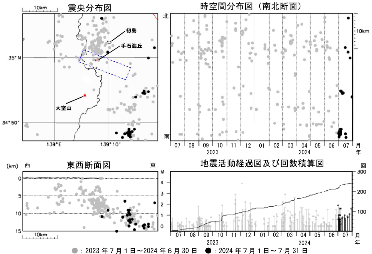
図2 伊豆東部火山群 広域地震観測網による震源分布図（2023 年 7 月 1 日～2024 年 7 月 31 日） □ の領域は群発地震活動の発生する可能性がある範囲（火口が出現する可能性のある範囲）を示しています。 https://www.data.jma.go.jp/vois/data/tokyo/STOCK/level/PDF/level_316.pdf 広域地震観測網により震源決定したもので、深さは全て海面以下として決定しています。 M（マグニチュード）は地震の規模を表し、M0.0 以上を表示しています。 図中の震源要素は一部暫定値が含まれており、後日変更することがあります。 この図では、関係機関の地震波形を一元的に処理し、地震観測点の標高を考慮する等した手法で得られた震源を用いています。
