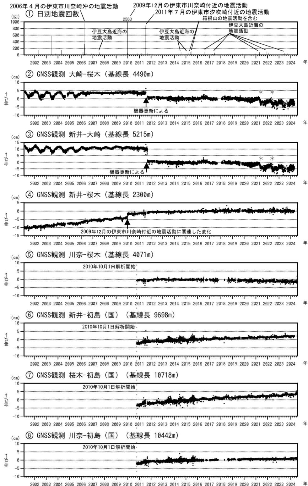
図3 伊豆東部火山群 火山活動経過図（2001年2月1日～2024年7月31日）
