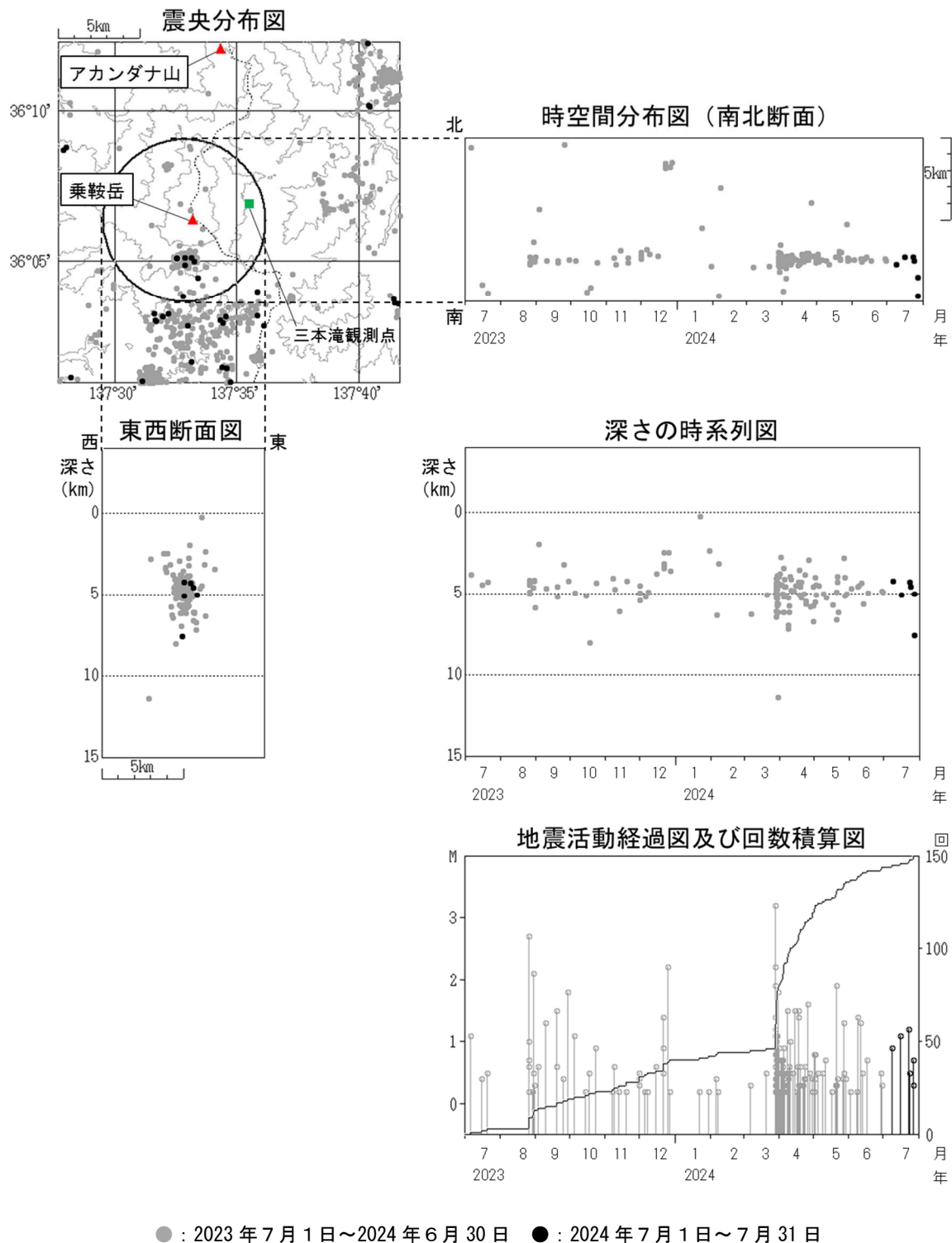
図3 乗鞍岳 広域地震観測網による山体・周辺の地震活動(2023年7月1日～2024年7月31日)
