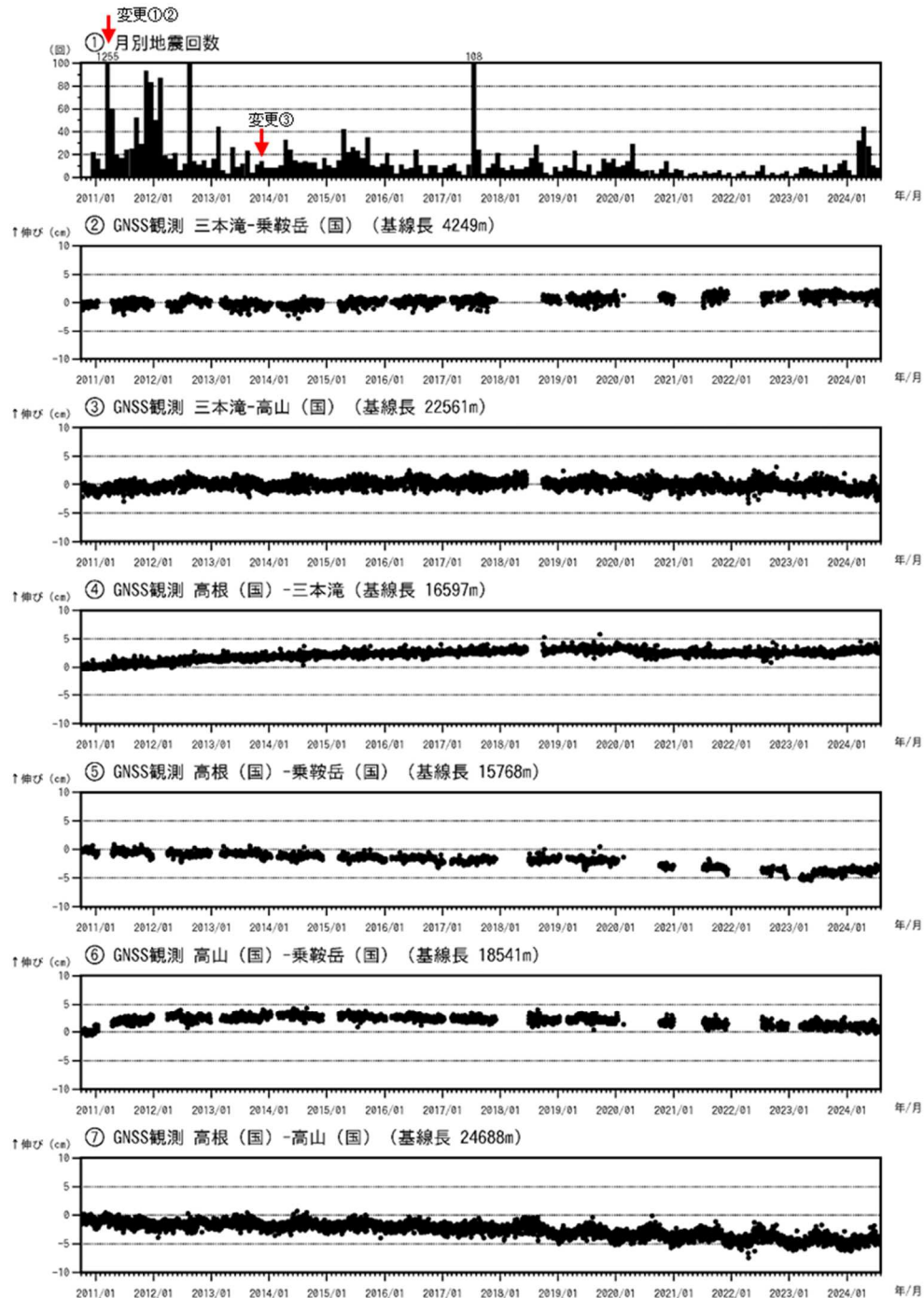
図2 乗鞍岳 火山活動経過図（2010年10月1日～2024年7月31日）
