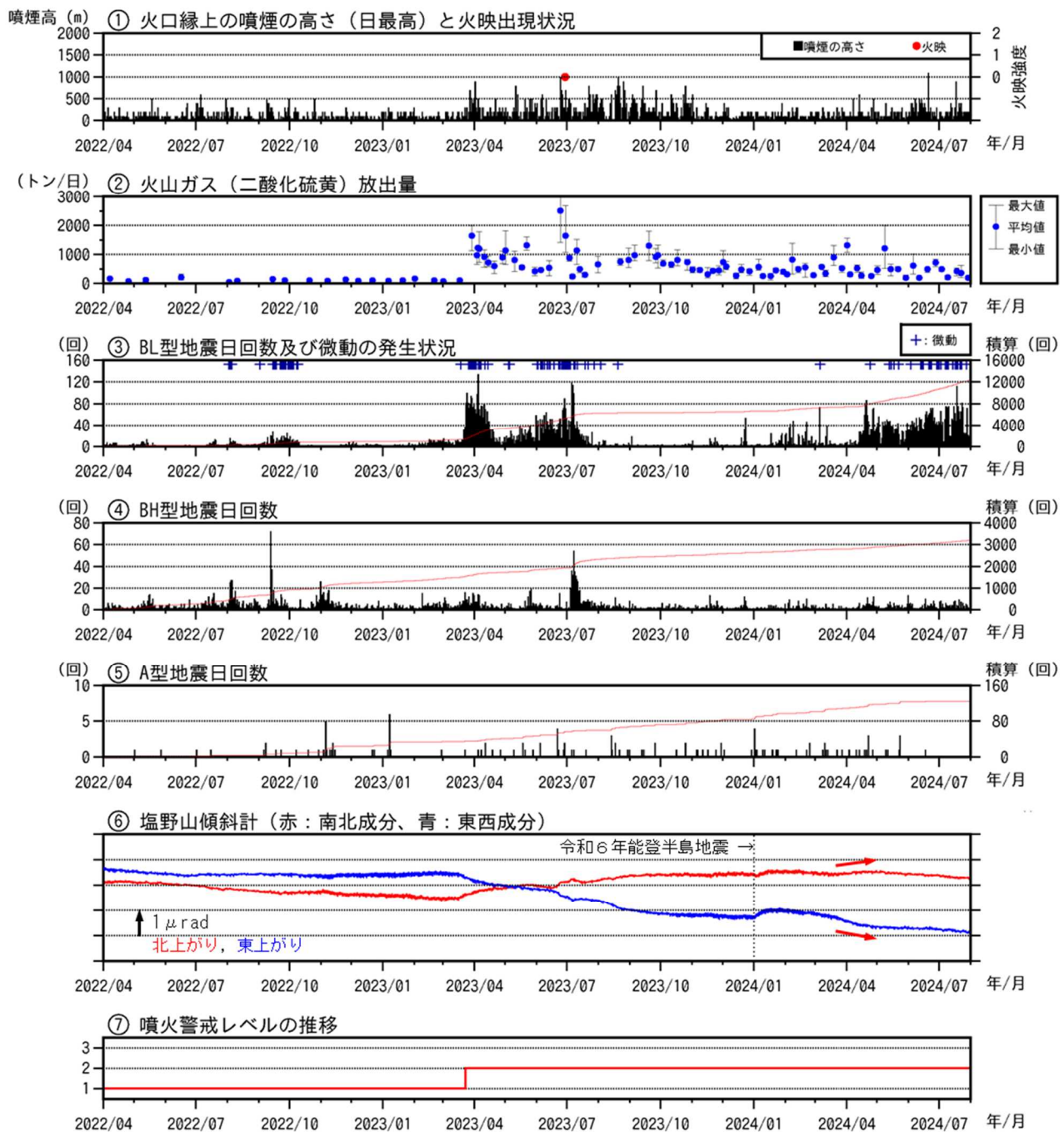
図2 浅間山 短期火山活動経過図（2022年4月1日～2024年7月31日）
