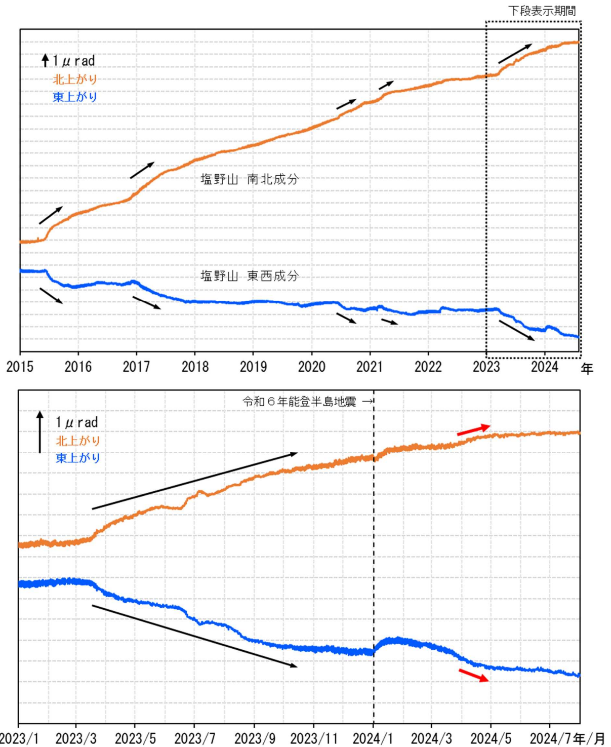
図6 浅間山 塩野山観測点における傾斜データ（2015年1月1日～2024年7月31日）
