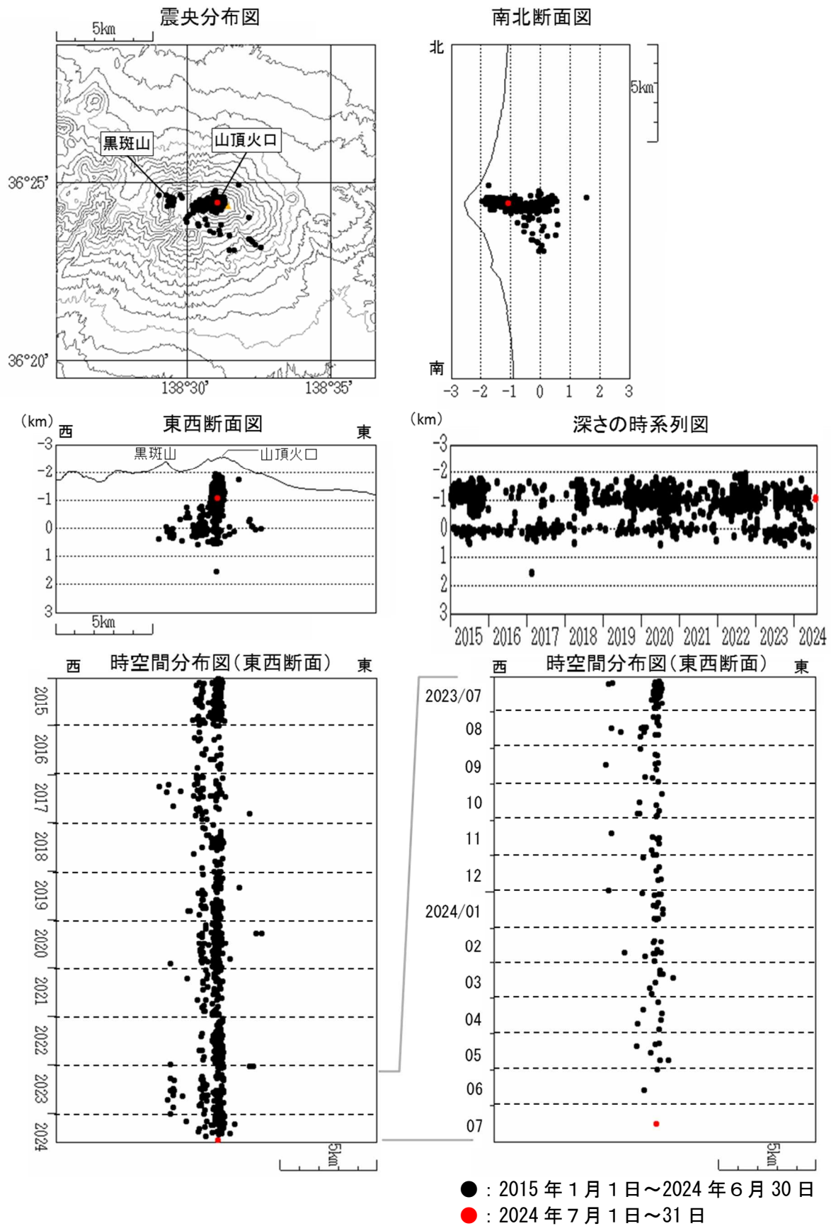
図5 浅間山 震源分布図（2015 年 1 月 1 日～2024 年 7 月 31 日）
