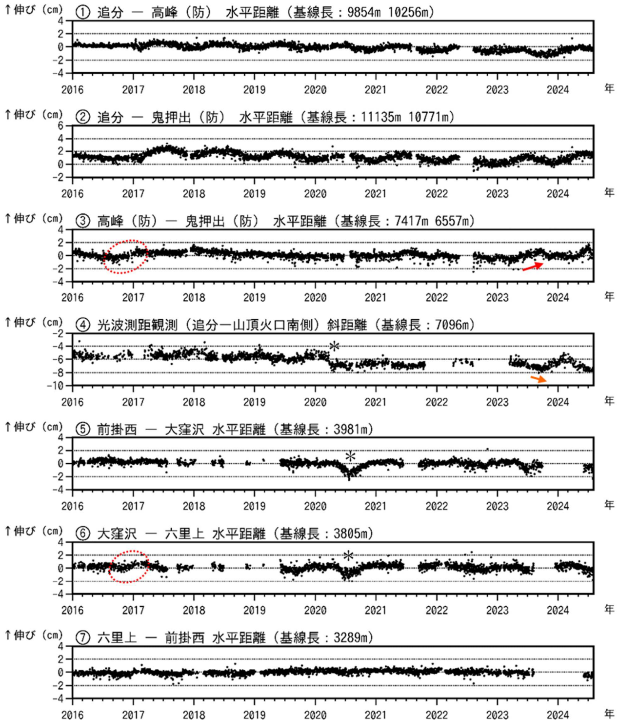
図7-1 浅間山 GNSS 連続観測及び光波測距観測結果(2016年1月1日～2024年7月31日)
