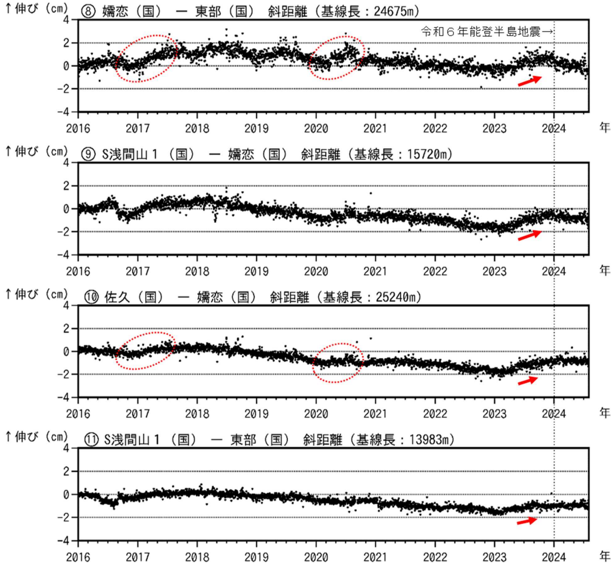
図7-2 浅間山 GNSS 連続観測結果(2016年1月1日~2024年7月31日)
