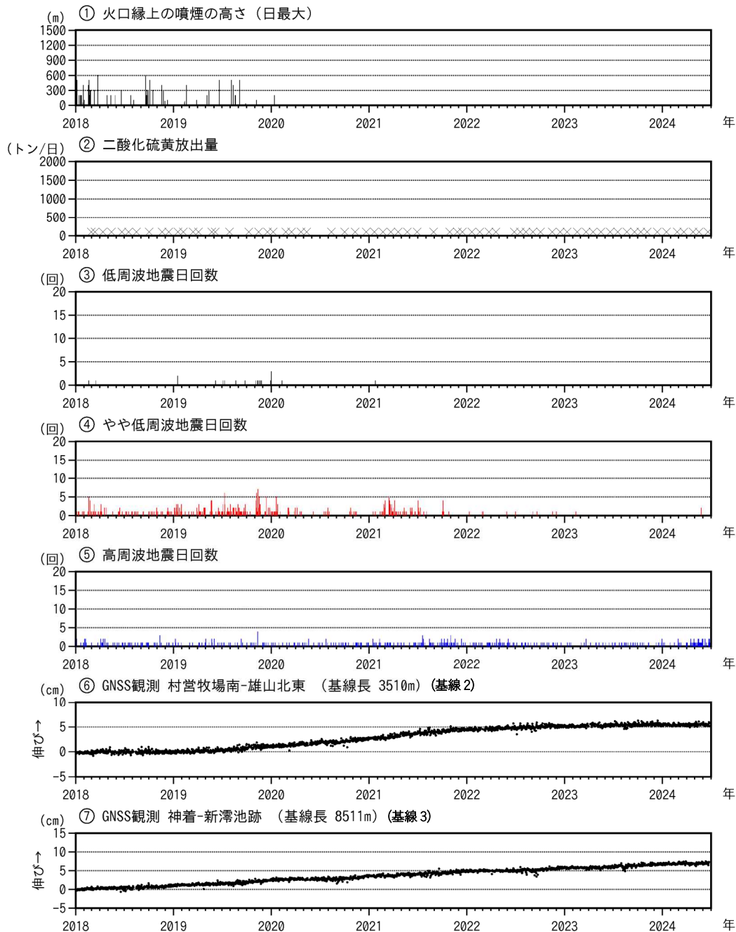
図6 三宅島 火山活動経過図（2018年1月1日～2024年6月30日）
