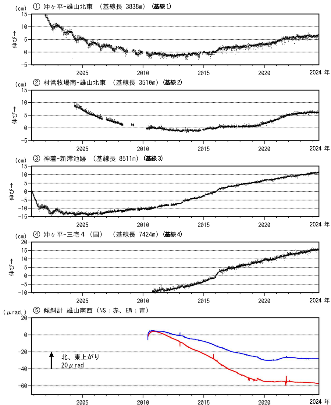
図8 三宅島 GNSS 連続観測及び傾斜計観測結果（2000年10月26日～2024年6月30日）
