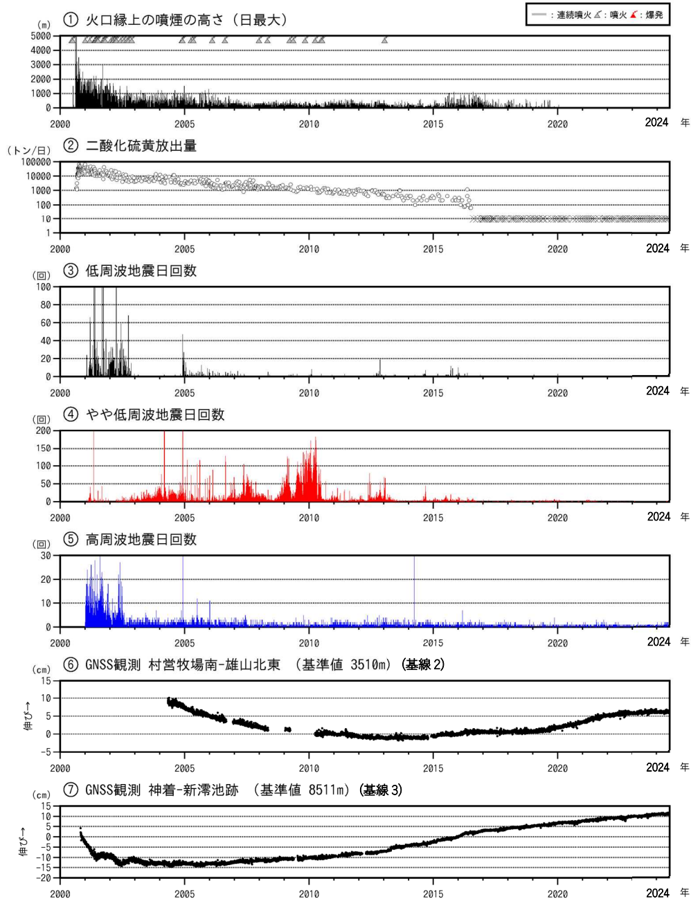
図7 三宅島 長期の火山活動経過図（2000年1月1日～2024年6月30日）
