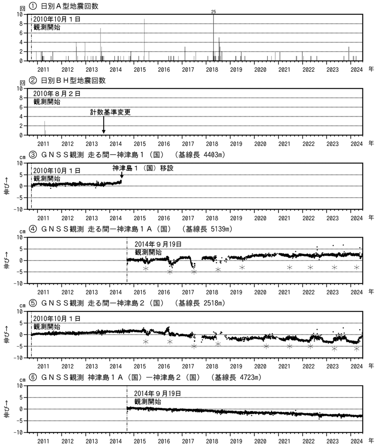
図2 神津島 火山活動経過図(2010年8月2日～2024年6月30日)
