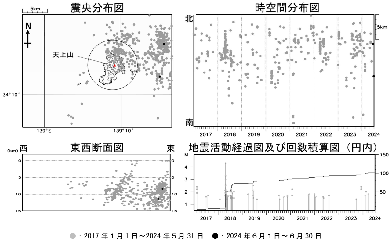
図3 神津島 広域地震観測網による山体・周辺の地震活動（2017年1月1日～2024年6月30日）
