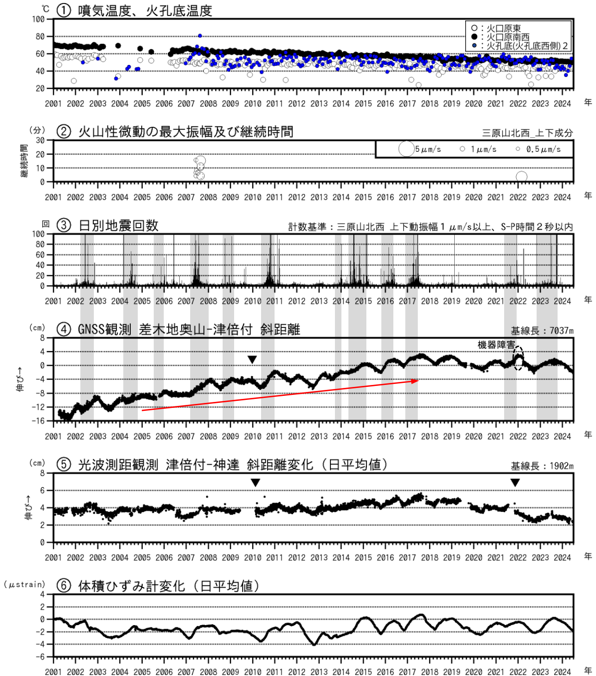
図2 伊豆大島 最近の火山活動経過図（2001年1月～2024年6月30日）
