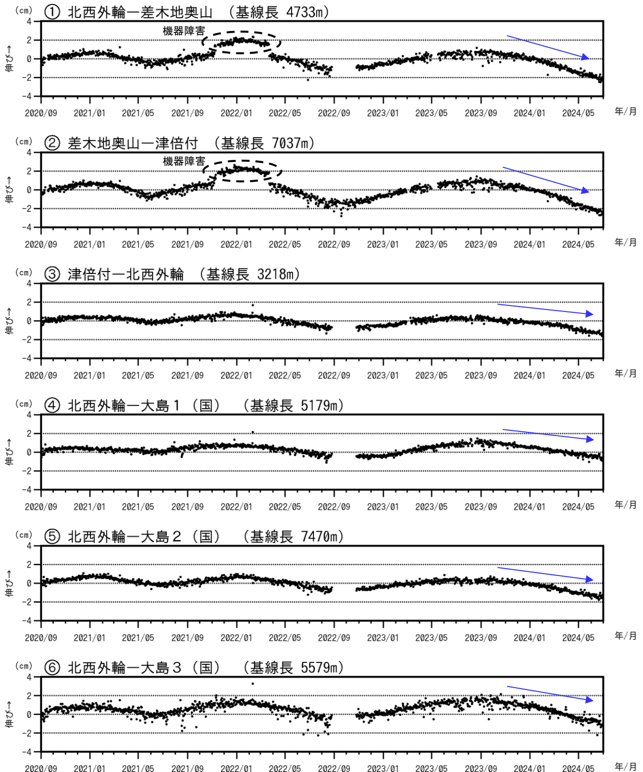
図3-2 伊豆大島 GNSS 連続観測による基線長変化(2020年9月～2024年6月30日)
