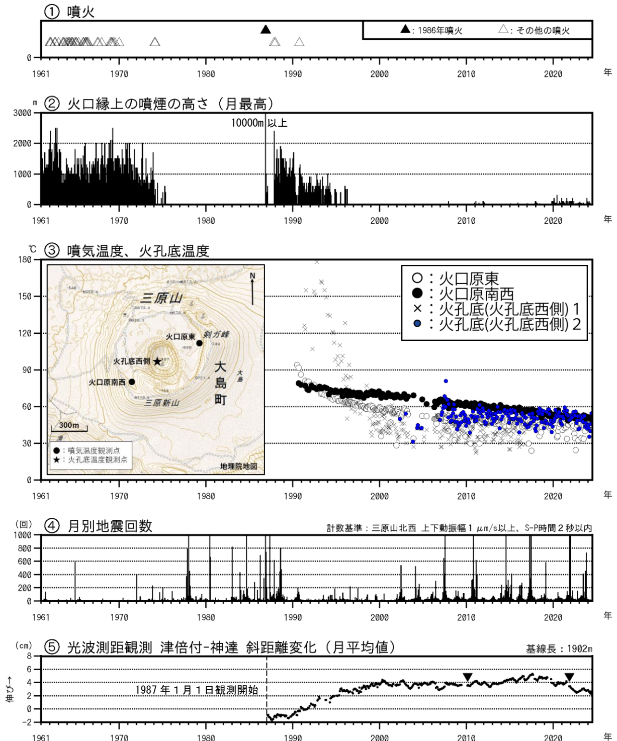
図1 伊豆大島 長期間の火山活動経過図（1961年1月～2024年6月30日）
