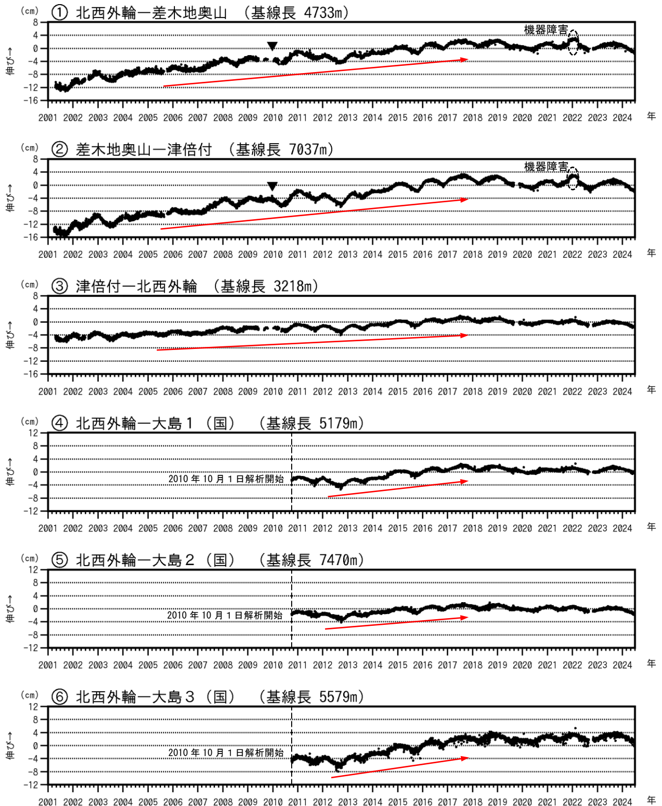
図3-1 伊豆大島 GNSS 連続観測による基線長変化(2001年1月～2024年6月30日)
