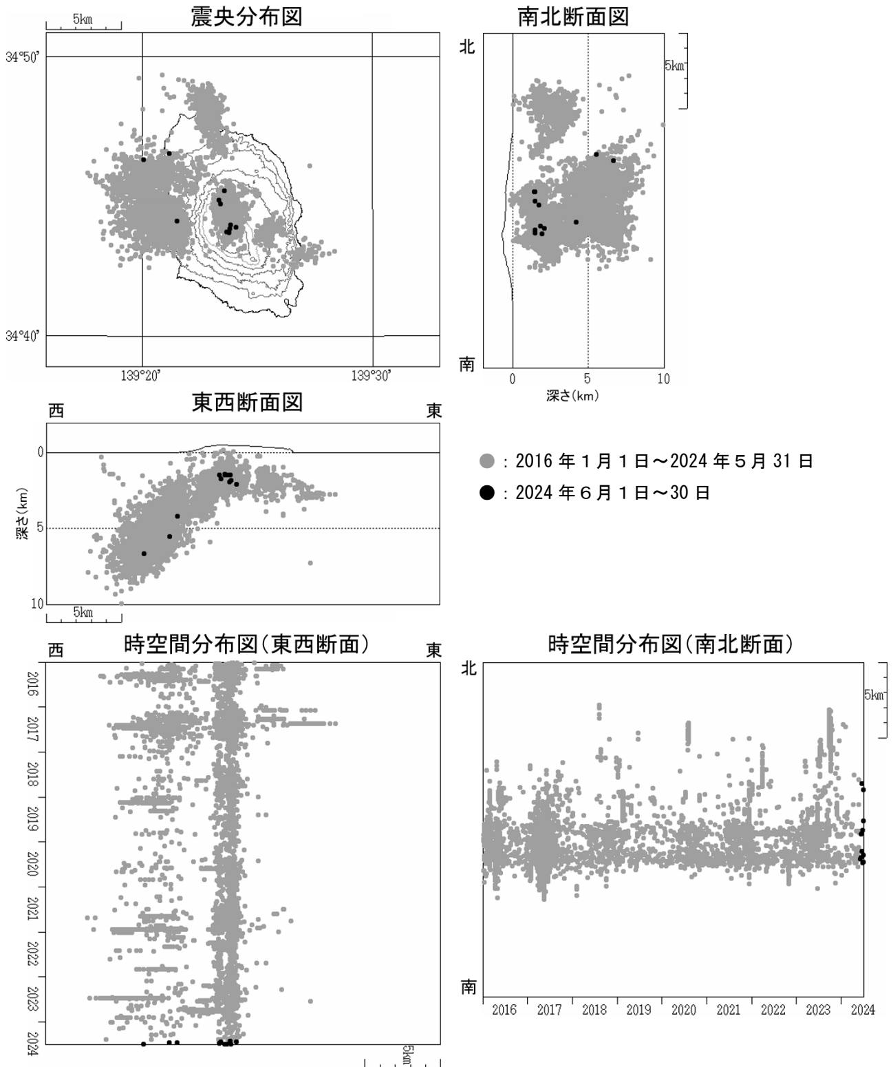
図4 伊豆大島 震源分布図（2016 年 1 月 1 日～2024 年 6 月 30 日）
