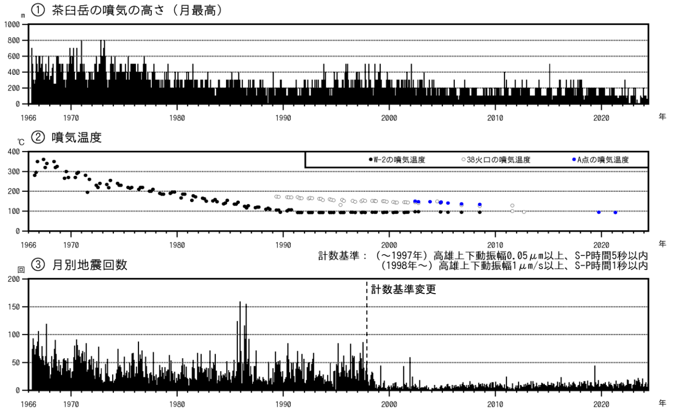
図3-1 那須岳 火山活動経過図（1966年6月～2024年6月）
