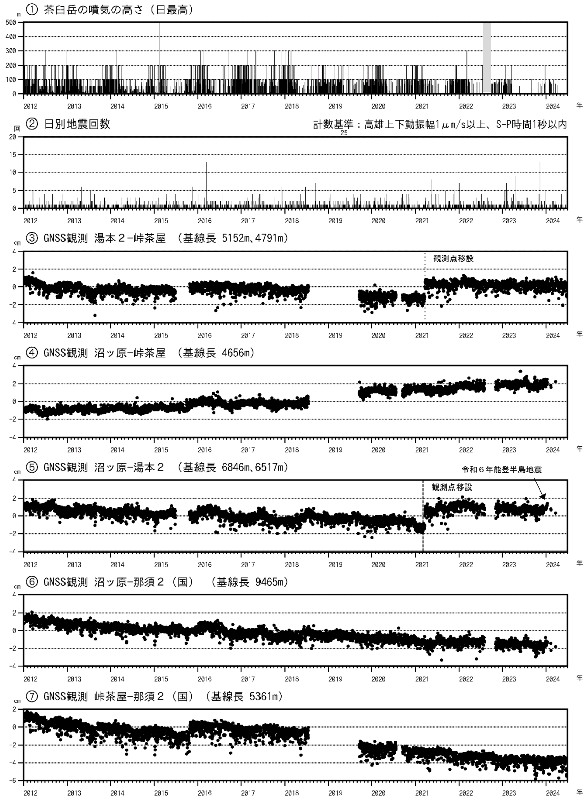
図4 那須岳 火山活動経過図（2012年1月1日～2024年6月30日）
