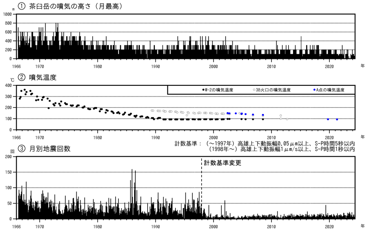
図3-1 那須岳 火山活動経過図（1966年5月～2024年5月）
