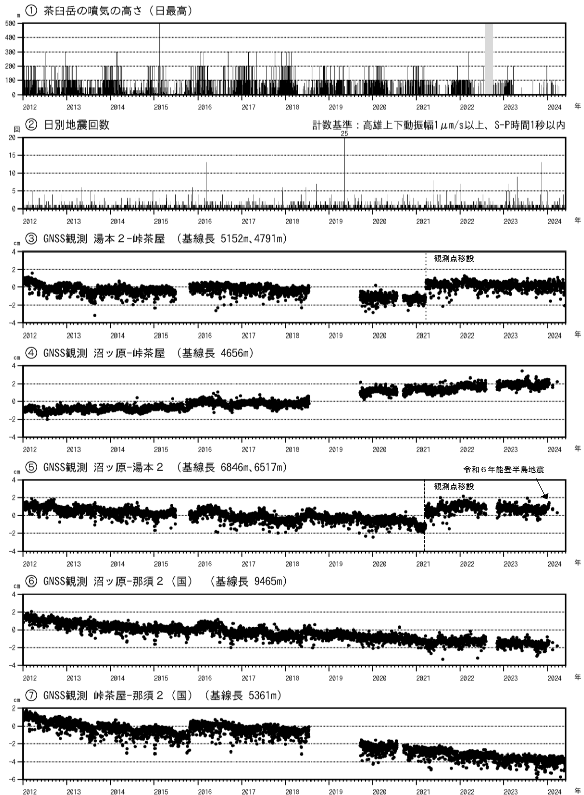
図4 那須岳 火山活動経過図（2012年1月1日～2024年5月31日）
