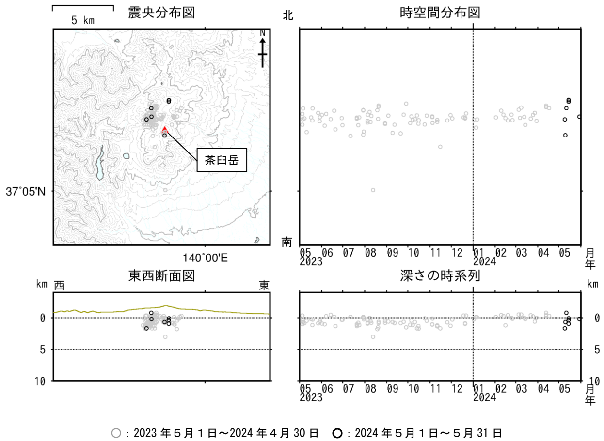
図5 那須岳 震源分布図（2023 年 5 月 1 日～2024 年 5 月 31 日）
