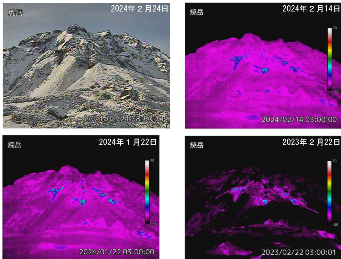
図4 焼岳 中尾峠赤外熱映像カメラによる焼岳の北側斜面の地表面温度分布と可視画像 撮影場所と撮影方向は図11を参照下さい。 ・前月（左下図）及び前年（右下図）と比較して、噴気の状態や地表面温度分布に特段の変化はありません。
