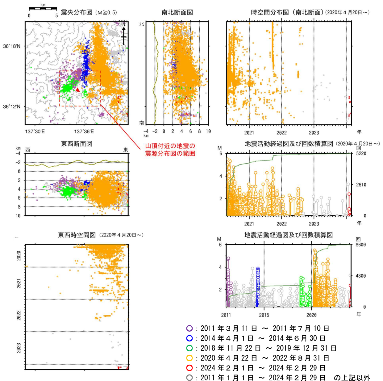
図9 焼岳 広域地震観測網による山体及び周辺の地震活動(2011年1月1日~2024年2月29日)
