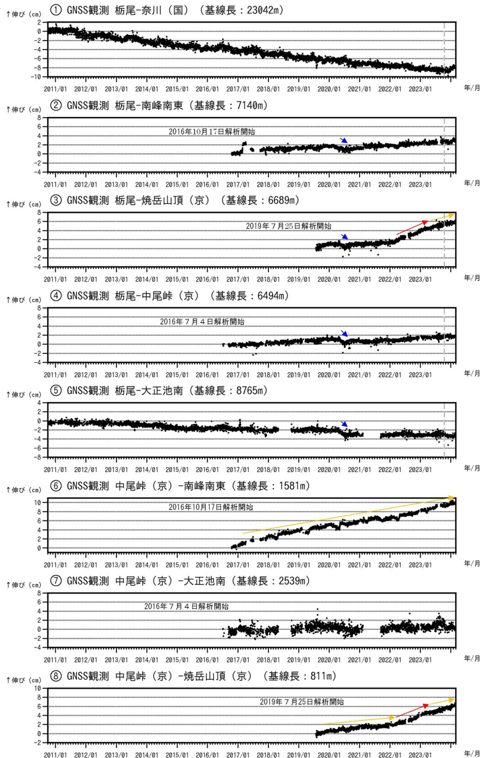
図6 焼岳 GNSS 連続観測による基線長変化（2010年10月1日～2024年2月29日）
