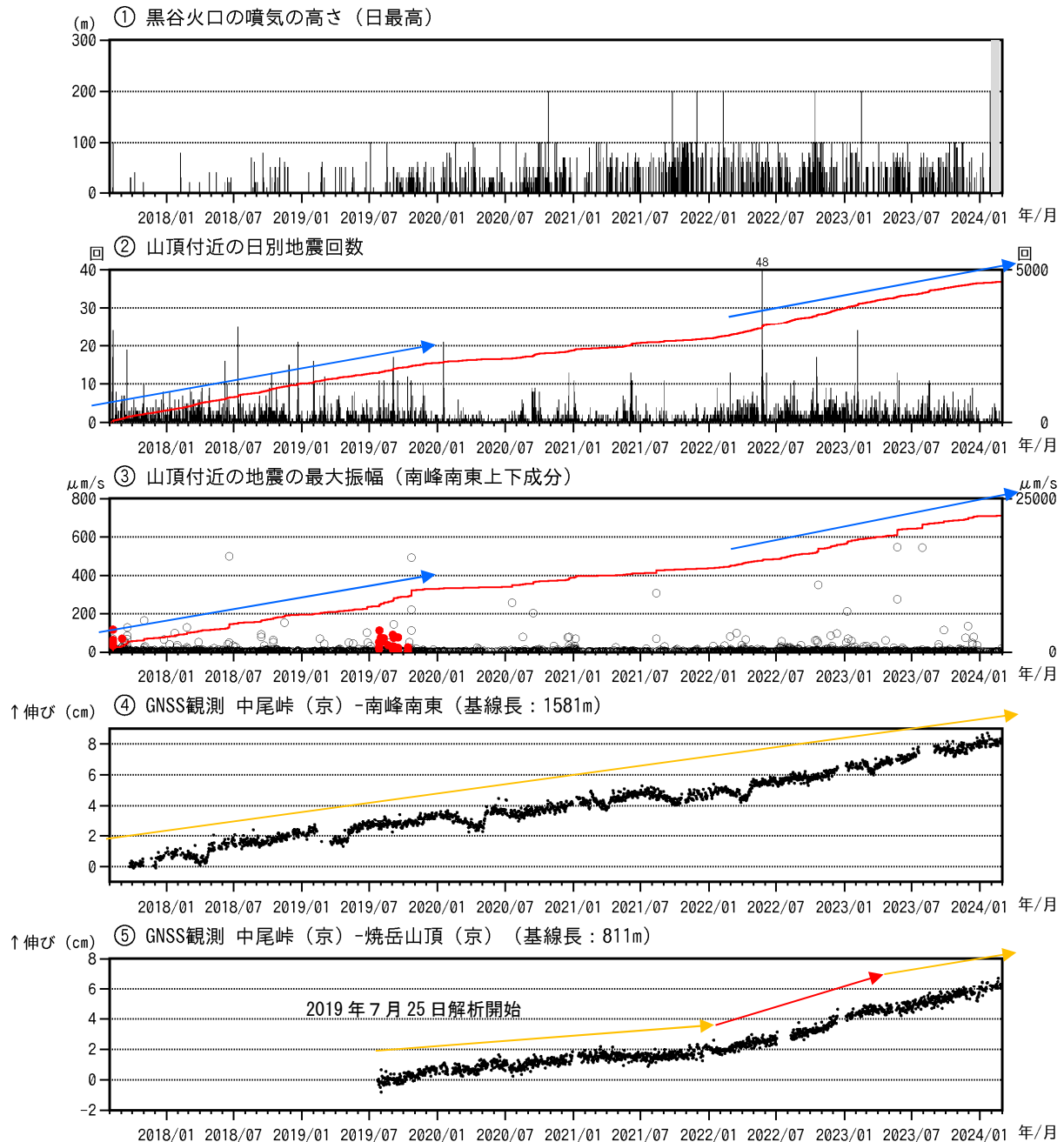
図1 焼岳 火山活動経過図（2017年8月1日～2024年2月29日）
