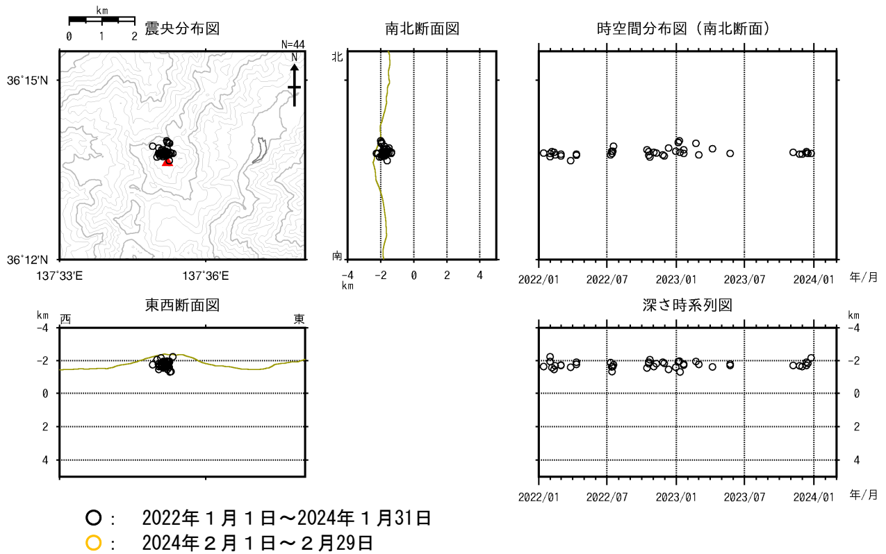
図2 焼岳 山頂付近の地震の震源分布図（2022年1月1日～2024年2月29日）
