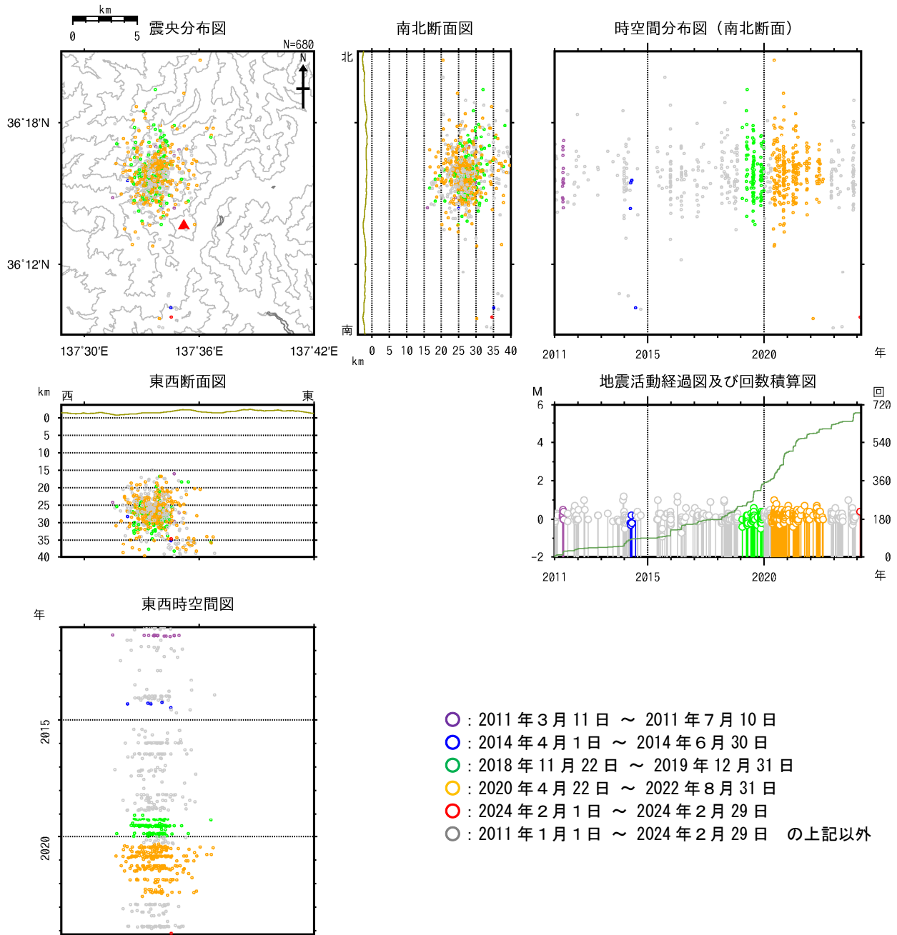
図10 焼岳 広域地震観測網による深部低周波地震の震源分布図（2011年1月1日～2024年2月29日） 広域地震観測網により震源決定したもので、深さは全て海面以下として決定しています。そのため、山頂付近の浅い地震の震源も海面下に決定されています。 M（マグニチュード）は地震の規模を表します。 図中の震源要素は一部暫定値が含まれており、後日変更することがあります。 ・ 焼岳の北西側の深い所を震源とする低周波地震の発生状況に特段の変化はみられません。 ・ 過去には、図9に示したような焼岳周辺の地震活動の活発化がみられた期間付近で、深部低周波地震が増加したことがあります。
