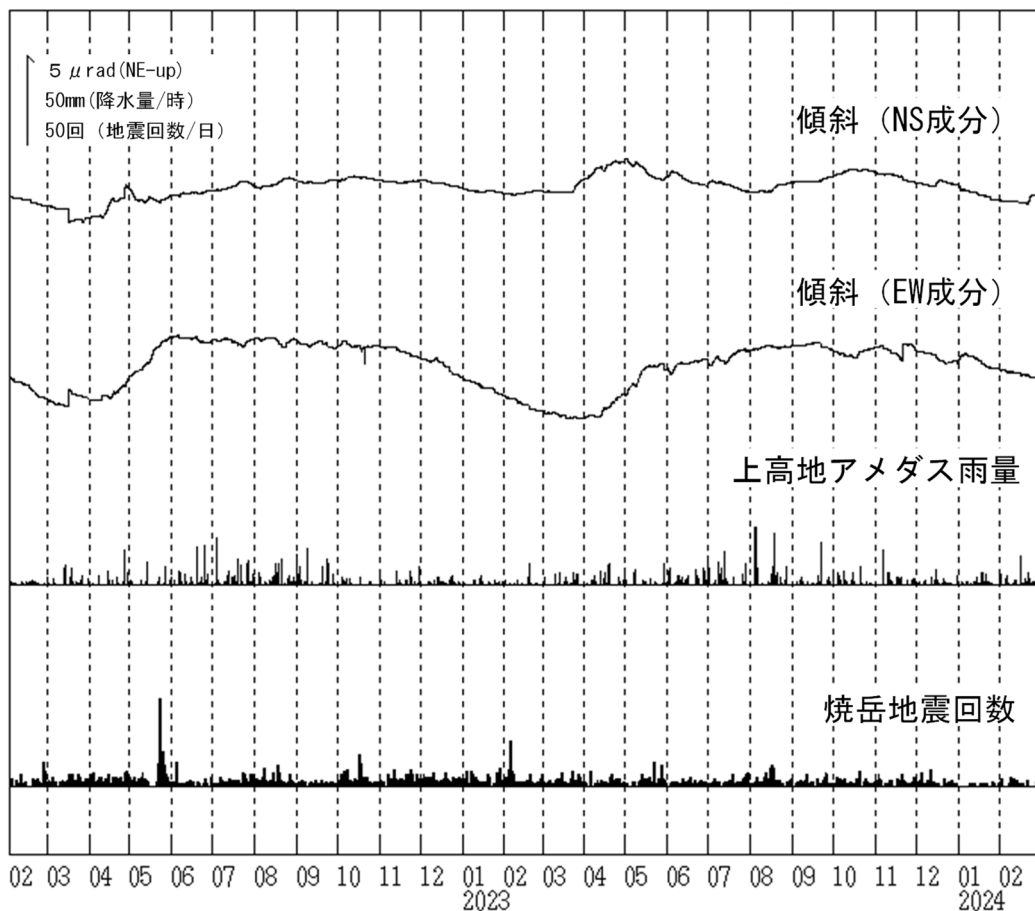
図8 焼岳 南峰南東観測点における傾斜データ（2022年2月1日～2024年2月29日）
