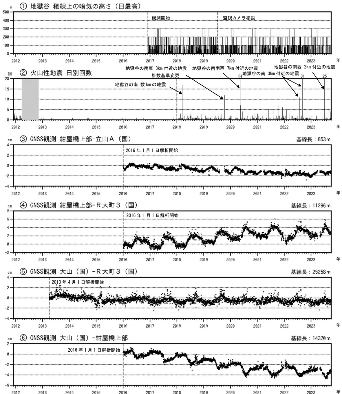
図3 弥陀ヶ原 火山活動経過図（2011年12月1日～2023年9月30日）
