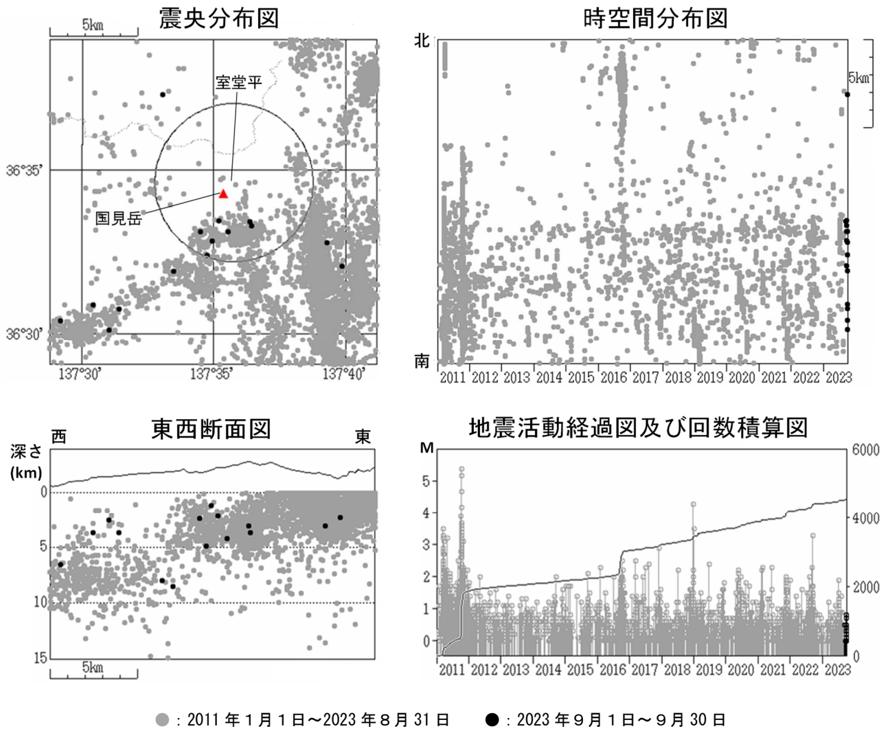
図2 弥陀ヶ原 広域地震観測網による山体・周辺の地震活動（2011 年 1 月 1 日～2023 年 9 月 30 日） 震央分布図中の円は弥陀ヶ原の計数対象地震（室堂平で S-P 時間 1 秒以内）のおよその範囲を示しています。 広域地震観測網により震源決定したもので、深さは全て海面以下として決定しています。 図中の震源要素は一部暫定値が含まれており、後日変更することがあります。 この図では、関係機関の地震波形を一元的に処理し、地震観測点の標高を考慮する等した手法で得られた震源を用いています（ただし、2020 年 8 月以前の地震については火山活動評価のための参考震源です）。
