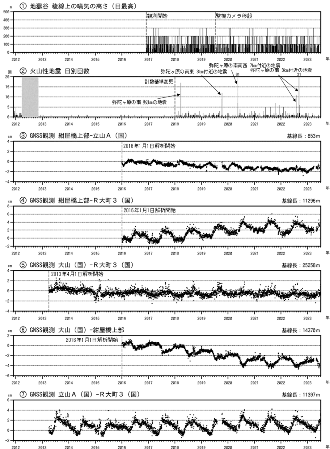
図3 弥陀ヶ原 火山活動経過図（2011年12月1日～2023年6月30日）
