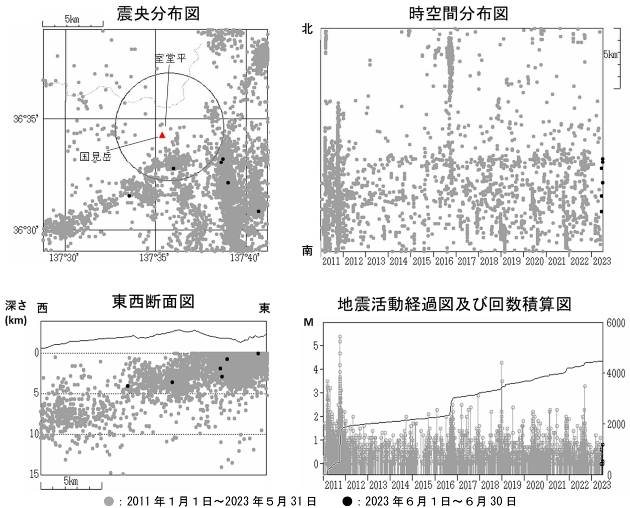
図2 弥陀ヶ原 広域地震観測網による山体・周辺の地震活動（2011 年 1 月 1 日～2023 年 6 月 30 日） 震央分布図中の円は弥陀ヶ原の計数対象地震（室堂平で S-P 時間 1 秒以内）のおよその範囲を示しています。 広域地震観測網により震源決定したもので、深さは全て海面以下として決定しています。 図中の震源要素は一部暫定値が含まれており、後日変更することがあります。 この図では、関係機関の地震波形を一元的に処理し、地震観測点の標高を考慮する等した手法で得られた震源を用いています（ただし、2020 年 8 月以前の地震については火山活動評価のための参考震源です）。
