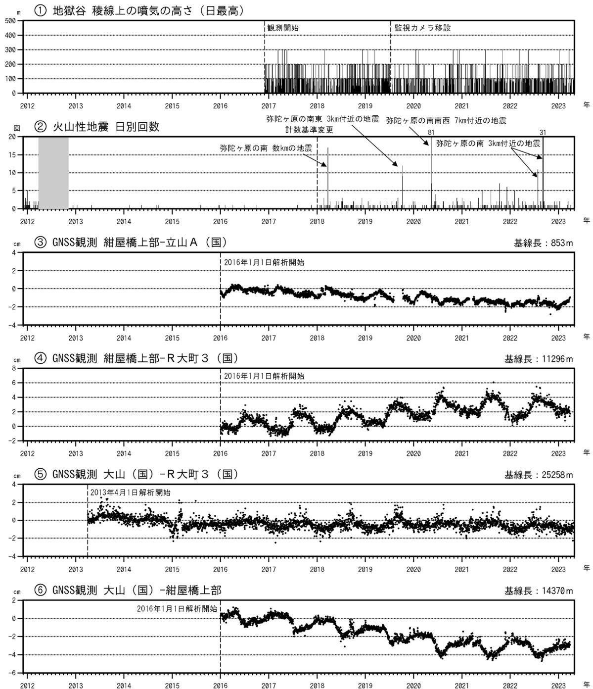
図3 弥陀ヶ原 火山活動経過図（2011年12月1日～2023年4月30日）
