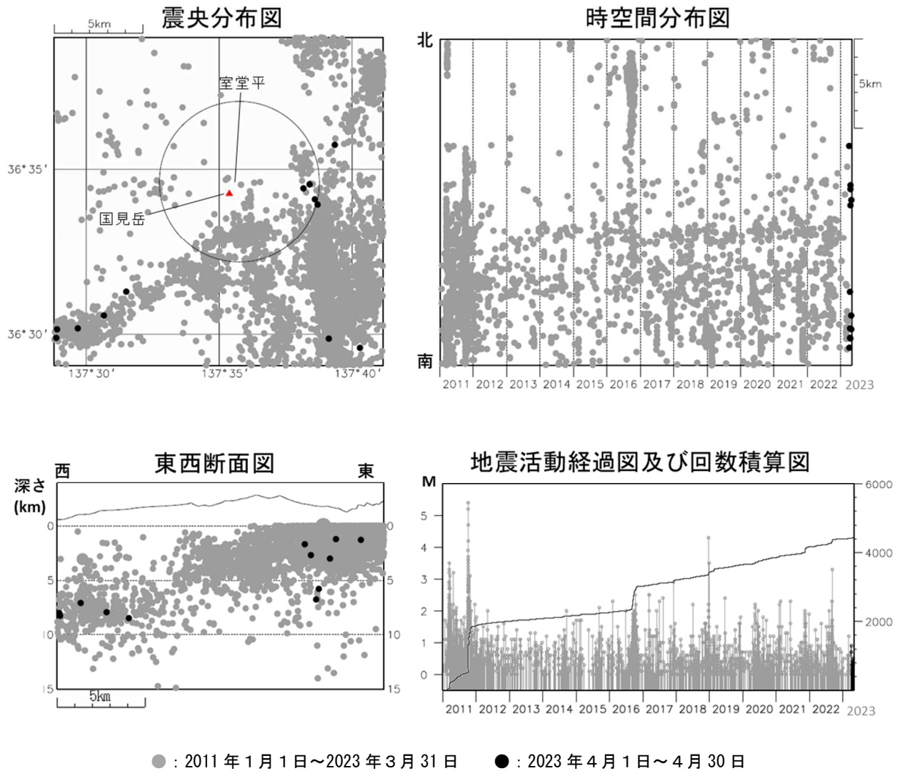
図2 弥陀ヶ原 広域地震観測網による山体・周辺の地震活動（2011 年 1 月 1 日～2023 年 4 月 30 日） 震央分布図中の円は弥陀ヶ原の計数対象地震（室堂平で S-P 時間 1 秒以内）のおよその範囲を示しています。 広域地震観測網により震源決定したもので、深さは全て海面以下として決定しています。 図中の震源要素は一部暫定値が含まれており、後日変更することがあります。 この図では、関係機関の地震波形を一元的に処理し、地震観測点の標高を考慮する等した手法で得られた震源を用いています（ただし、2020 年 8 月以前の地震については火山活動評価のための参考震源です）。
