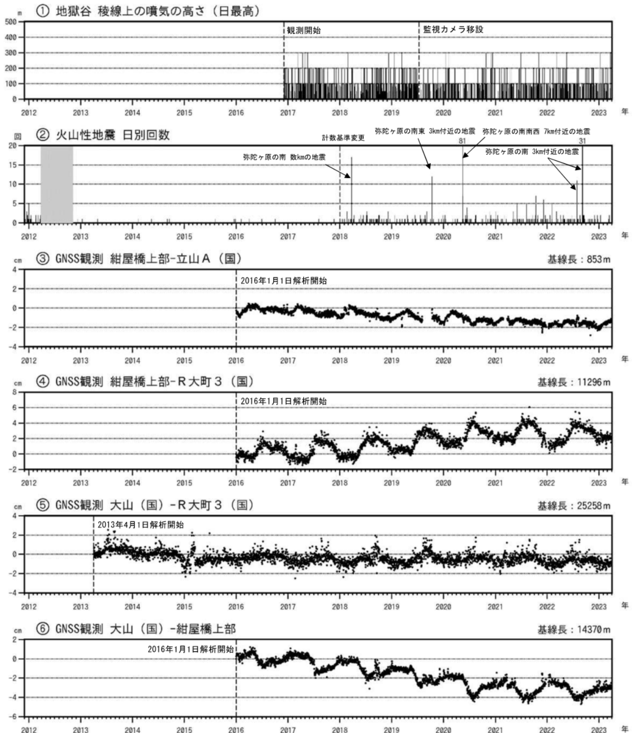
図3 弥陀ヶ原 火山活動経過図（2011年12月1日～2023年3月31日）
