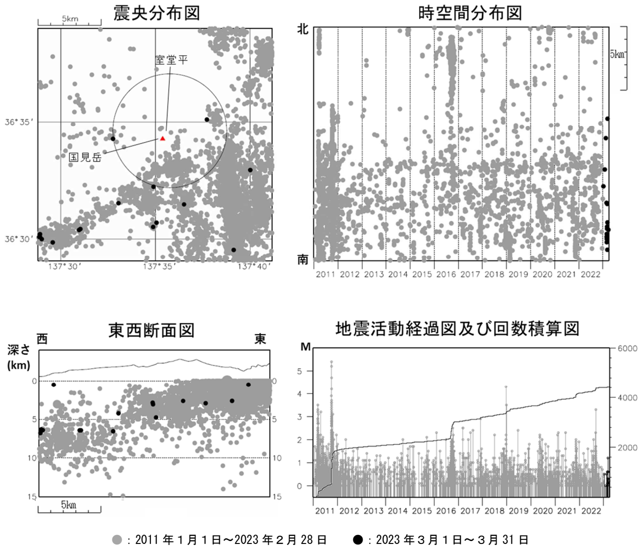
図2 弥陀ヶ原 広域地震観測網による山体・周辺の地震活動（2011 年 1 月 1 日～2023 年 3 月 31 日） 震央分布図中の円は弥陀ヶ原の計数対象地震（室堂平で S-P 時間 1 秒以内）のおよその範囲を示しています。 広域地震観測網により震源決定したもので、深さは全て海面以下として決定しています。 図中の震源要素は一部暫定値が含まれており、後日変更することがあります。 この図では、関係機関の地震波形を一元的に処理し、地震観測点の標高を考慮する等した手法で得られた震源を用いています（ただし、2020 年 8 月以前の地震については火山活動評価のための参考震源です）。
