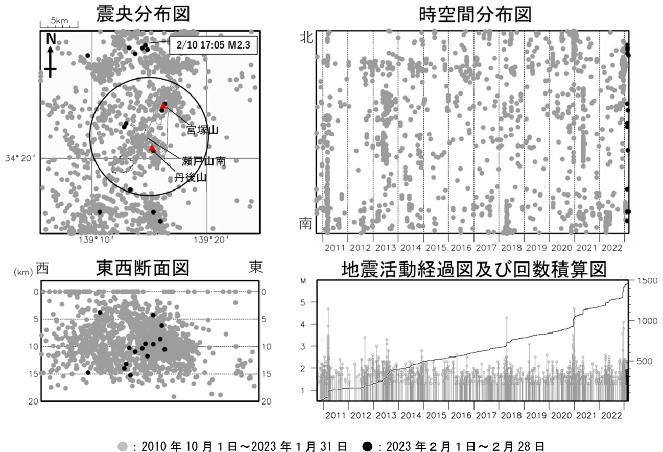
図3 新島 広域地震観測網による山体・周辺の地震活動（2010年10月1日～2023年2月28日）
