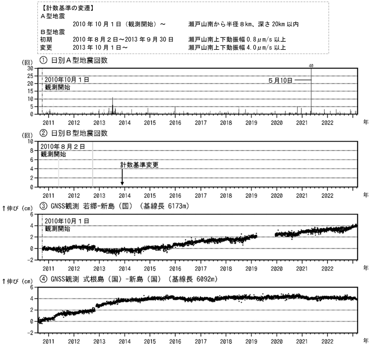
図2 新島 火山活動経過図(2010年8月2日～2023年2月28日)
