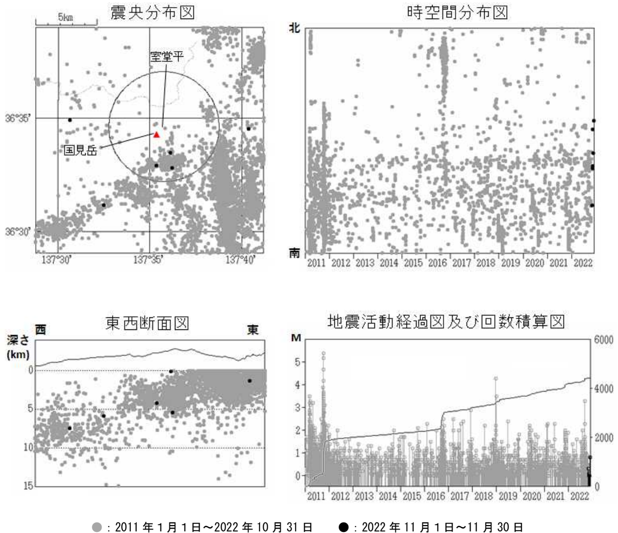
図2 弥陀ヶ原 広域地震観測網による山体・周辺の地震活動（2011年1月1日～2022年11月30日） 震央分布図中の円は弥陀ヶ原の計数対象地震（室堂平でS-P時間1秒以内）のおよその範囲を示しています。 広域地震観測網により震源決定したもので、深さは全て海面以下として決定しています。 図中の震源要素は一部暫定値が含まれており、後日変更することがあります。 この図では、関係機関の地震波形を一元的に処理し、地震観測点の標高を考慮する等した手法で得られた震源を用いています（ただし、2020年8月以前の地震については火山活動評価のための参考震源です）。
