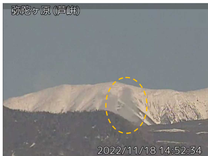
図1 弥陀ヶ原 地獄谷からの噴気の状況（橙丸）（11月18日、芦峠監視カメラによる）
