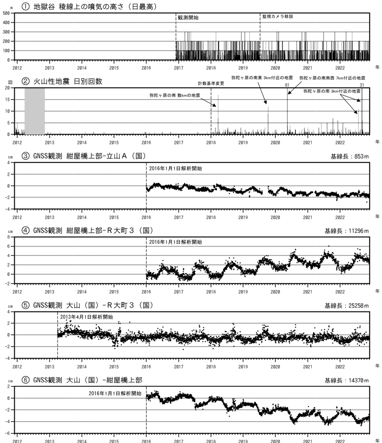
図3 弥陀ヶ原 火山活動経過図（2011年12月1日～2022年11月30日）
