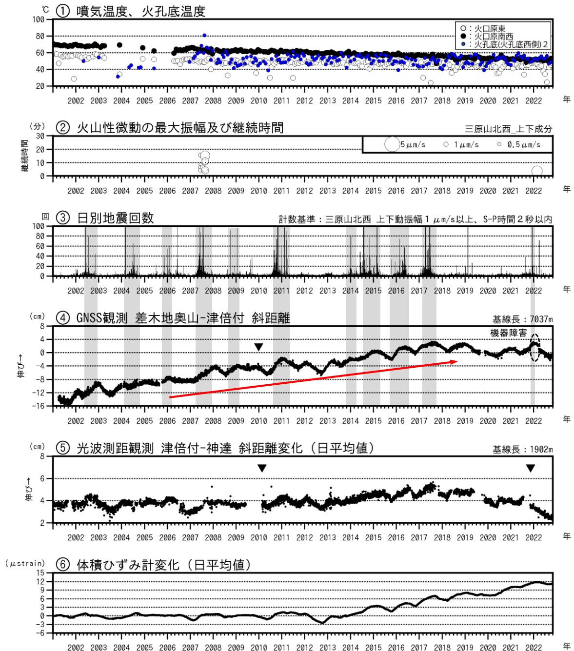
図2 伊豆大島 最近の火山活動経過図（2001年1月～2022年10月31日）
