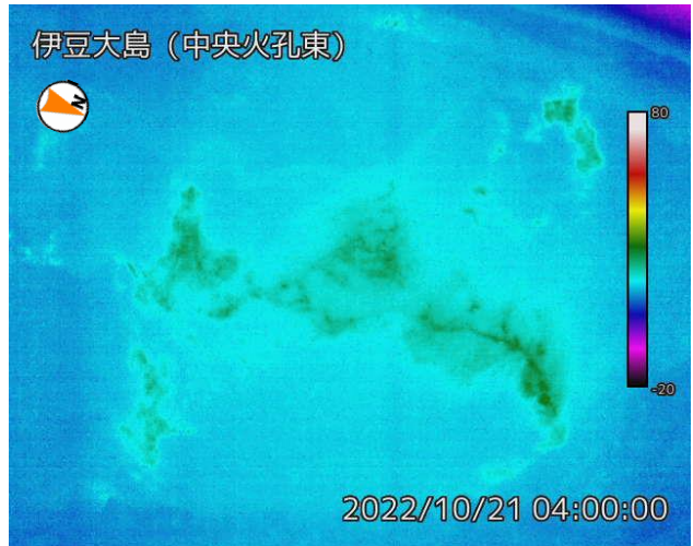
10月21日 中央火孔東監視カメラによる
