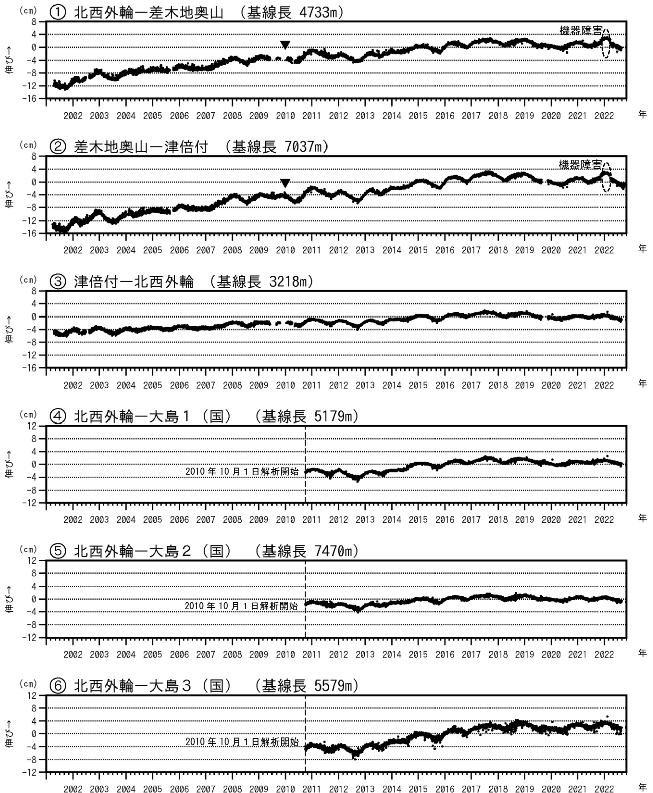
図3-1 伊豆大島 GNSS 連続観測による基線長変化(2001年1月～2022年10月31日)
