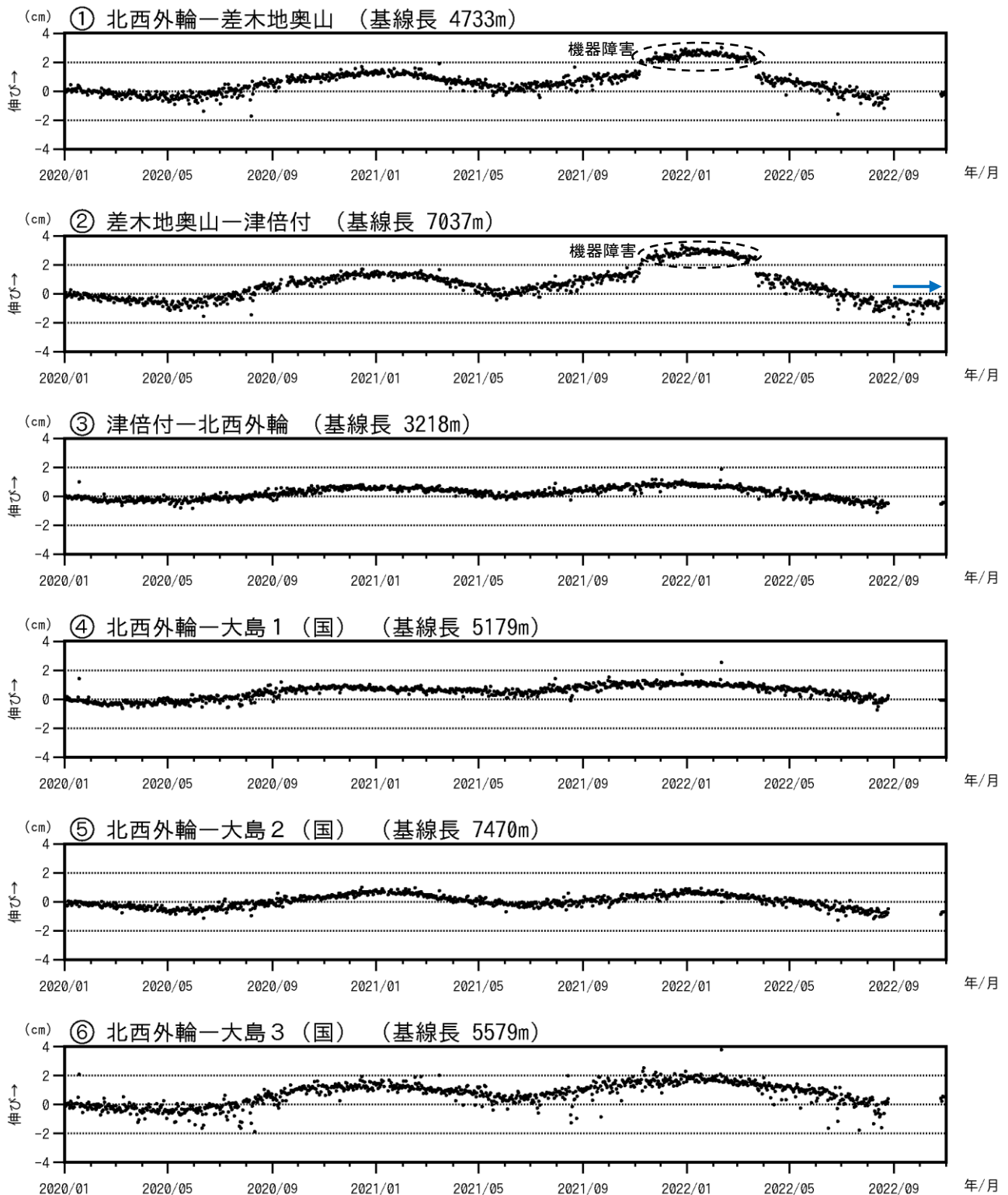
図3-2 伊豆大島 GNSS 連続観測による基線長変化(2020年1月～2022年10月31日)
