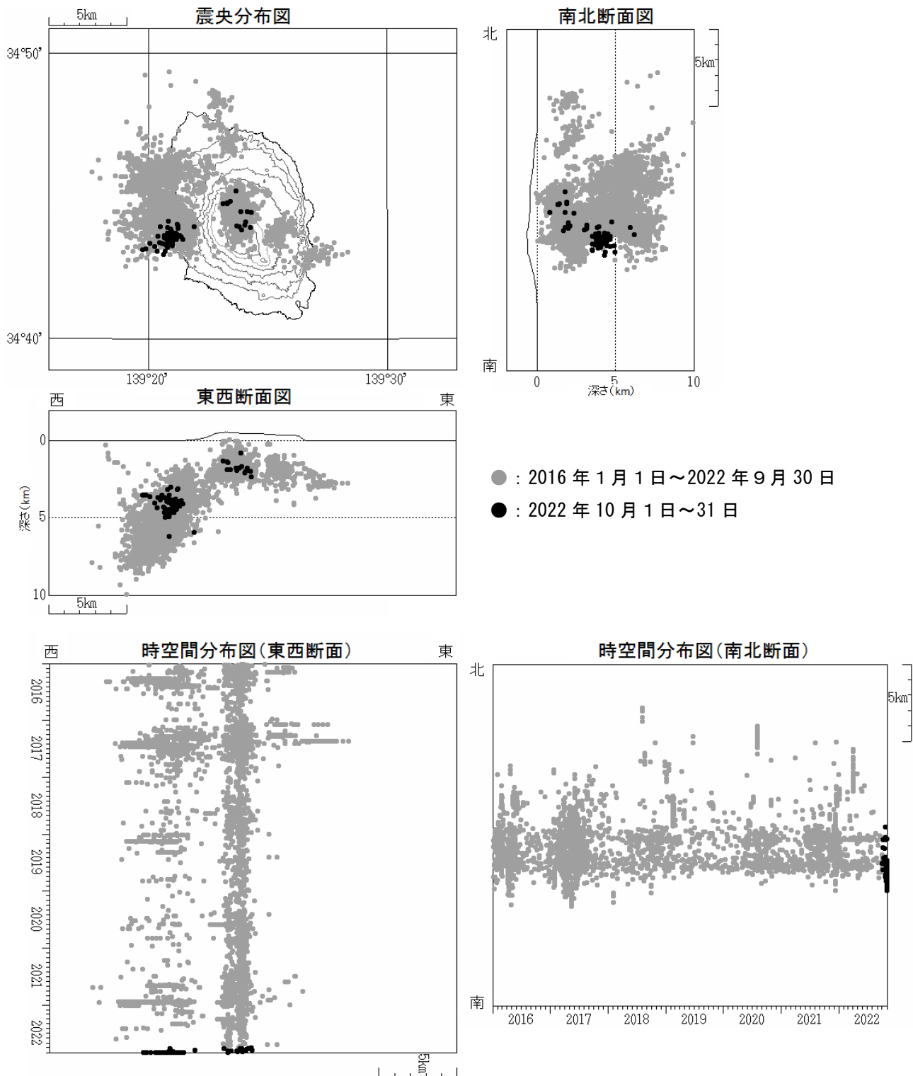
図4 伊豆大島 震源分布図（2016 年 1 月 1 日～2022 年 10 月 31 日）
