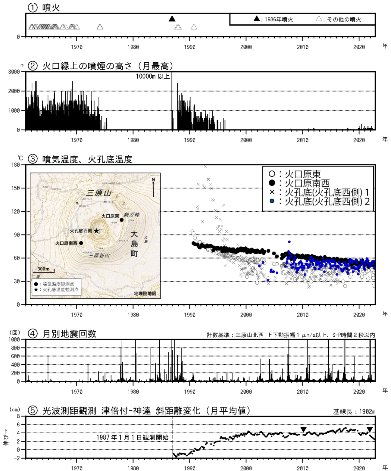
図1 伊豆大島 長期間の火山活動経過図（1961年1月～2022年10月31日）
