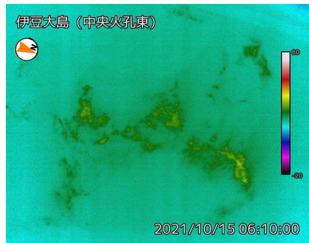
2021年10月15日 中央火孔東監視カメラによる
