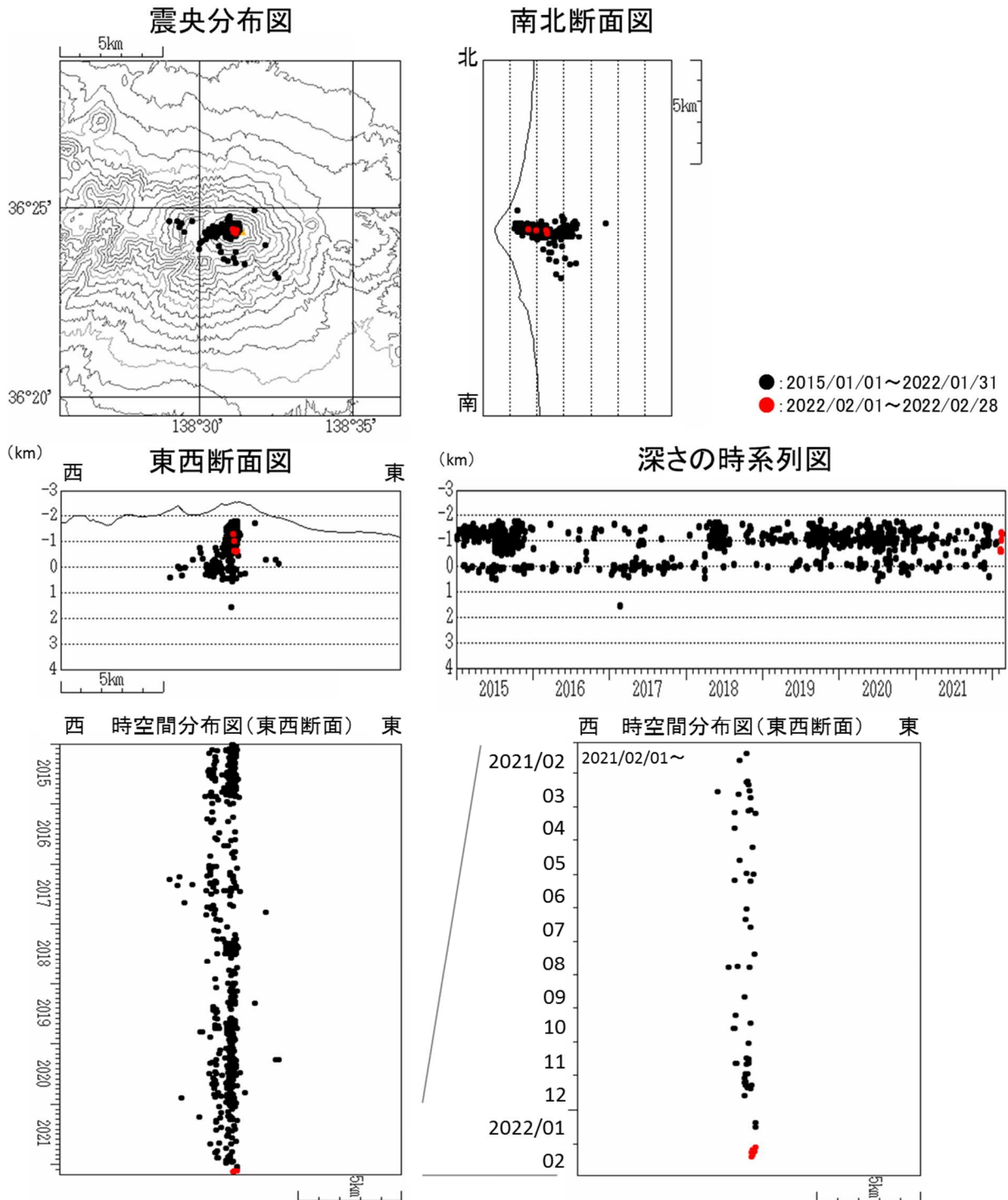
図5 浅間山 震源分布図（2015年1月1日～2022年2月28日） ・火山性地震の震源は、従来からみられている山頂直下の海拔1km付近に分布しています。
