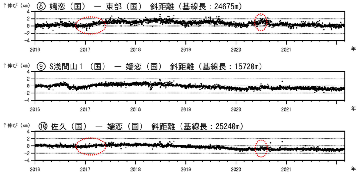
図6-2 浅間山 GNSS 連続観測結果(2016年1月1日～2022年2月28日)
