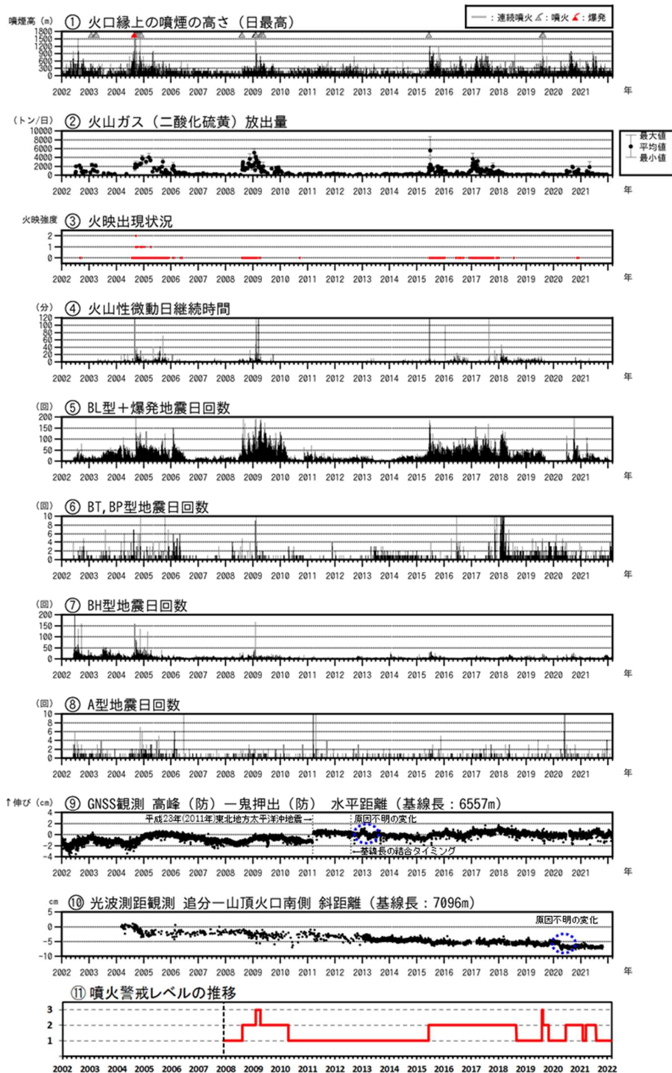
図4 浅間山 火山活動経過図（2002年1月1日～2022年2月28日）
