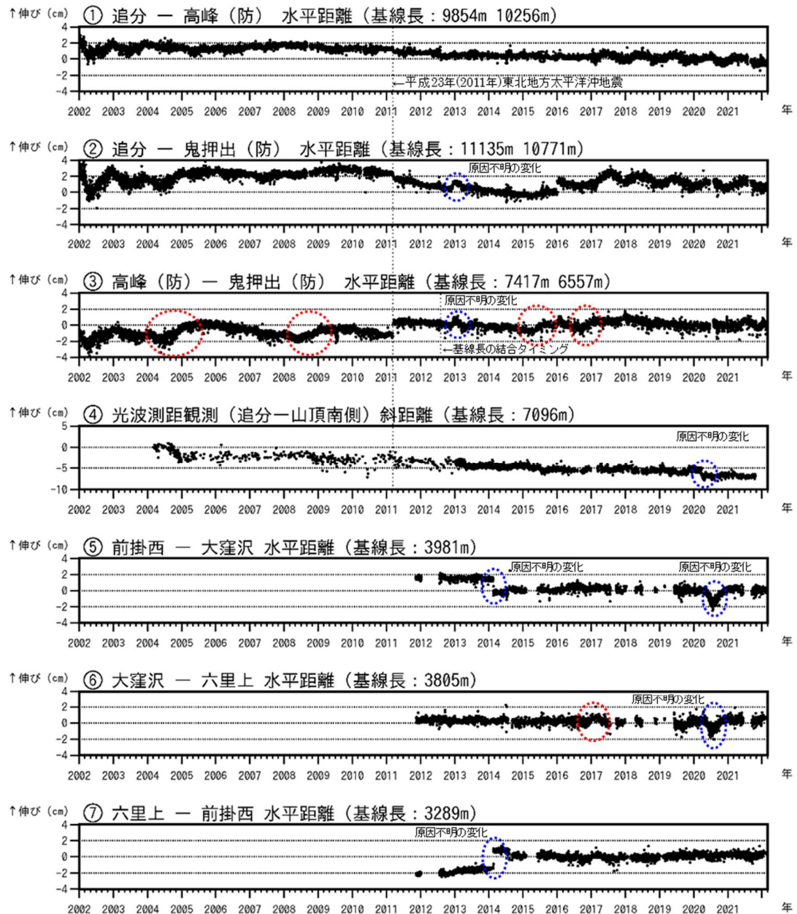
図6-1 浅間山 GNSS連続観測及び光波測距観測の結果(2002年1月1日~2022年2月28日)
