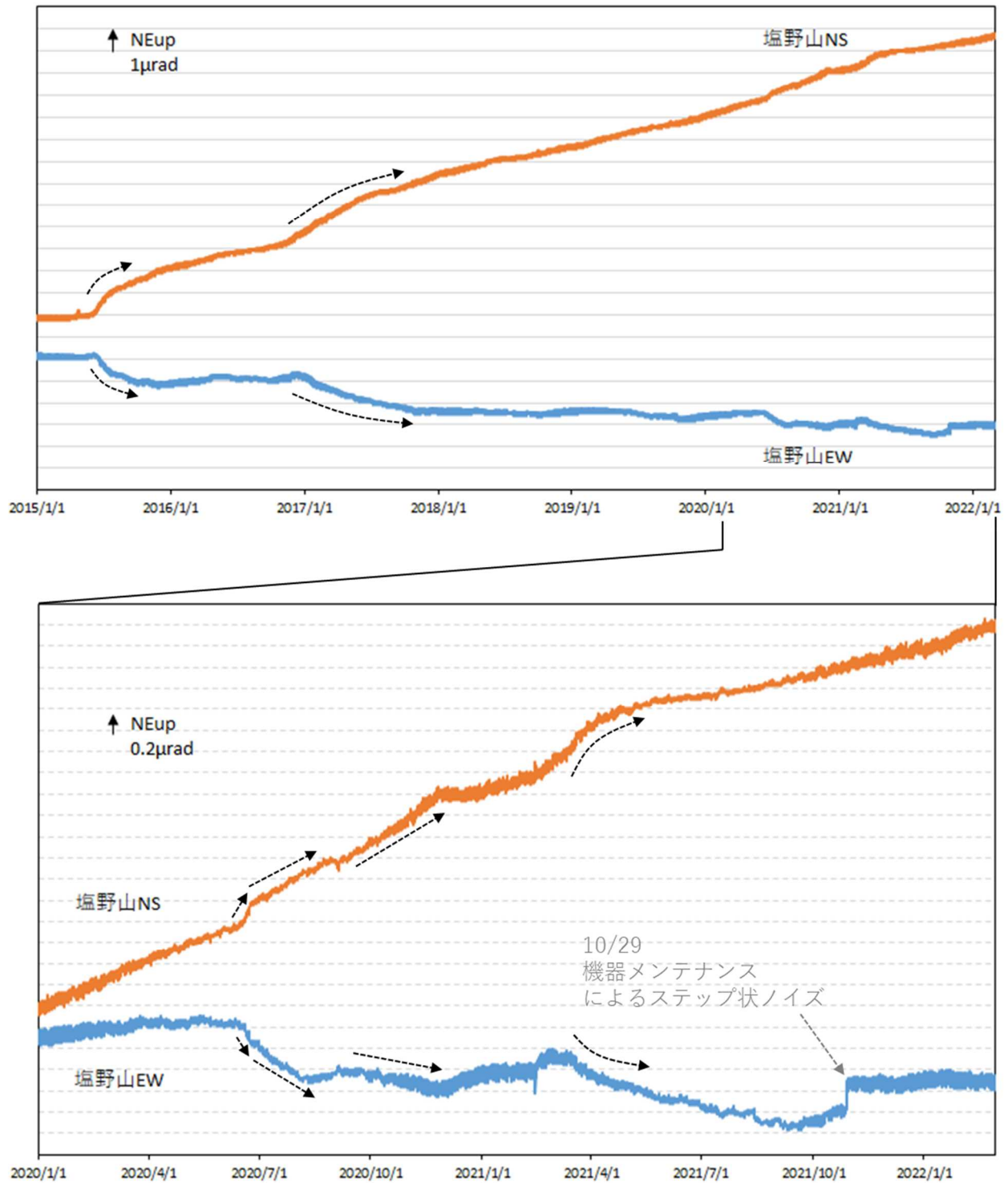
図8 浅間山 塩野山観測点における傾斜データ（2015年1月1日～2022年2月28日）
