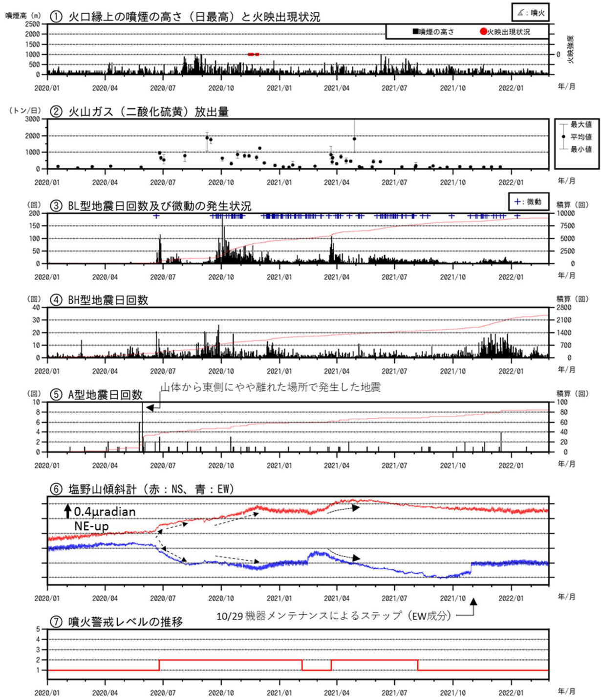
図3 浅間山 火山活動経過図（2020年1月1日～2022年2月28日）
