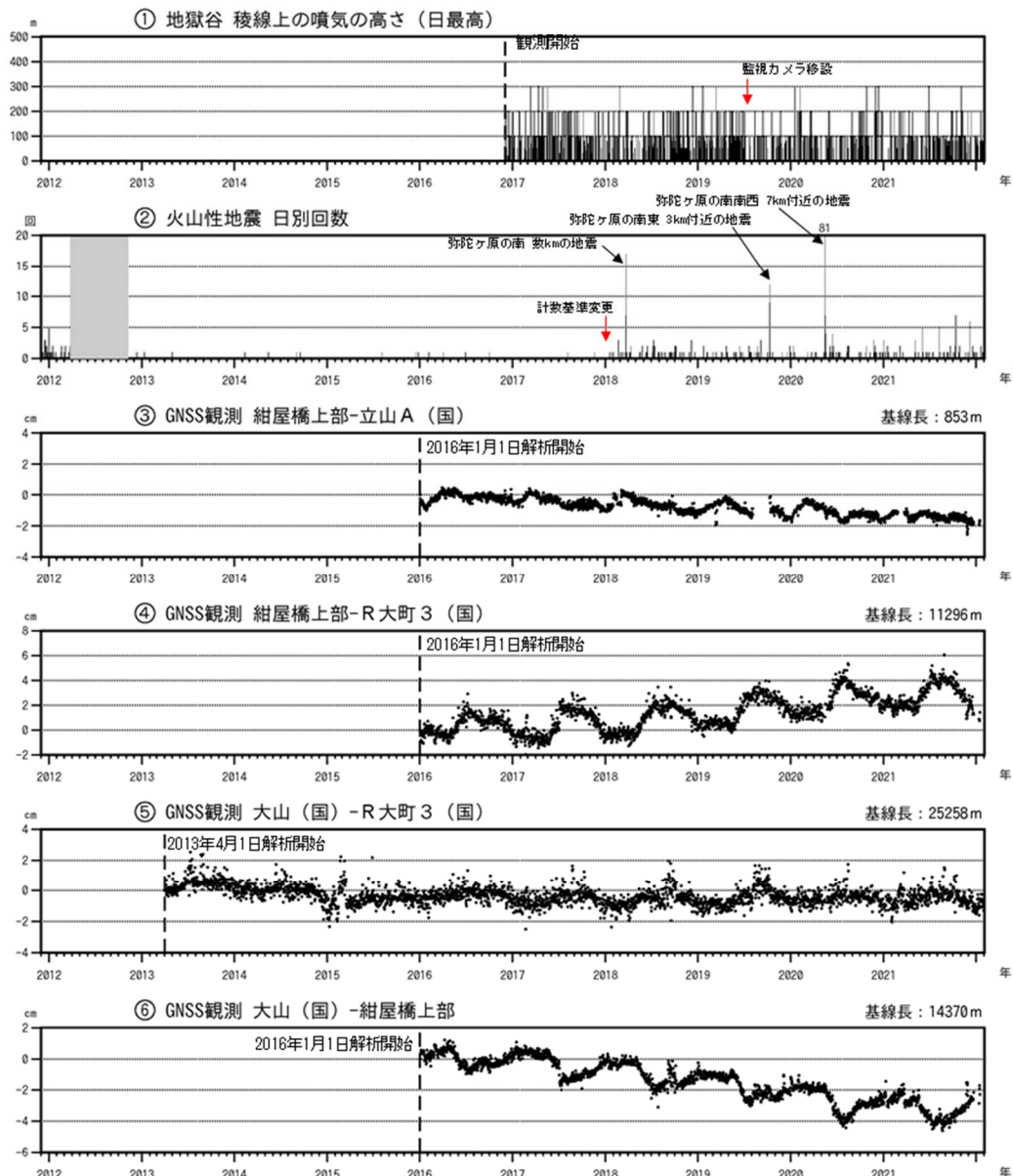
図3 弥陀ヶ原 火山活動経過図（2011年12月1日～2022年1月31日）
