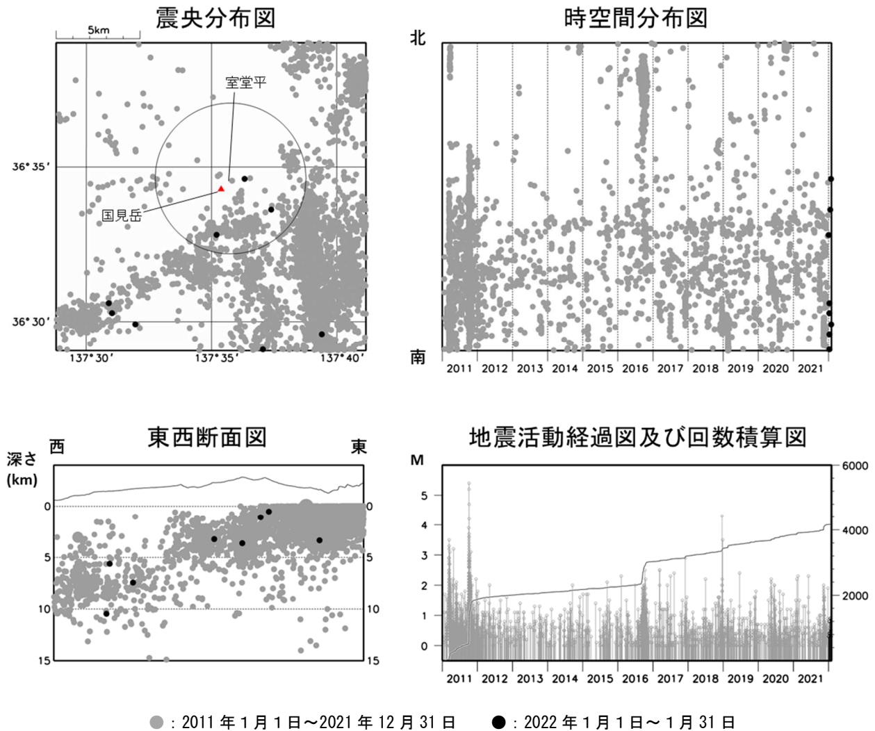
図2 弥陀ヶ原 広域地震観測網による山体・周辺の地震活動（2011 年 1 月 1 日～2022 年 1 月 31 日） 震央分布図中の円は弥陀ヶ原の計数対象地震（室堂平で S-P 時間 1 秒以内）のおよその範囲を示しています。 広域地震観測網により震源決定したもので、深さは全て海面以下として決定しています。 図中の震源要素は一部暫定値が含まれており、後日変更することがあります。 この図では、関係機関の地震波形を一元的に処理し、地震観測点の標高を考慮する等した新手法で得られた震源を用いています（ただし、2020 年 8 月以前の地震については火山活動評価のための参考震源です）。 2022 年 2 月 8 日現在、次の期間の地震について、暫定的に震源精査の基準を変更しているため、その前後の期間と比較して微小な地震での震源決定数の変化（増減）が見られます。 (1) 2020 年 9 月 1 日から 10 月 23 日まで、(2) 2021 年 1 月 9 日から 3 月 7 日まで、 (3) 2021 年 4 月 19 日から 12 月 5 日まで
