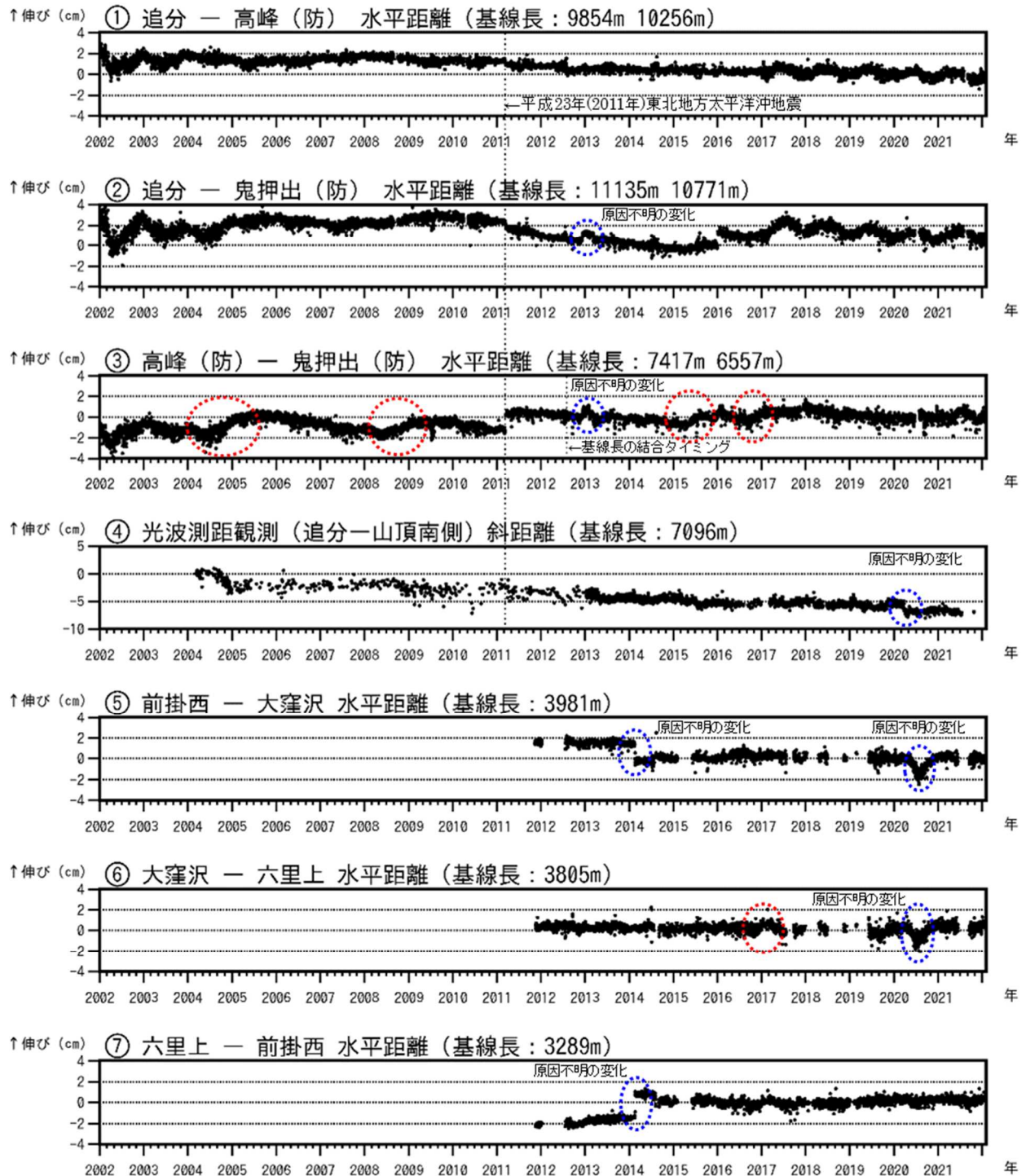
図6-1 浅間山 GNSS連続観測及び光波測距観測の結果(2002年1月1日~2022年1月31日) 2010年10月及び2016年1月に解析方法を変更しています。
