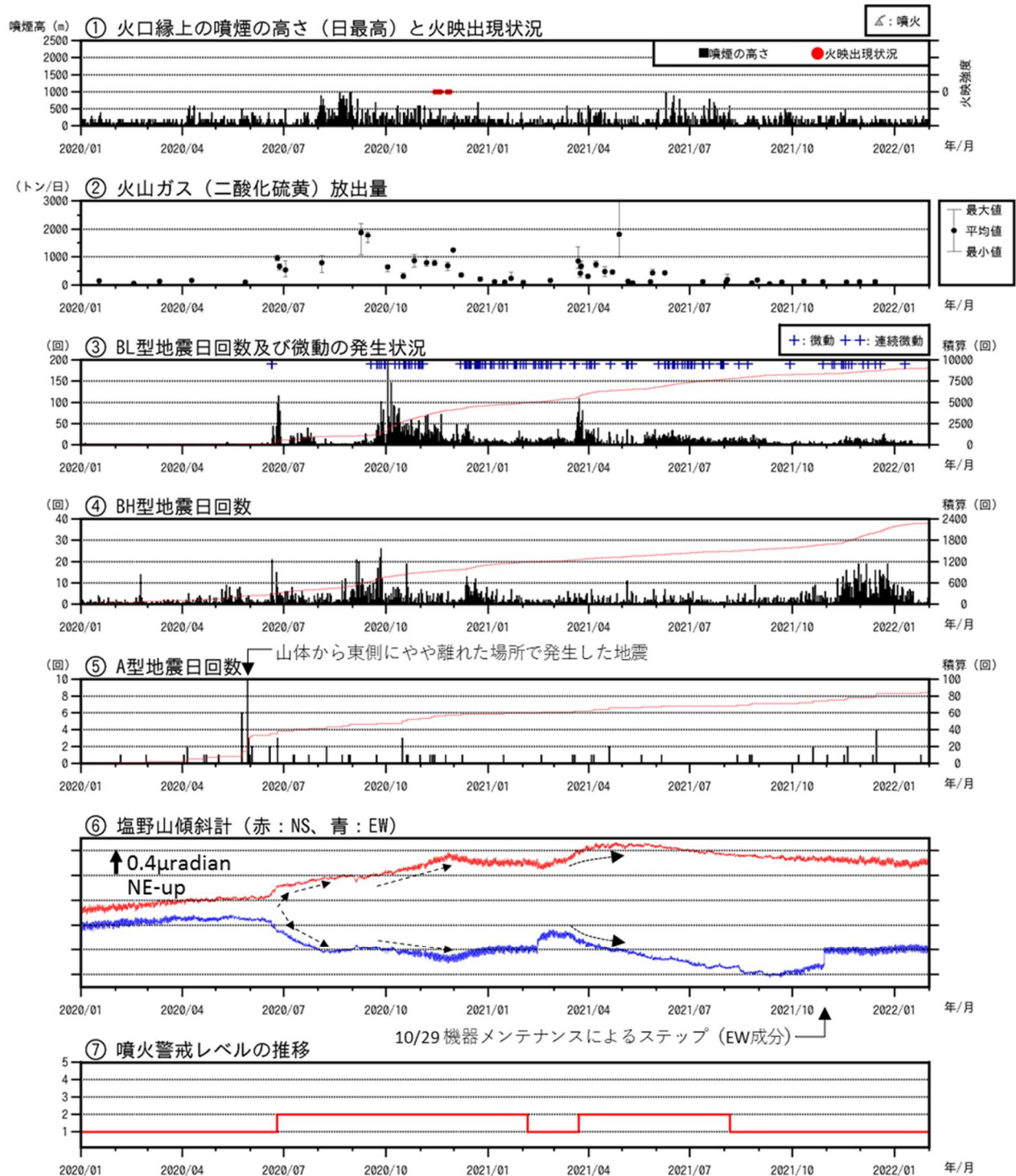
図3 浅間山 火山活動経過図（2020年1月1日～2022年1月31日）
