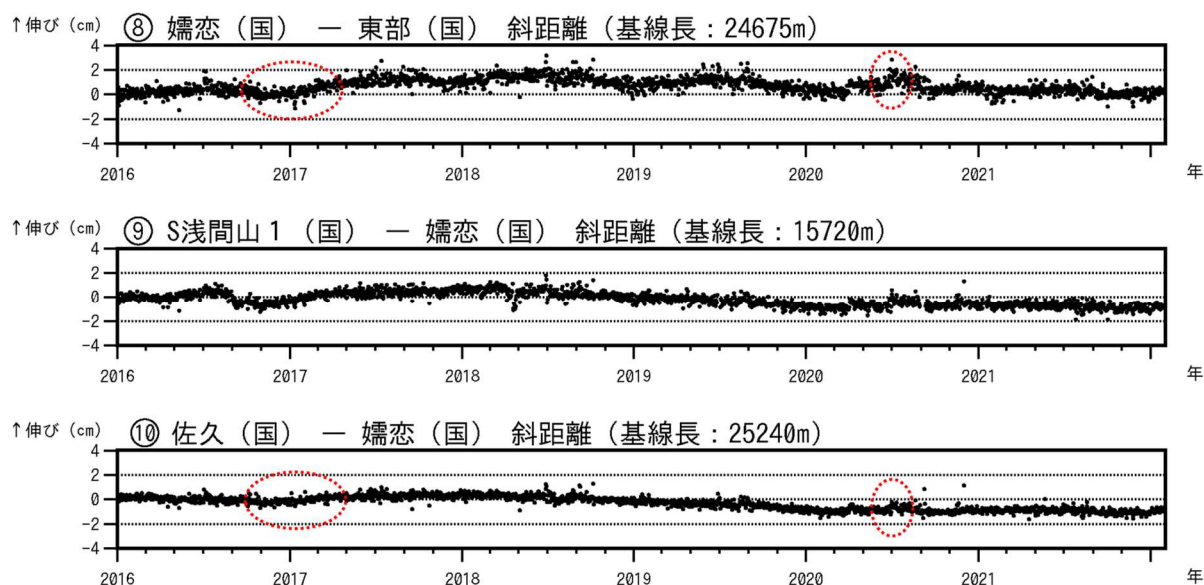
図6-2 浅間山 GNSS連続観測結果(2016年1月1日~2022年1月31日)
