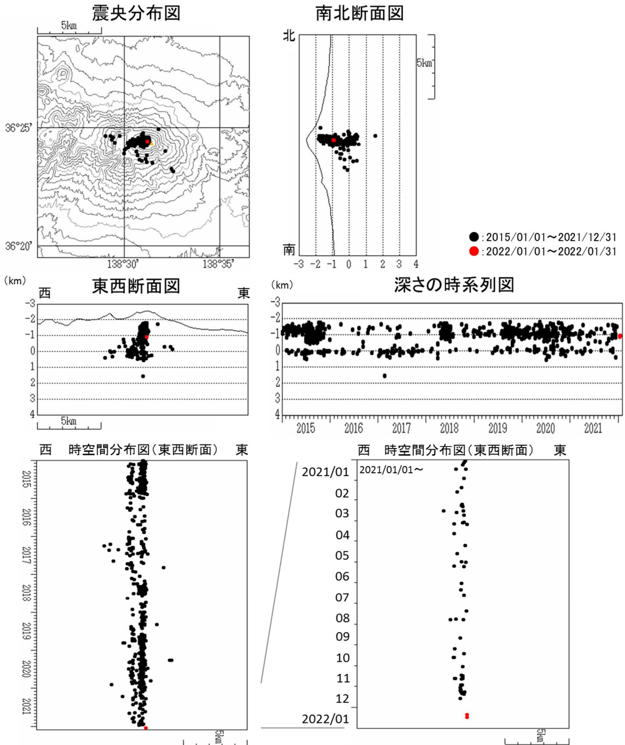
図5 浅間山 震源分布図（2015年1月1日～2022年1月31日） ・火山性地震の震源は、従来からみられている山頂直下の海拔1km付近に分布しています。
