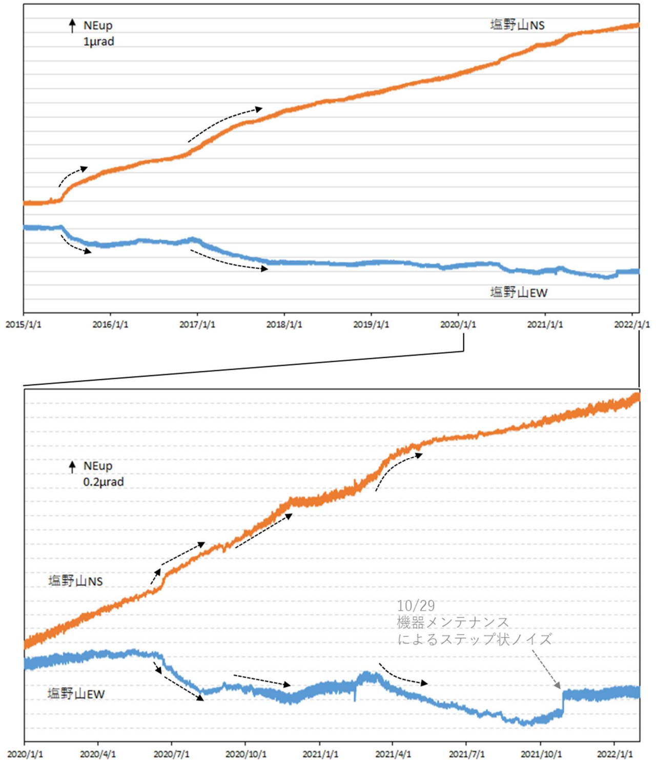
図8 浅間山 塩野山観測点における傾斜データ（2015年1月1日～2022年1月31日）
