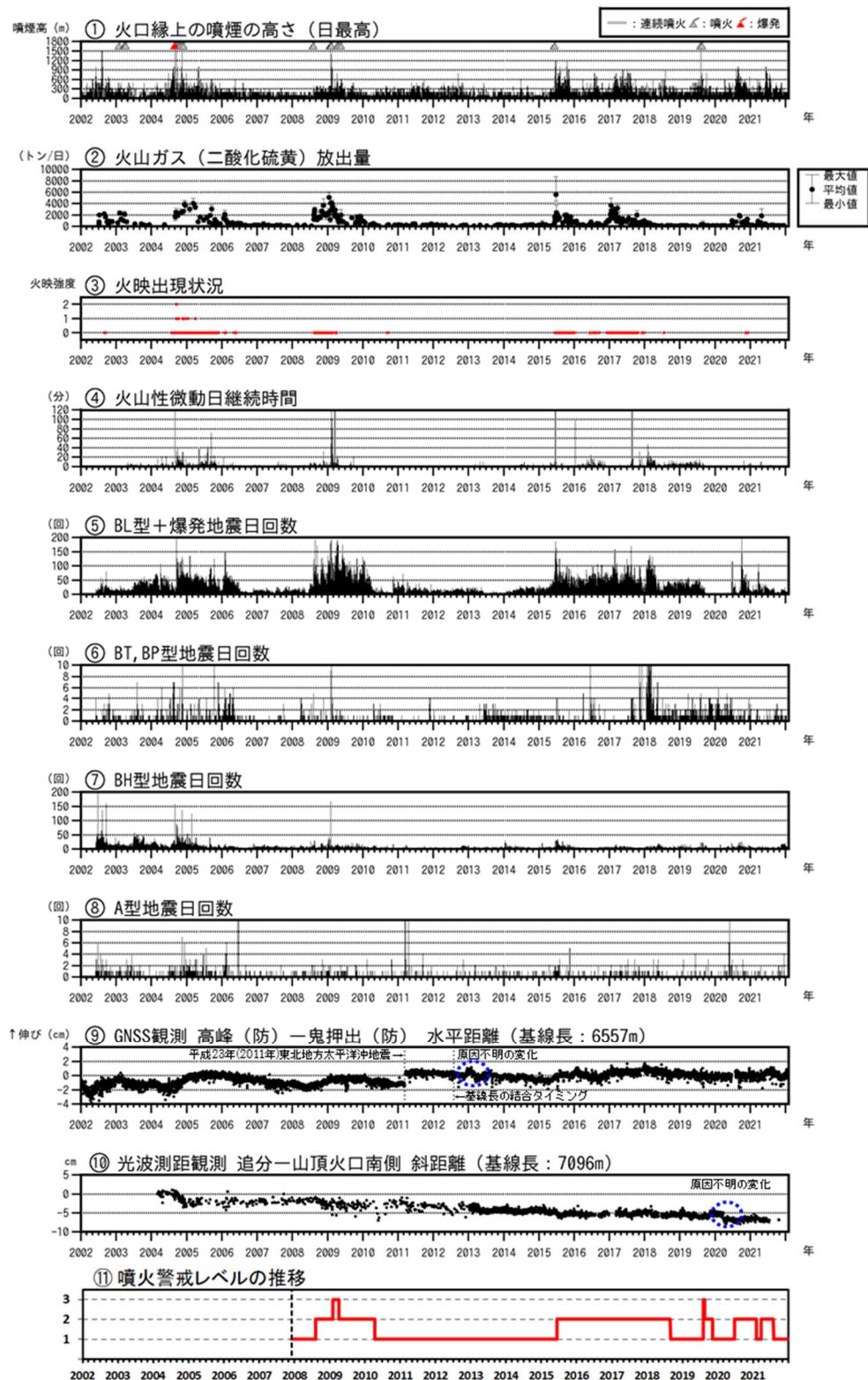
図4 浅間山 火山活動経過図（2002年1月1日～2022年1月31日）
