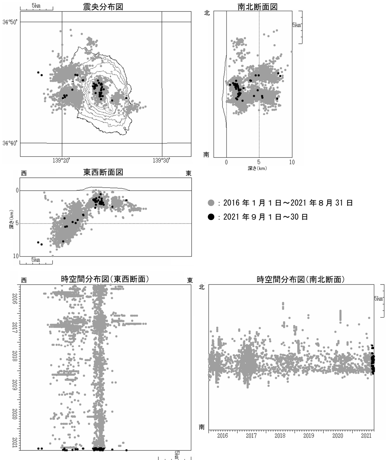
図4 伊豆大島 震源分布図（2016 年 1 月 1 日～2021 年 9 月 30 日）
