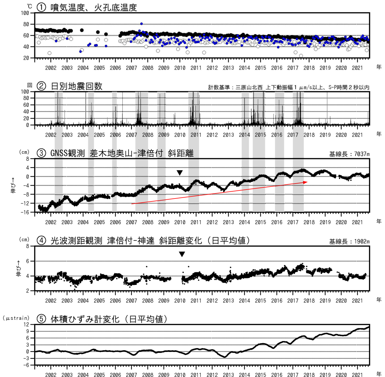
図2 伊豆大島 最近の火山活動経過図（2001年1月～2021年9月30日）
