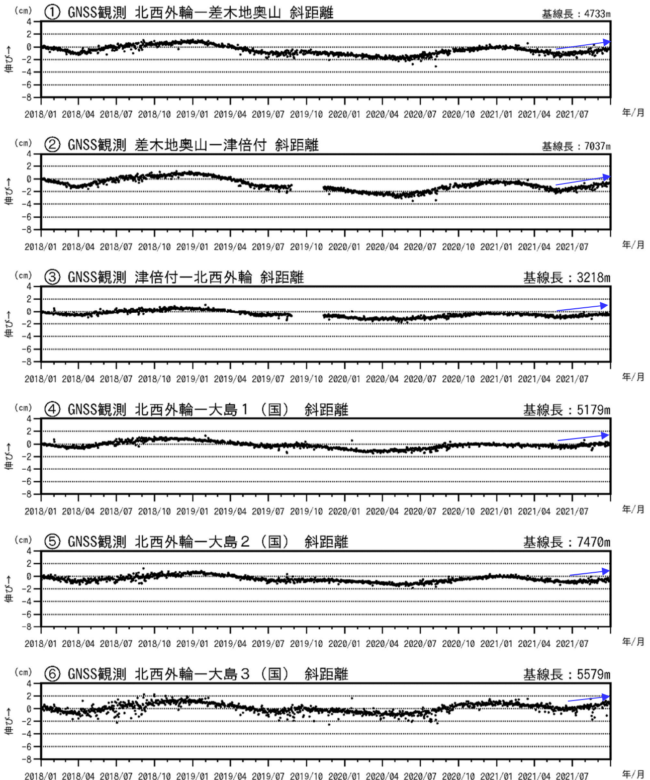
図3-2 伊豆大島 GNSS 連続観測による基線長変化(2018年1月～2021年9月30日)
