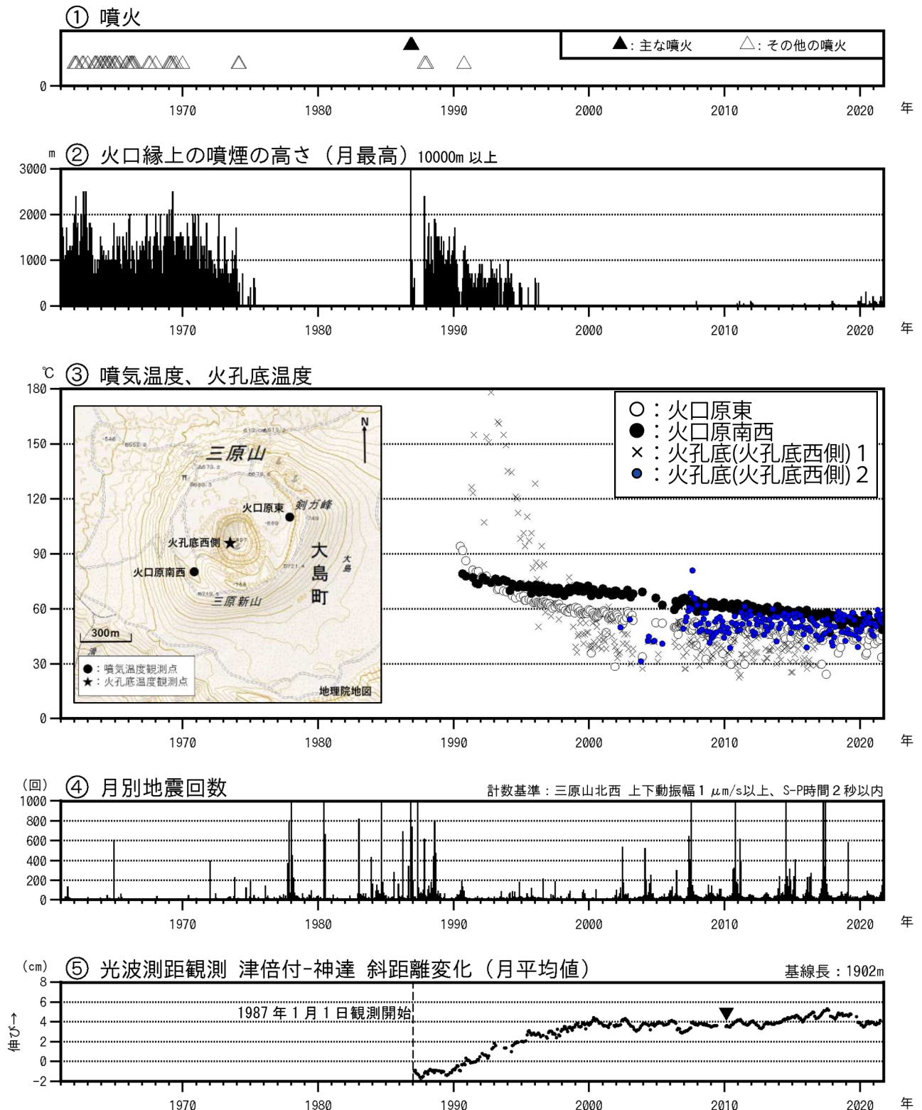
図1 伊豆大島 長期間の火山活動経過図（1961年1月～2021年9月30日）
