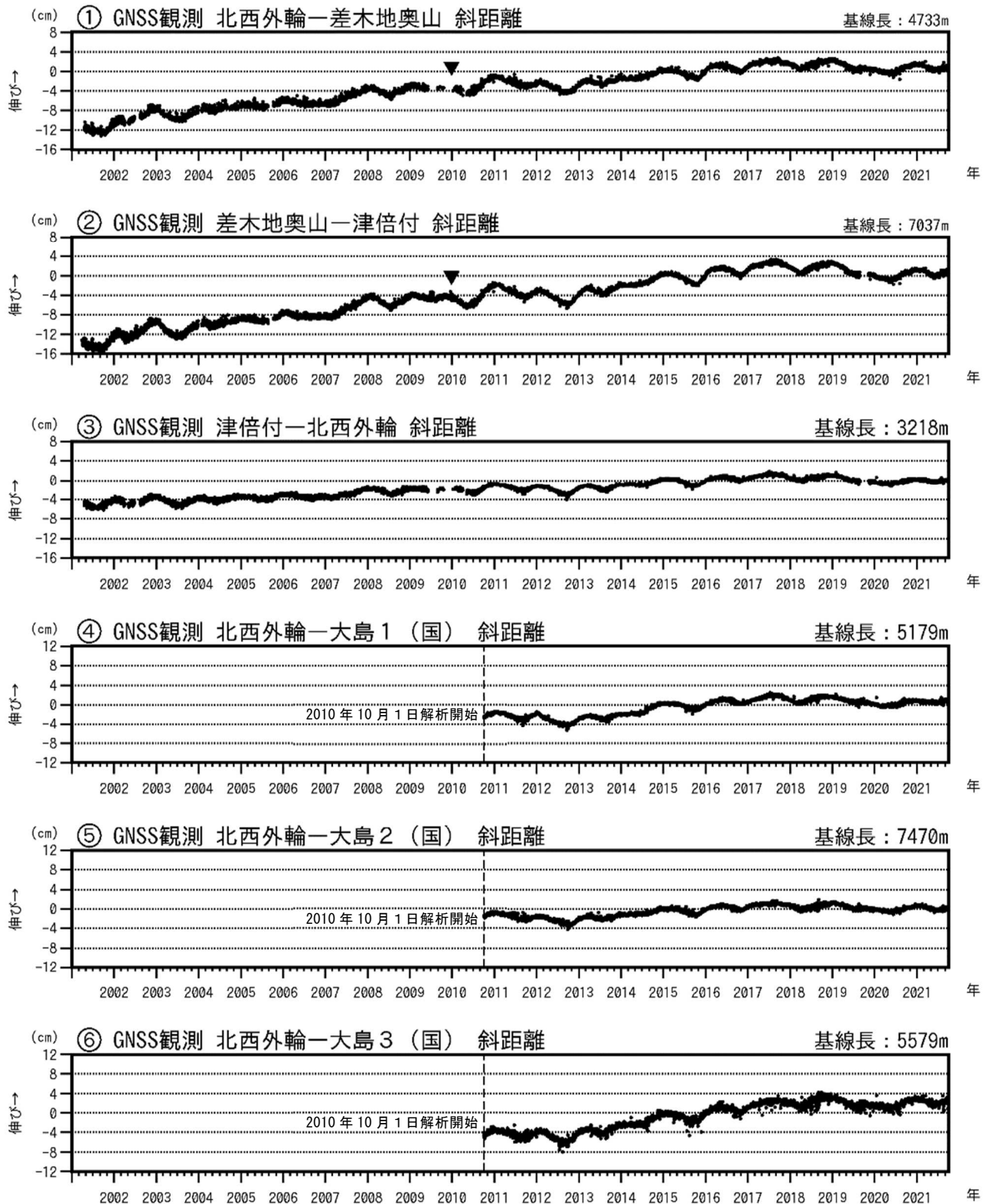
図3-1 伊豆大島 GNSS 連続観測による基線長変化(2001年1月～2021年9月30日)
