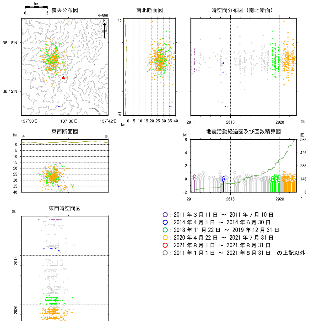
図9 焼岳 広域地震観測網による深部低周波地震の震源分布図（2011年1月1日～2021年8月31日） 広域地震観測網により震源決定したもので、深さは全て海面以下として決定しています。そのため、山頂付近の浅い地震の震源も海面下に決定されています。
