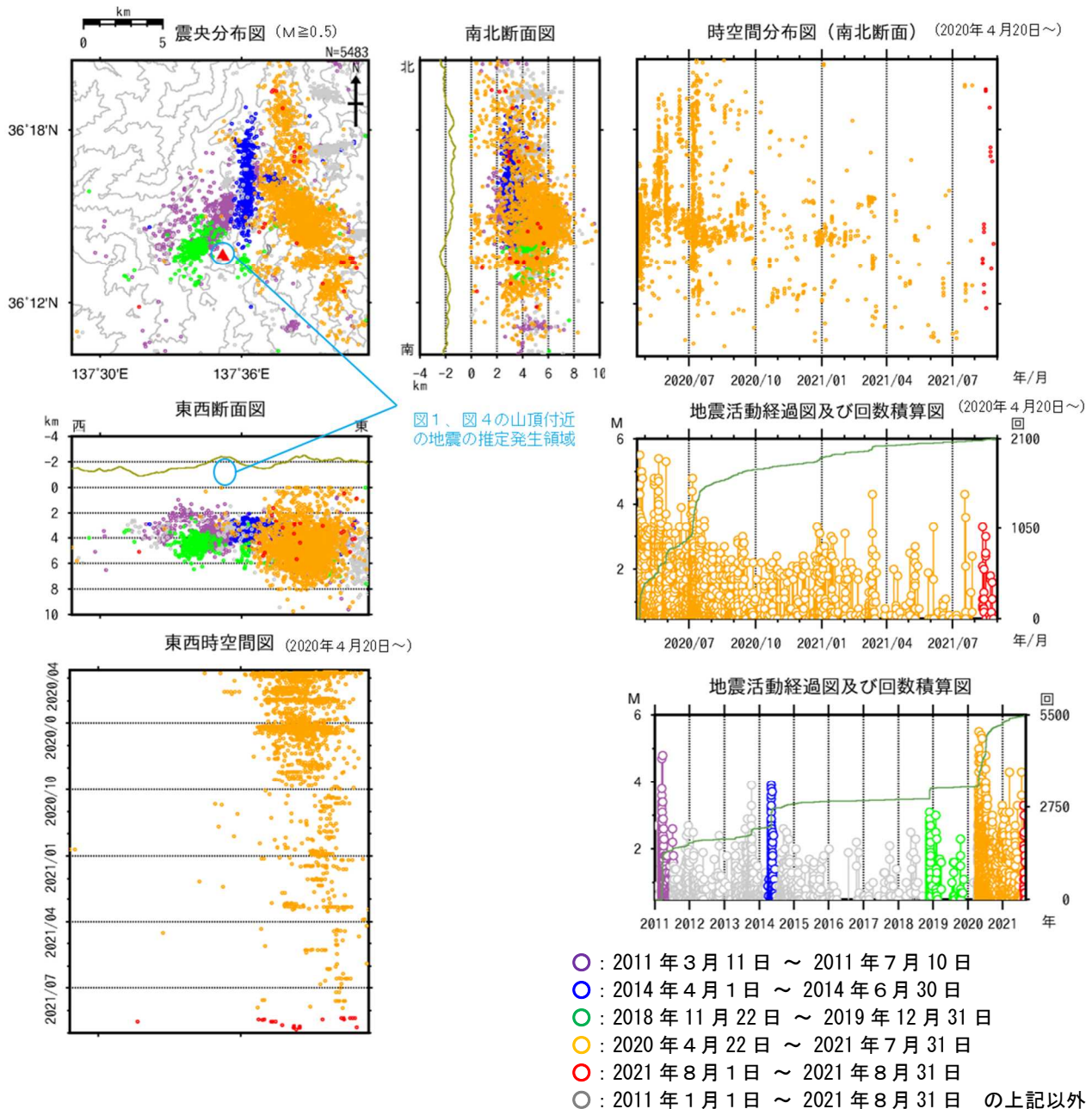
図8 焼岳 広域地震観測網による山体及び周辺の地震活動(2011年1月1日～2021年8月31日)
