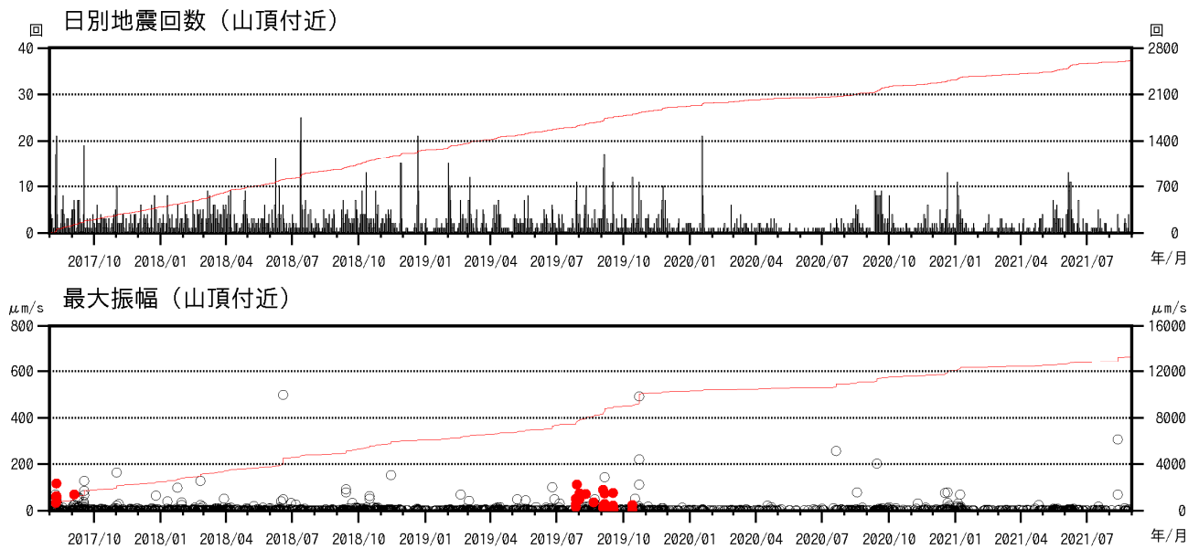
図1 焼岳 山頂付近の地震回数、及び南峰南東観測点上下動最大振幅 (2017年8月1日～2021年8月31日)
