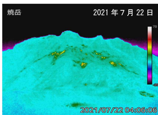
図3 焼岳 中尾峠赤外熱映像カメラによる焼岳の北側斜面の地表面温度分布と可視画像 撮影場所と撮影方向は図10を参照下さい。
