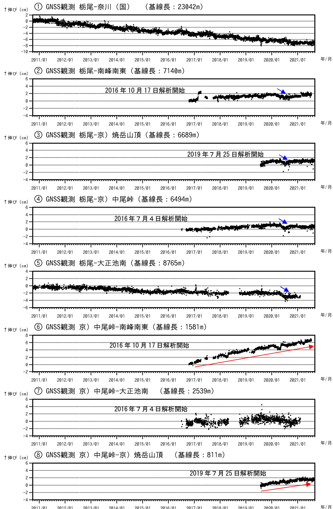
図5 焼岳 GNSS連続観測による基線長変化（2010年10月1日～2021年8月31日）
