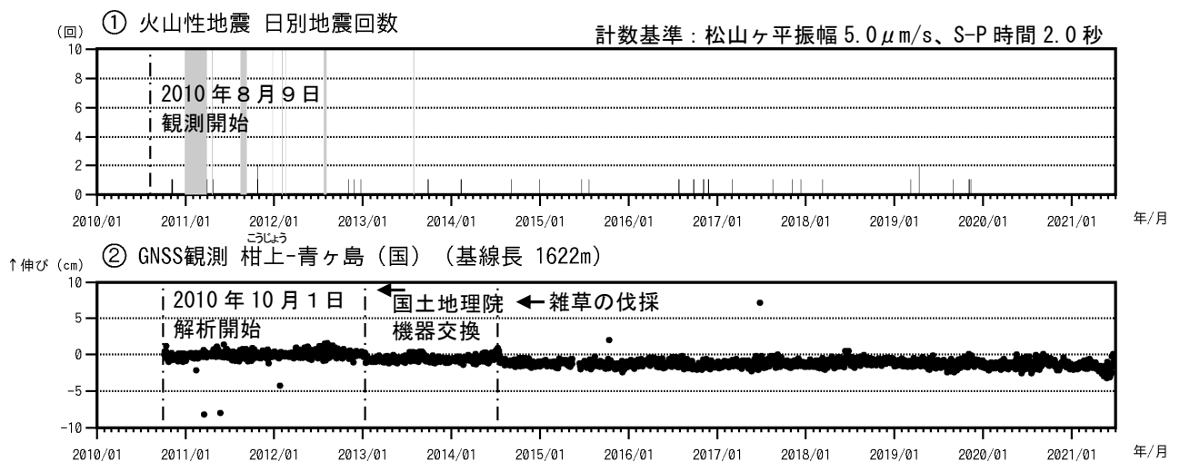
図3 青ヶ島 火山活動経過図（2010年8月9日～2021年6月30日）
