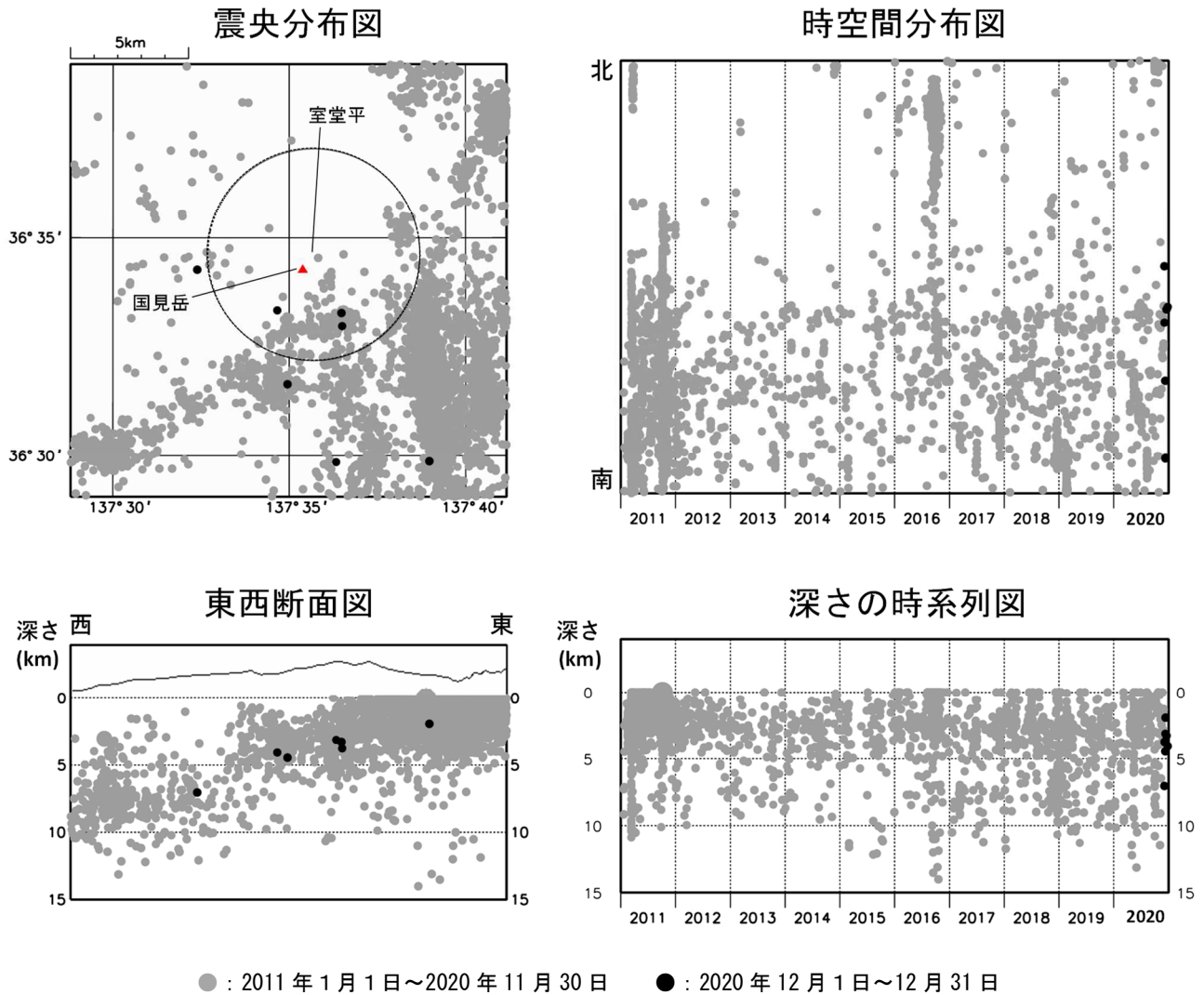
図2 弥陀ヶ原 広域地震観測網による山体・周辺の地震活動（2011 年 1 月 1 日～2020 年 12 月 31 日） 震央分布図中の円は弥陀ヶ原の計数対象地震（室堂平で S-P 時間 1 秒以内）のおよその範囲を示しています。 広域地震観測網により震源決定したもので、深さは全て海面以下として決定しています。 図中の震源要素は一部暫定値が含まれており、後日変更することがあります。 この図では、関係機関の地震波形を一元的に処理し、地震観測点の標高を考慮する等した新手法で得られた震源を用いています（ただし、2020 年 8 月以前の地震については火山活動評価のための参考震源です）。 2021 年 1 月 12 日現在、2020 年 4 月 18 日から 10 月 23 日までの地震について、暫定的に震源精査の基準を変更しているため、その前後の期間と比較して微小な地震での震源決定数の変化（増減）が見られます。 ・今期間、地獄谷周辺の地震活動は、低調に経過しています。
