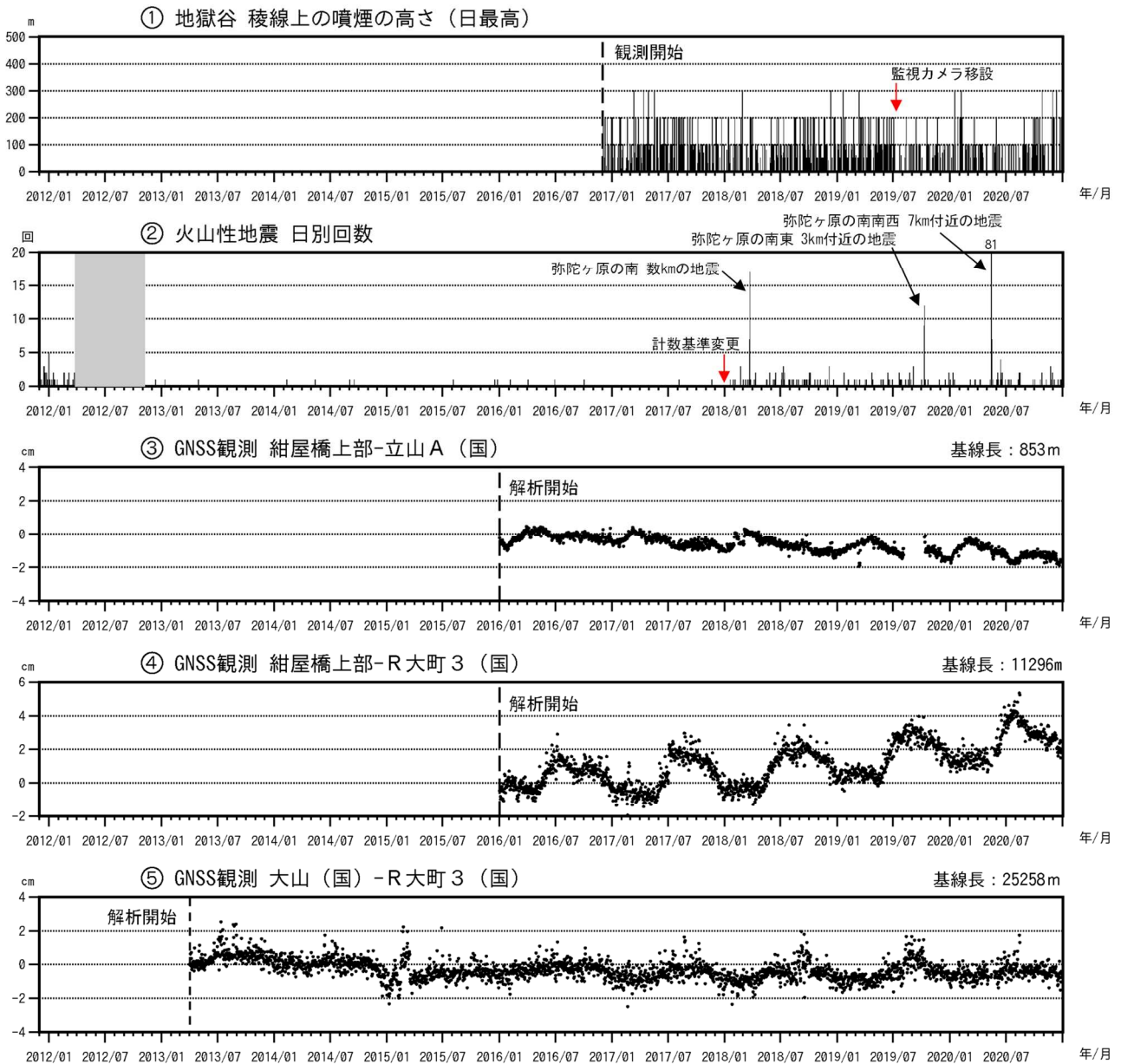
図3 弥陀ヶ原 火山活動経過図（2011年12月1日～2020年12月31日）
