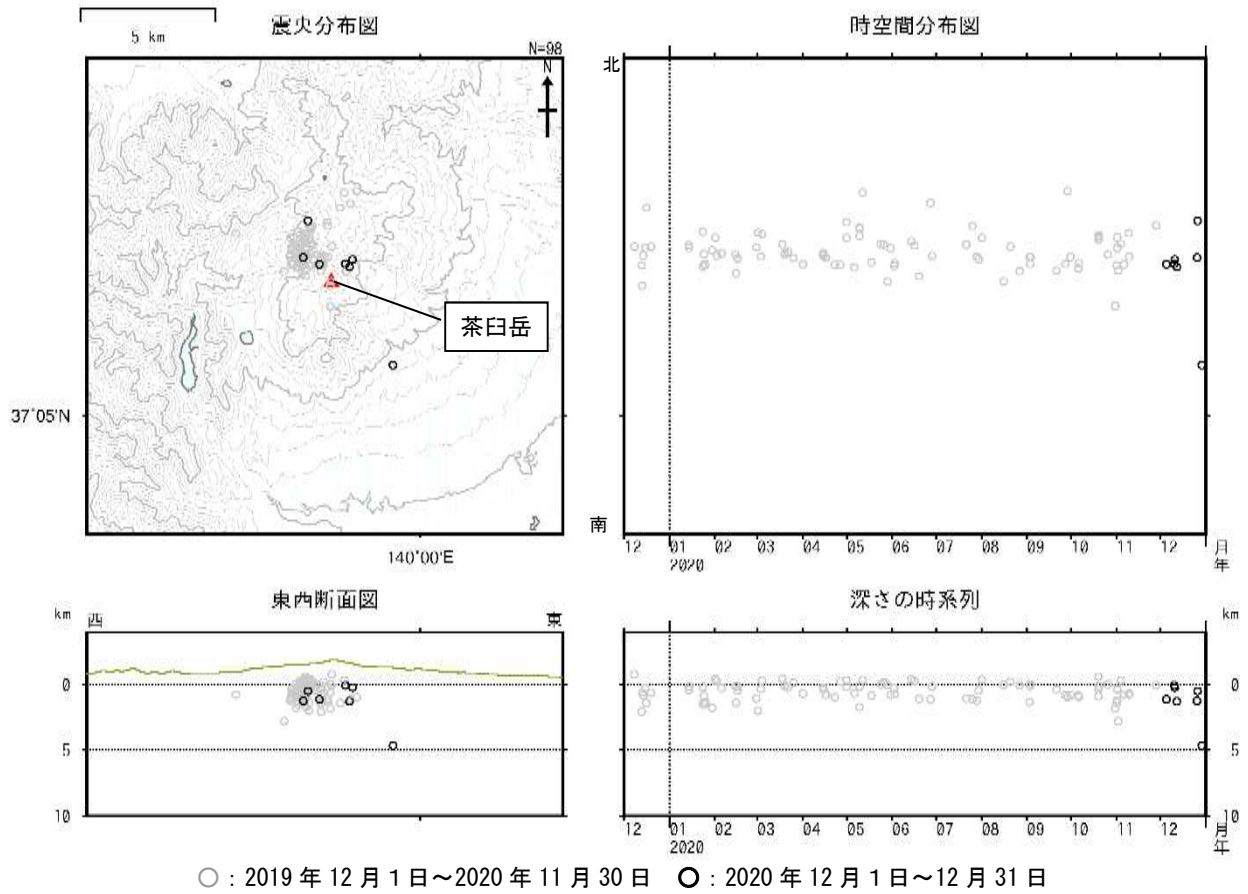
図5 那須岳 震源分布図（2019年12月1日～2020年12月31日）
