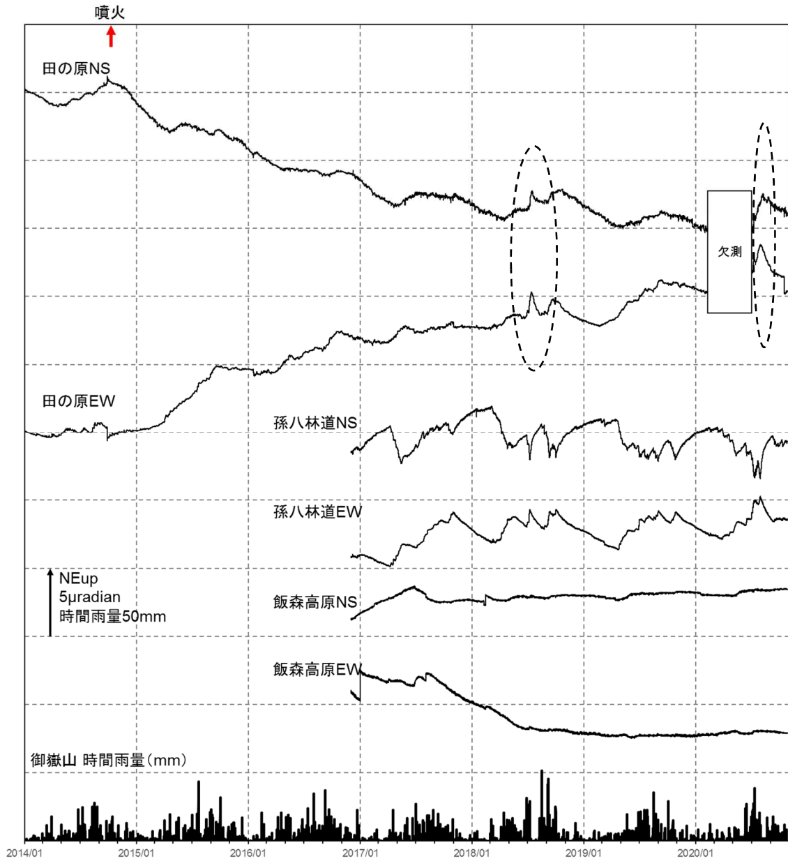
図7 御嶽山 傾斜変動（2014年1月1日～2020年10月31日）
