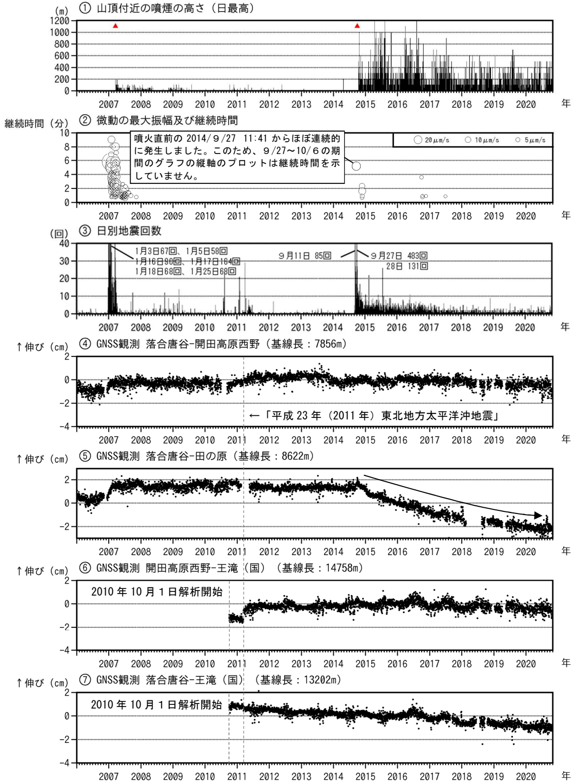
図5 御嶽山 長期間の火山活動経過図（2006年1月1日～2020年10月31日） ①監視カメラによる噴煙の高さ 噴煙の高さは日最大値。赤三角シンボルは噴火発生を示します。 ②火山性微動の最大振幅は田の原上観測点の上下振幅です（火山性微動の発生した2015年7月20日、2016年5月19日は欠測です）。 ④～⑦GNSS連続観測による基線長変化。（国）：国土地理院 2010年10月及び2016年1月以降のデータについては、解析方法を変更しています。空白部分は欠測を示します。 ⑤の基線では、2014年10月以降山体の収縮によると考えられる縮みの傾向が続いています。 ⑥には「平成23年（2011年）東北地方太平洋沖地震」に伴うステップ状の変化がみられます。 図中④～⑦は図6のGNSS基線④～⑦に対応します。
