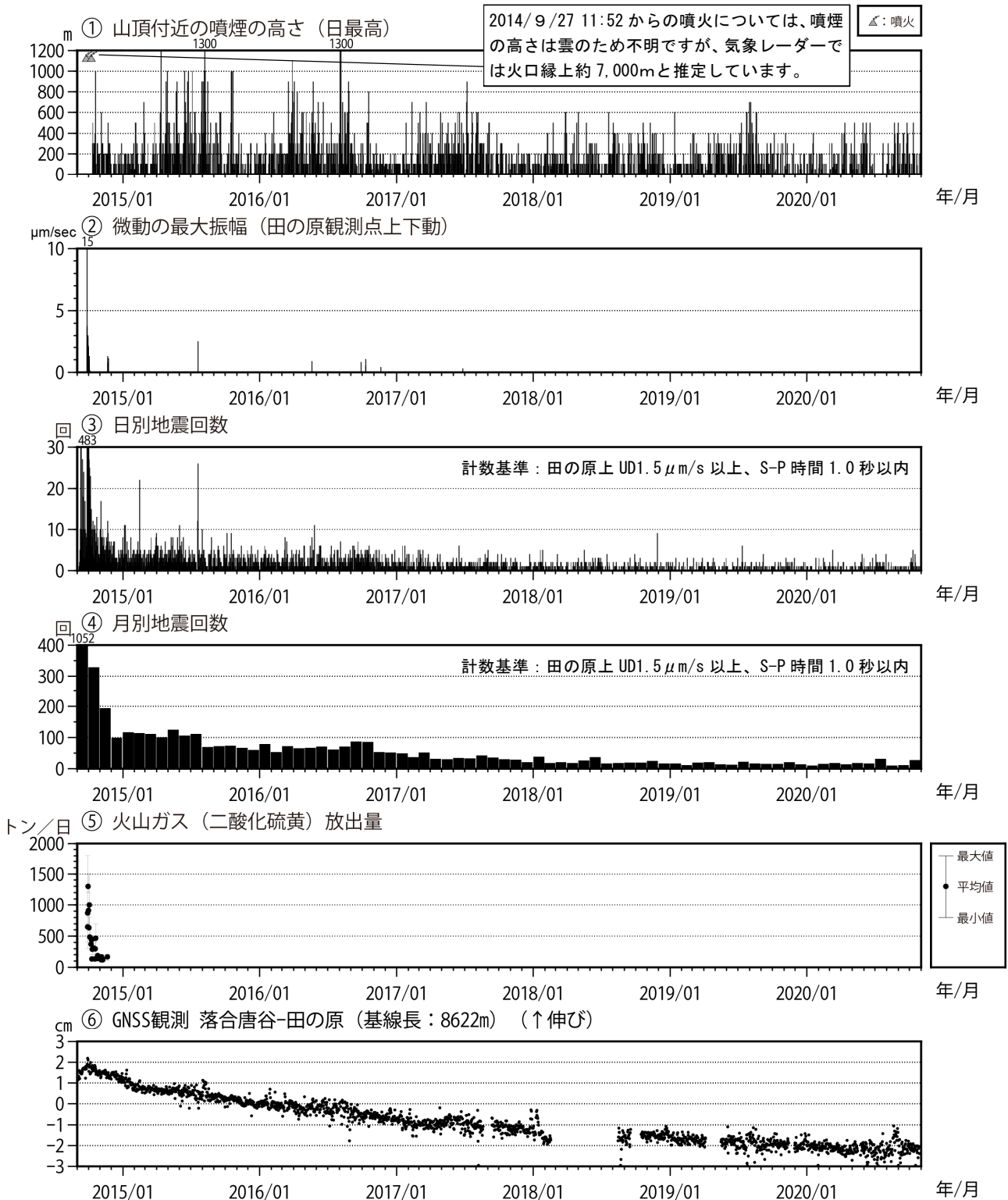
図4 御嶽山 最近の火山活動経過図（2014年9月1日～2020年10月31日）
