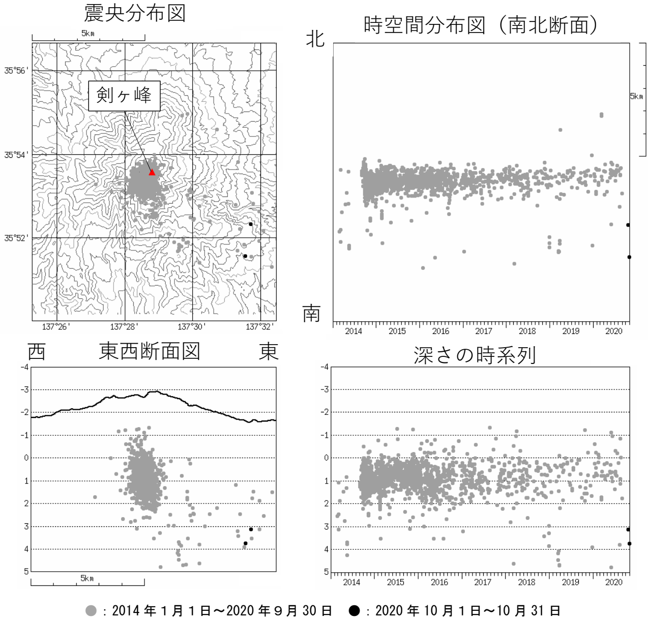
図3 御嶽山 震源分布図（2014年1月1日～2020年10月31日）
