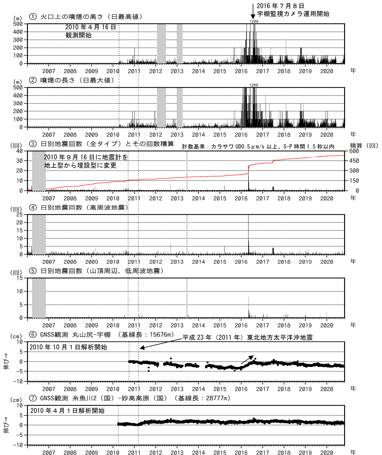
図2 新潟焼山 火山活動経過図（2006年1月1日～2020年10月31日）
