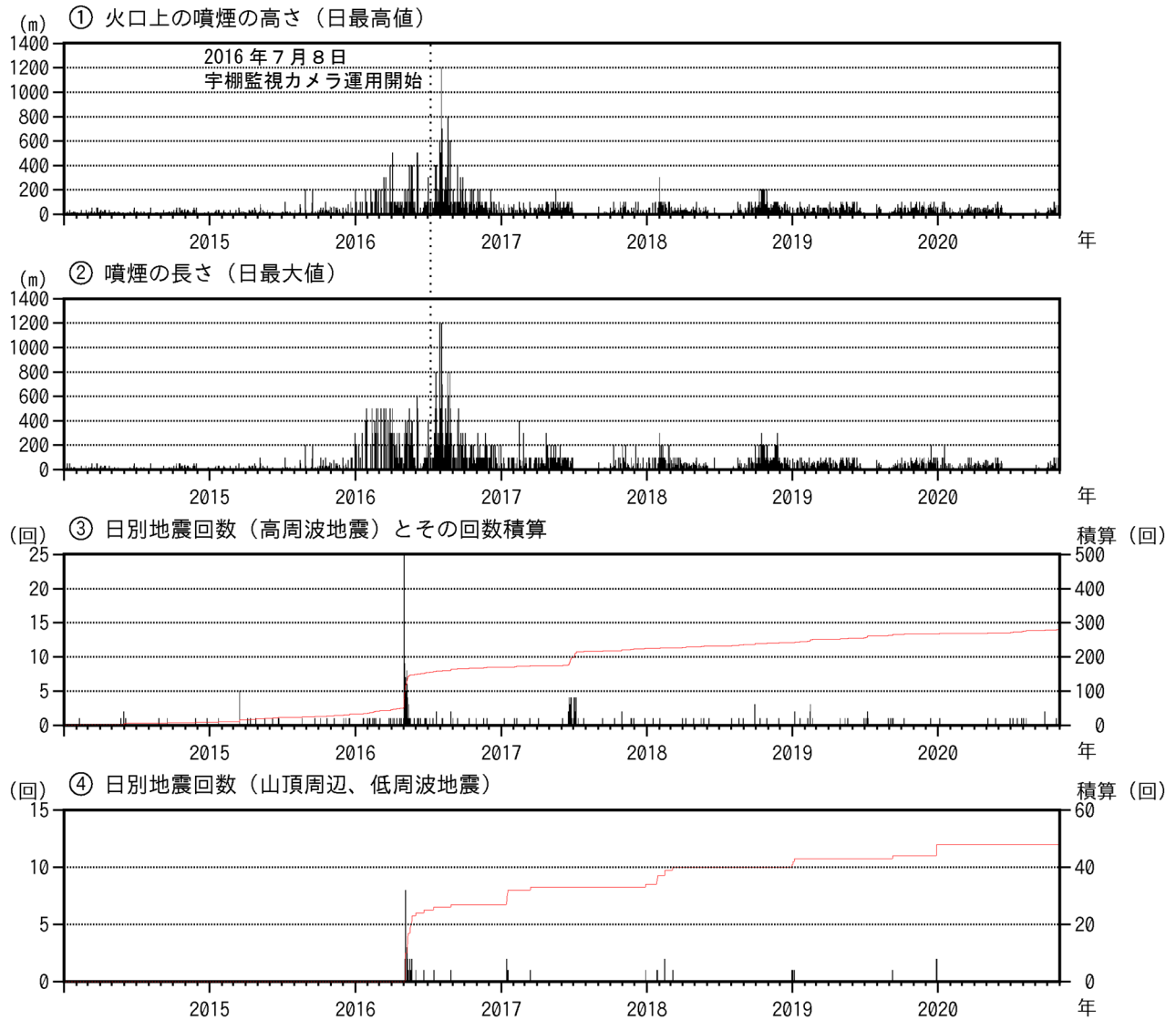
図3 新潟焼山 火山活動経過図（短期）（2014年1月1日～2020年10月31日）
