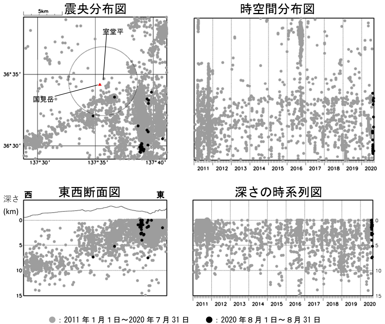
図2 弥陀ヶ原 広域地震観測網による山体・周辺の地震活動（2011 年 1 月 1 日～2020 年 8 月 31 日）
