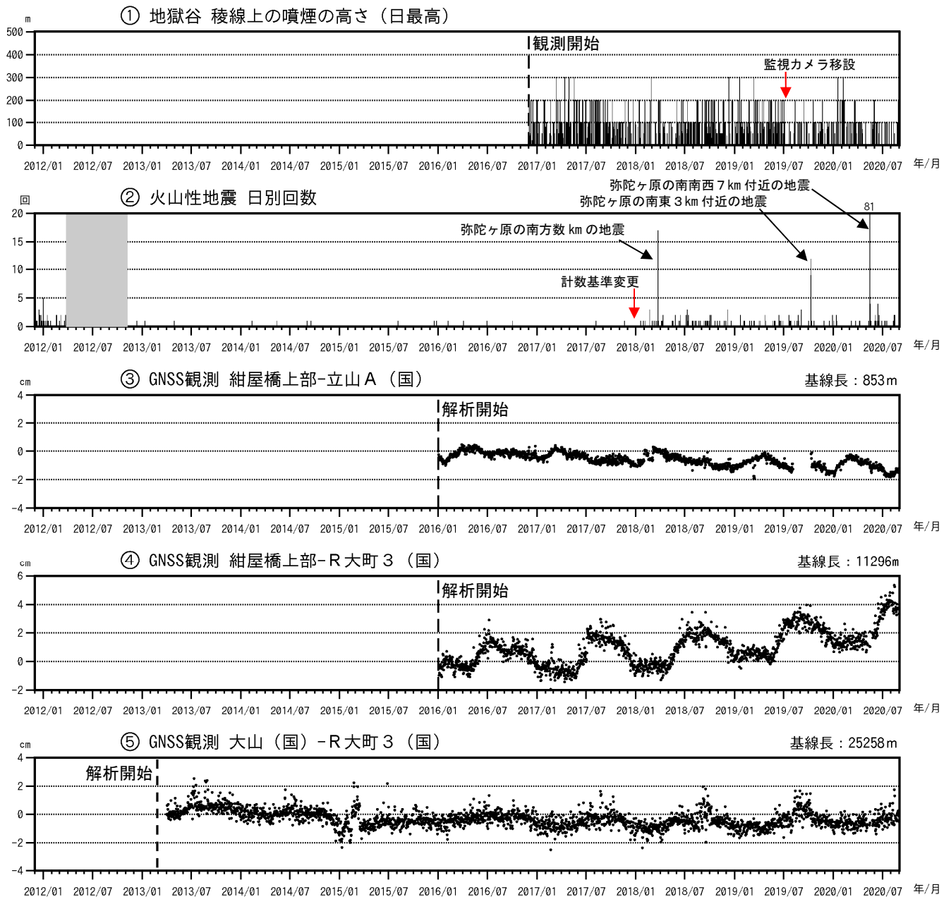
図3 弥陀ヶ原 火山活動経過図（2011年12月1日～2020年8月31日）
