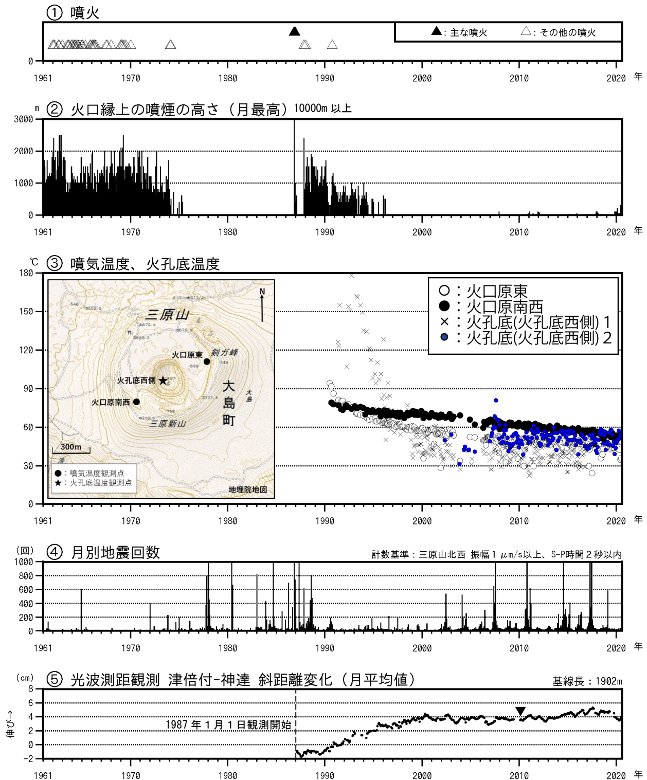
図1 伊豆大島 長期間の火山活動経過図（1961年1月～2020年7月31日）
