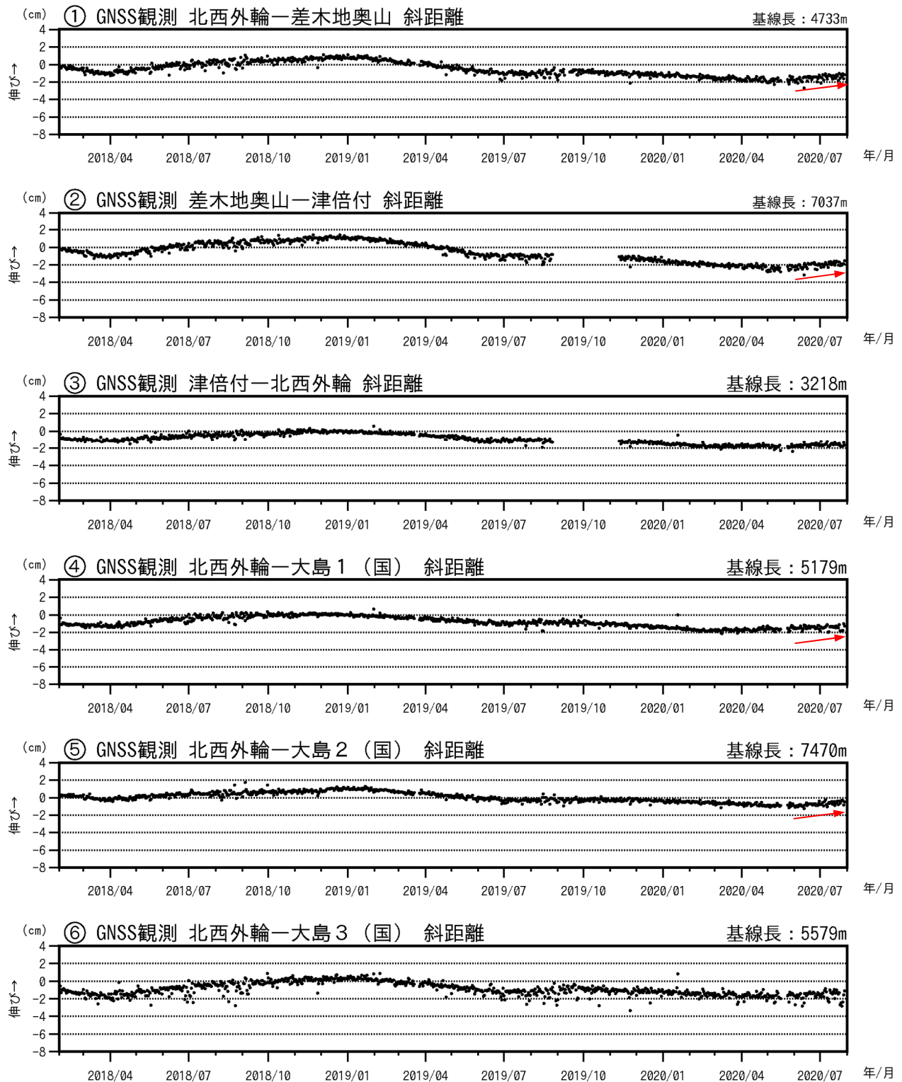
図3-2 伊豆大島 GNSS連続観測による基線長変化(2018年2月～2020年7月31日)
