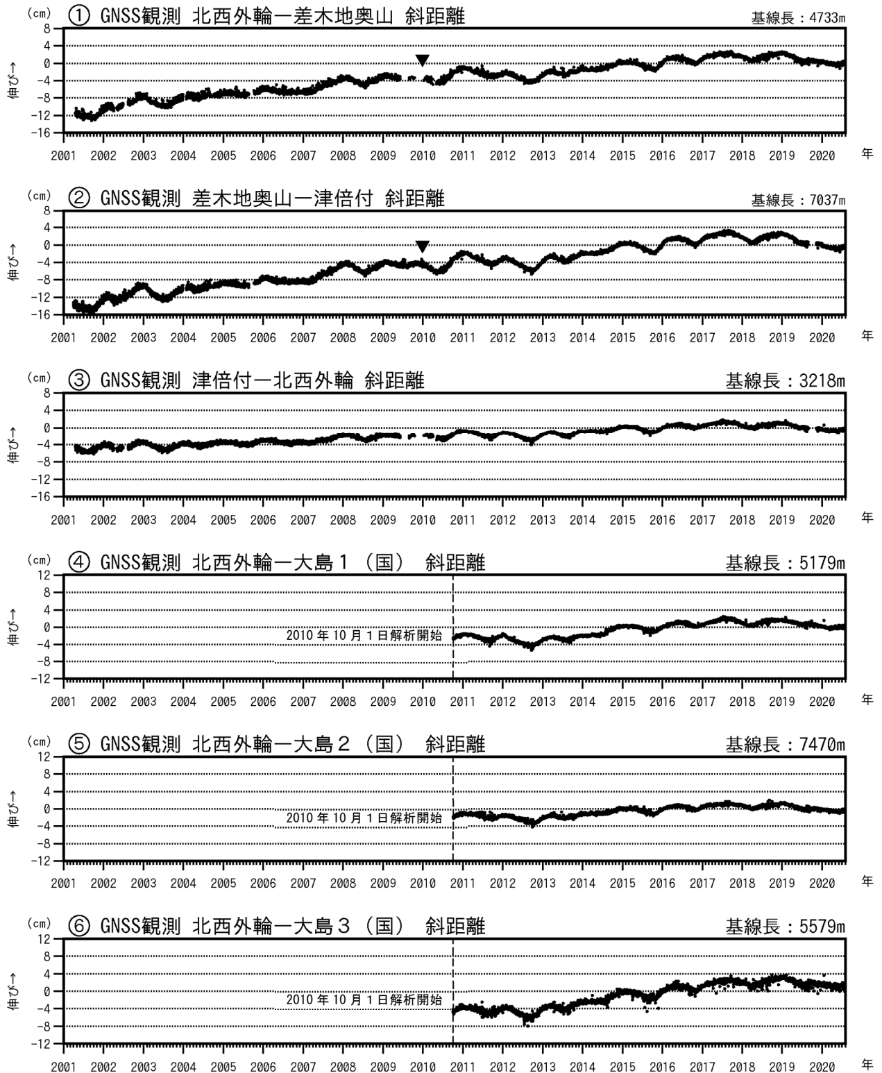
図3-1 伊豆大島 GNSS 連続観測による基線長変化(2001年1月～2020年7月31日)
