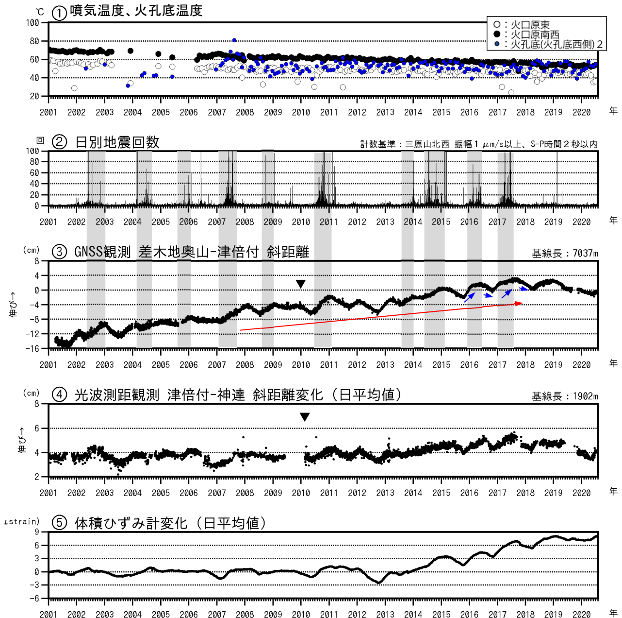
図2 伊豆大島 最近の火山活動経過図（2001年1月～2020年7月31日）
