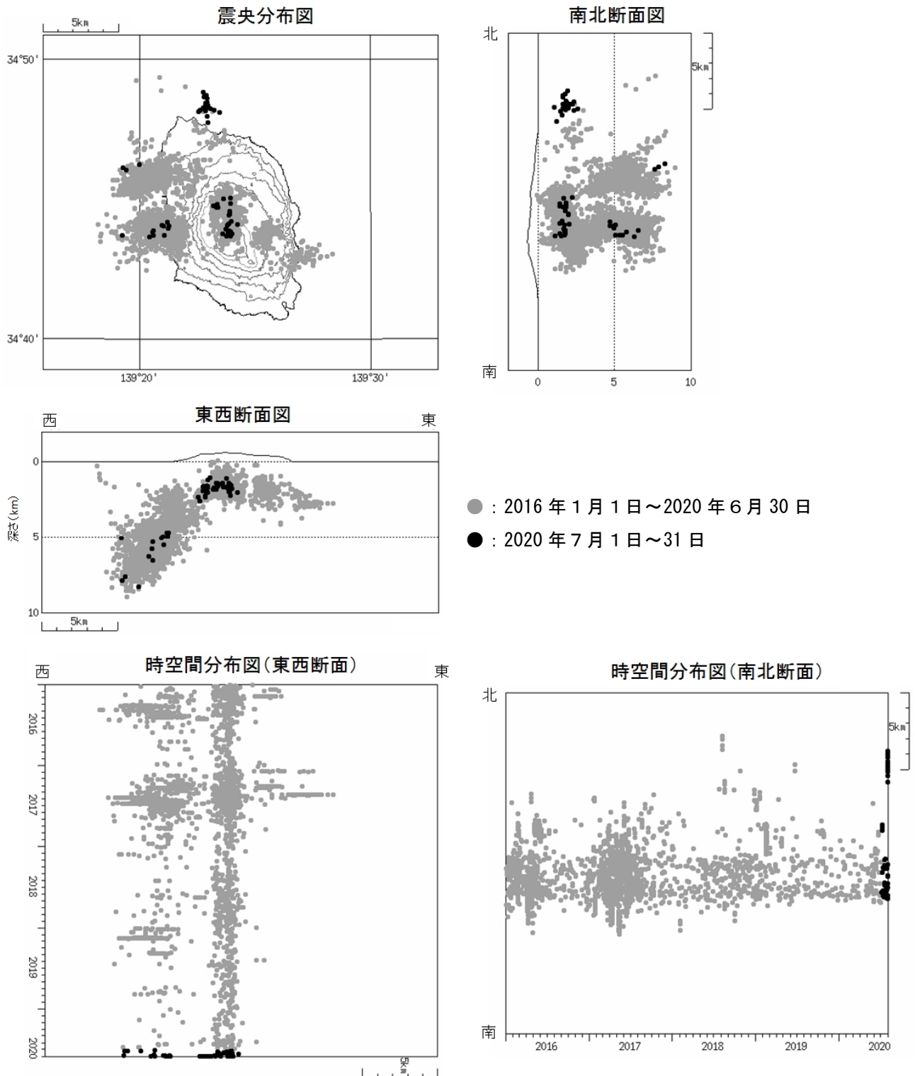
図4 伊豆大島 震源分布図（2016年1月1日～2020年7月31日）
