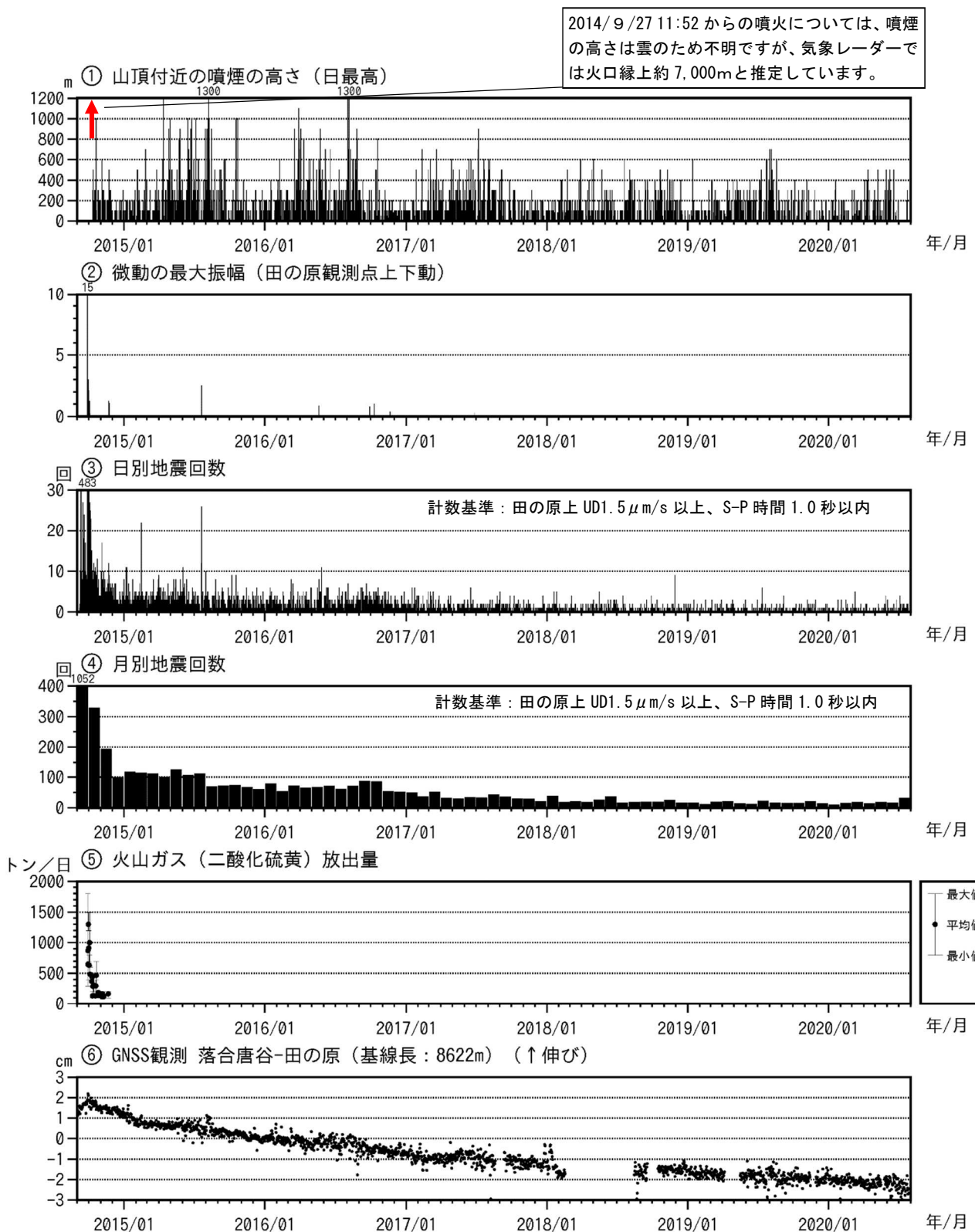
図4 御嶽山 最近の火山活動経過図（2014年9月1日～2020年7月31日）
