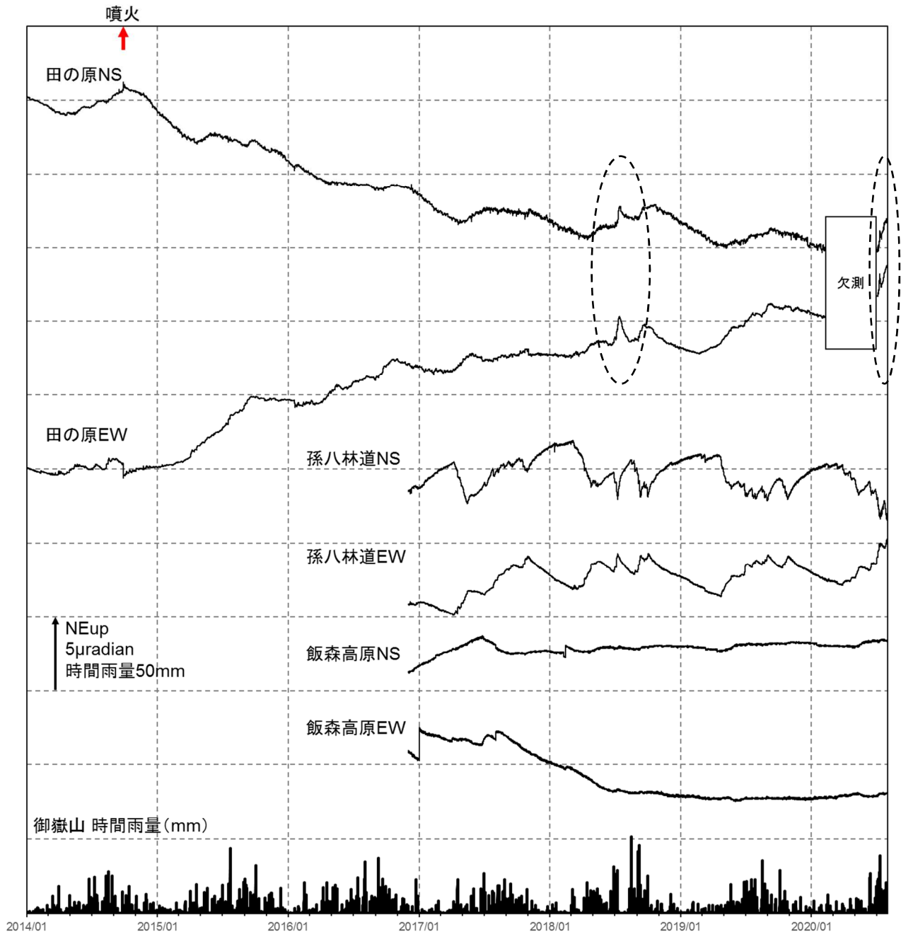
図7 御嶽山 傾斜変動（2014年1月1日～2020年7月31日）
