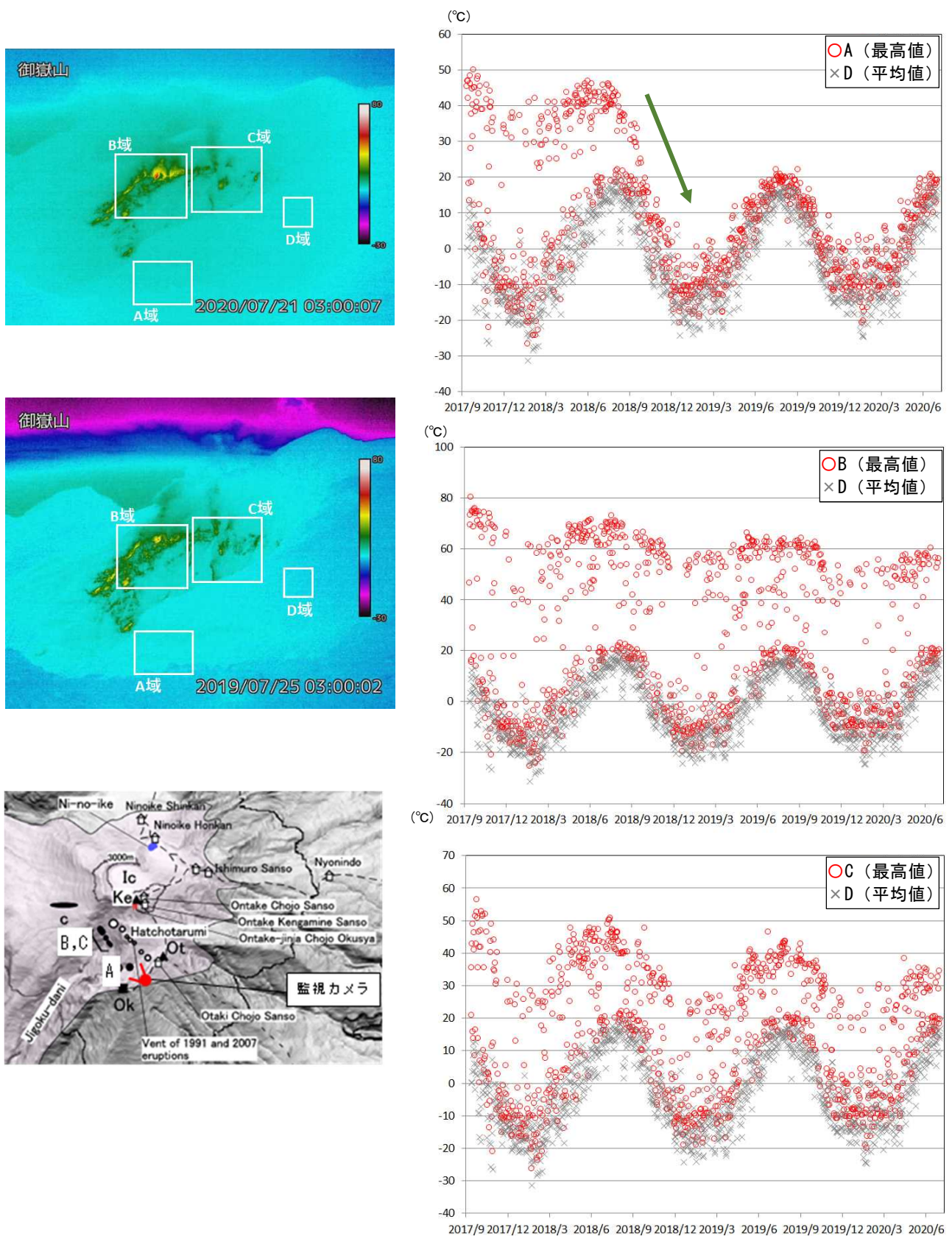
図3 御嶽山 奥の院赤外熱映像カメラによる剣ヶ峰南西側における最高温度の推移 (2017年9月13日～2020年7月31日)と同カメラの位置(左下図はOikawa et al., 2016に加筆) A～Cは地熱域、Dは非地熱域を示します。 ・年周変化はみられるものの、B及びC領域については長期的な低下傾向となっています。 ・A領域の温度は2018年秋頃から明瞭に低下し、非地熱域と同程度の温度となっています(緑矢印)。
