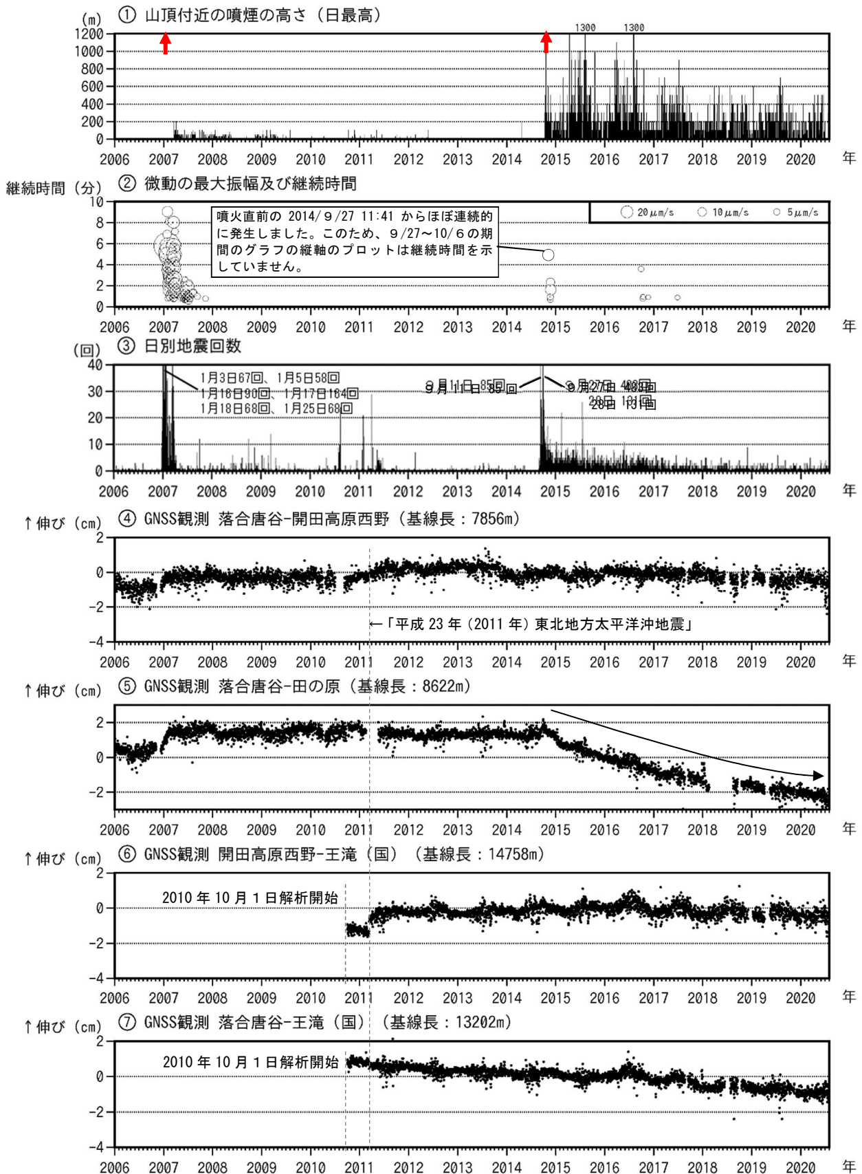
図5 御嶽山 長期間の火山活動経過図（2006年1月1日～2020年7月31日）
