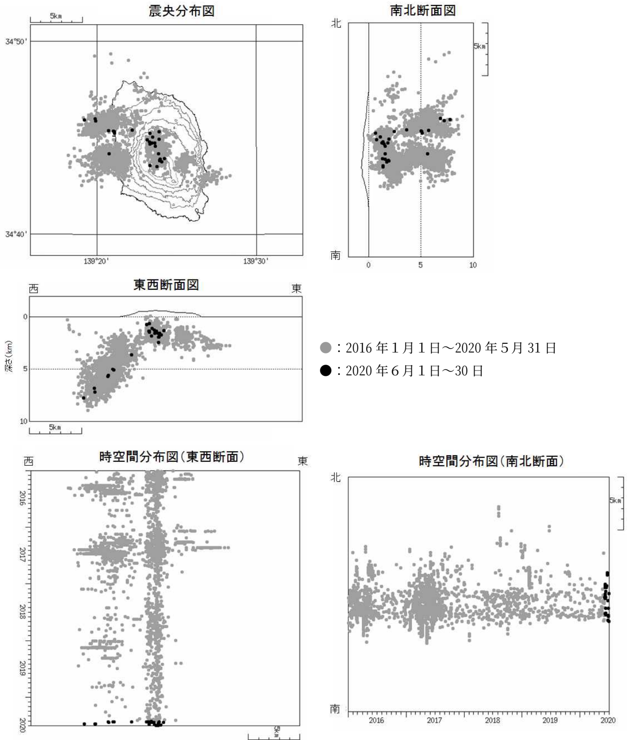
図4 伊豆大島 震源分布図（2016年1月1日～2020年6月30日）
