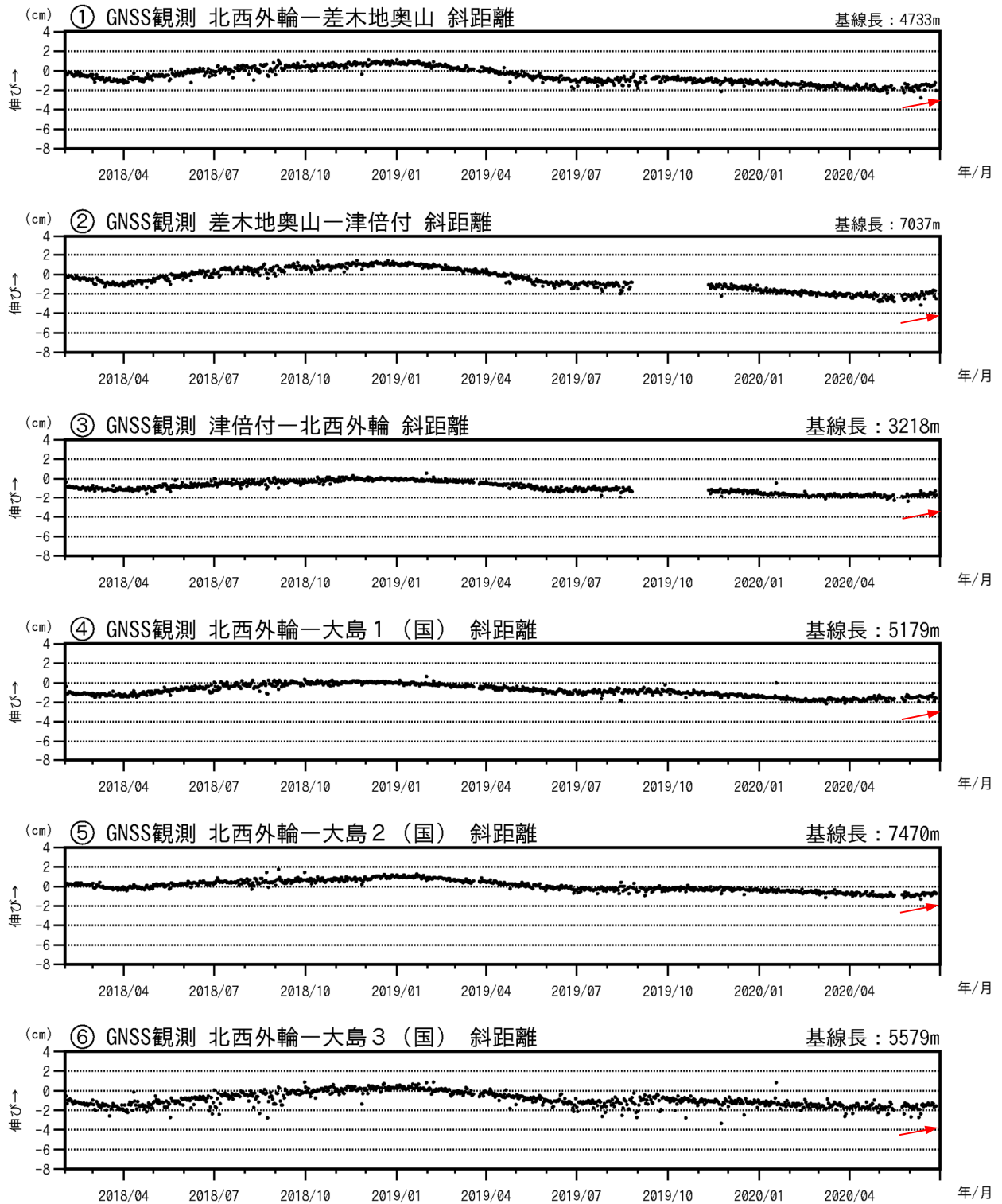
図3-2 伊豆大島 GNSS 連続観測による基線長変化(2018年2月～2020年6月30日)
