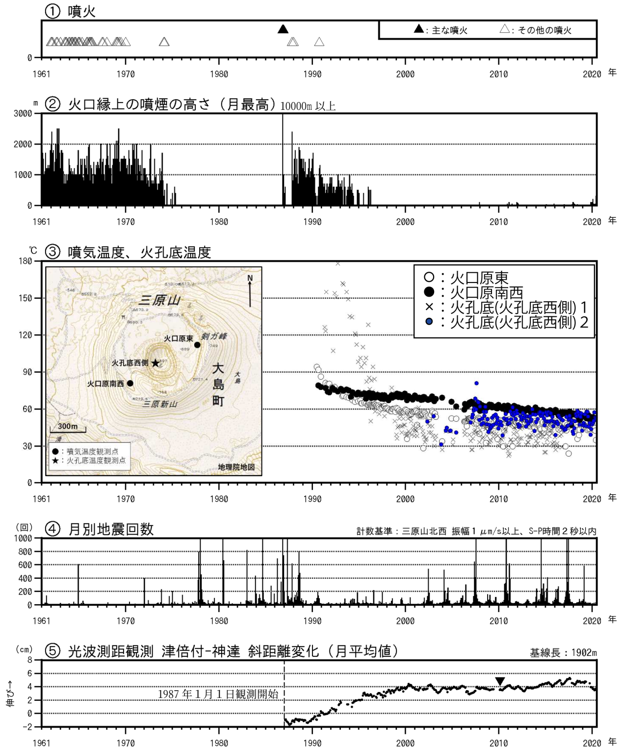
図1 伊豆大島 長期間の火山活動経過図（1961 年 1 月～2020 年 6 月 30 日）
