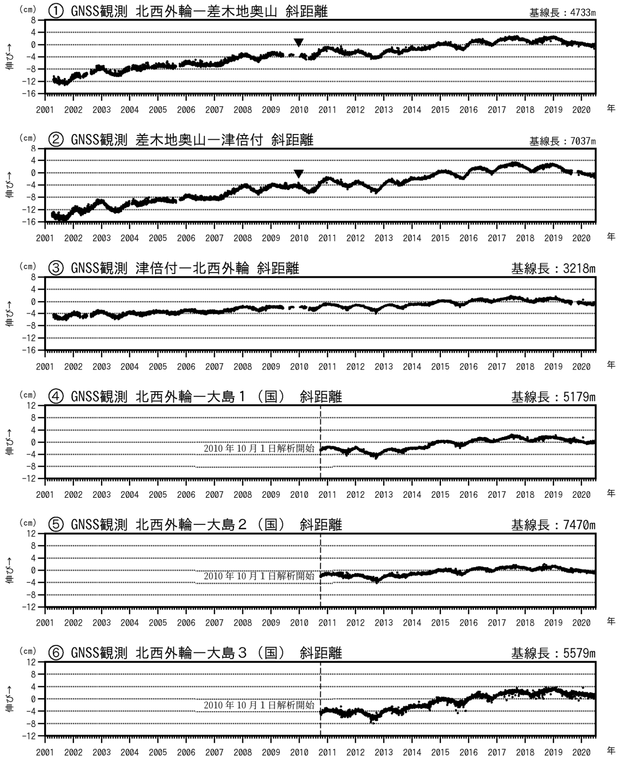
図3-1 伊豆大島 GNSS連続観測による基線長変化(2001年1月～2020年6月30日)
