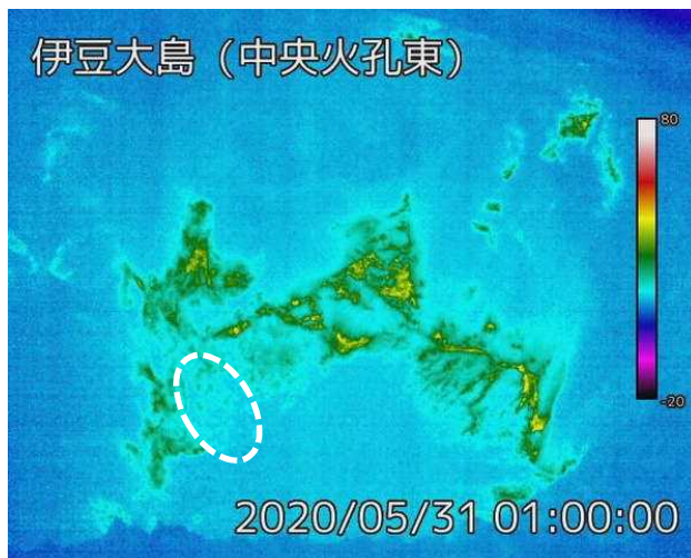
2020年5月31日 中央火孔東監視カメラによる
