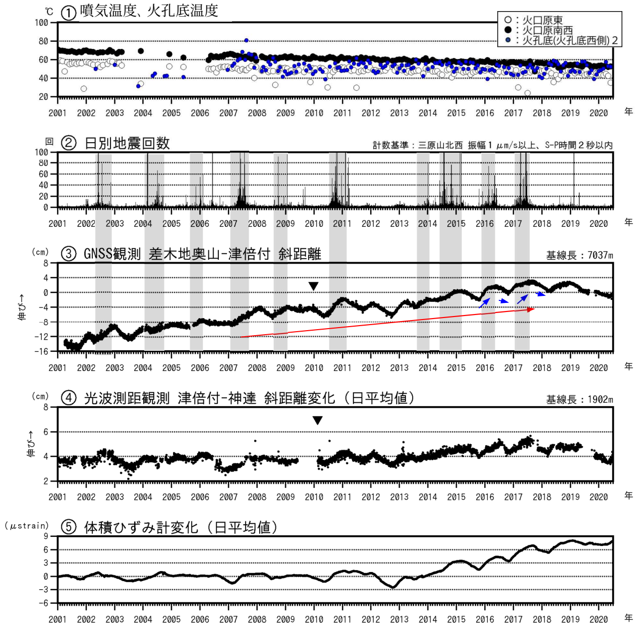
図2 伊豆大島 最近の火山活動経過図（2001年1月～2020年6月30日）
