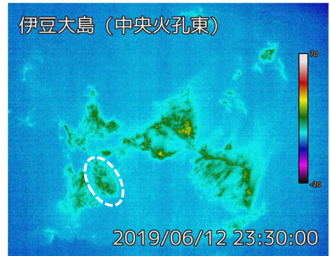
2019年6月12日 中央火孔東監視カメラによる
