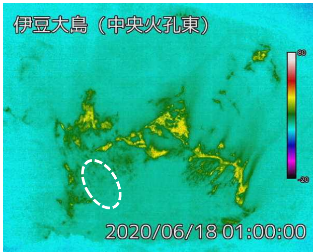
2020年6月18日 中央火孔東監視カメラによる
