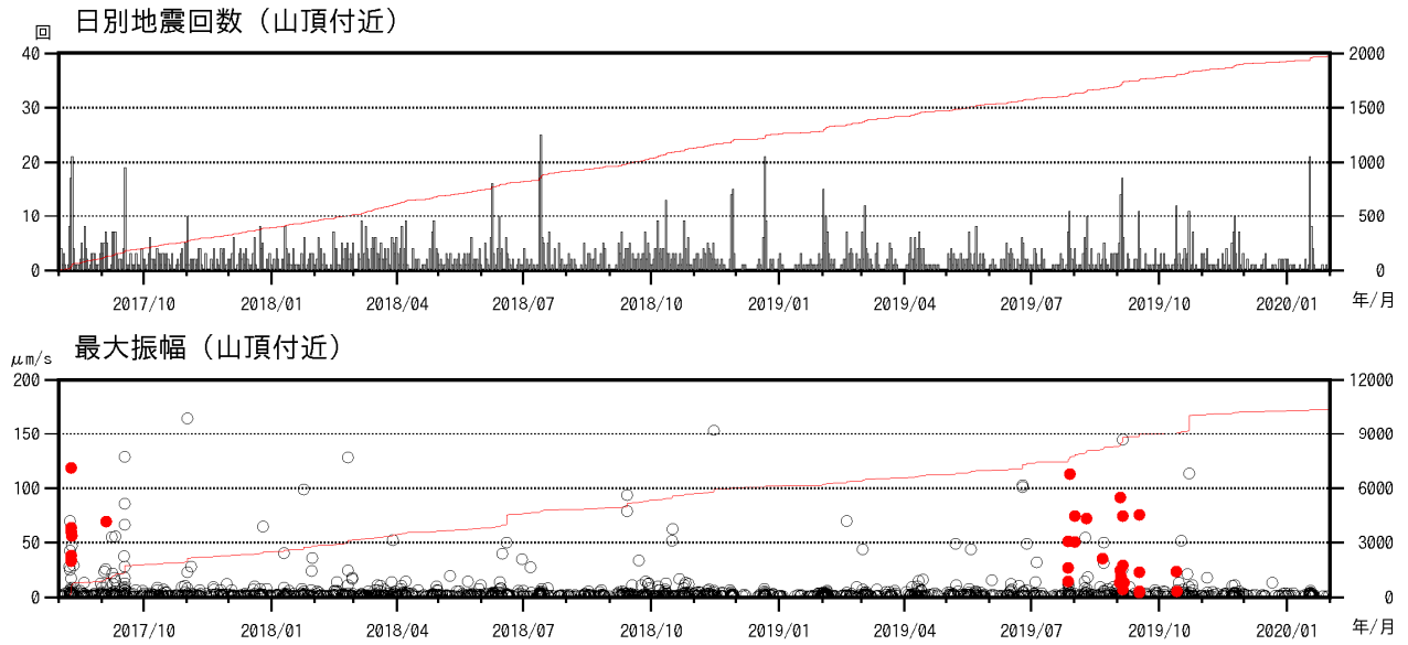
図4 焼岳 山頂付近の地震回数、および南峰南東観測点上下動最大振幅 (2017年8月1日～2020年1月31日)
