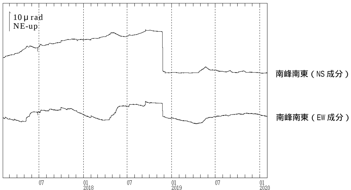
図7 焼岳 南峰南東観測点における傾斜データ (2017年2月1日～2020年1月31日)
