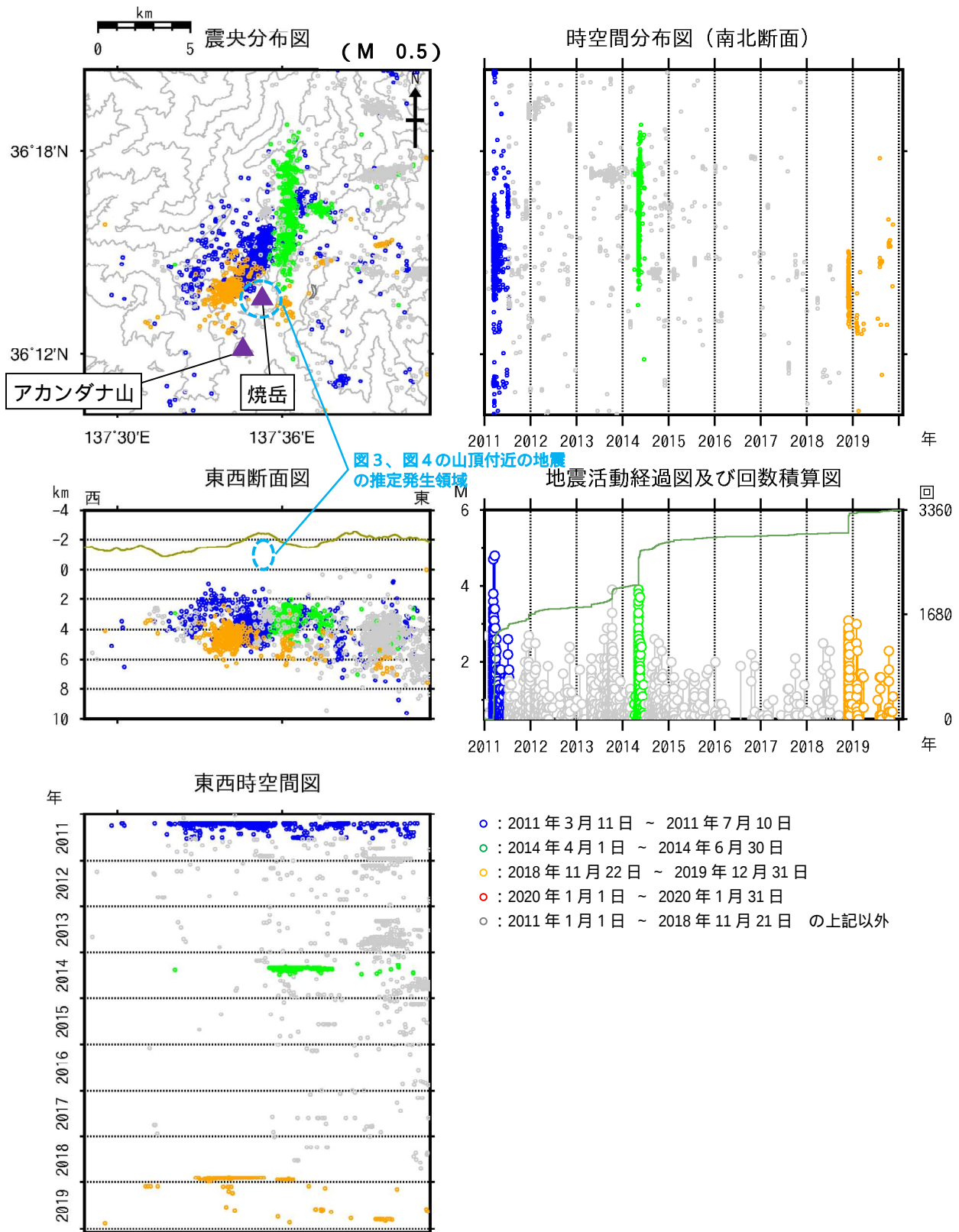
図5 焼岳 広域地震観測網による山体及び周辺の地震活動(2011年1月1日～2020年1月31日)
