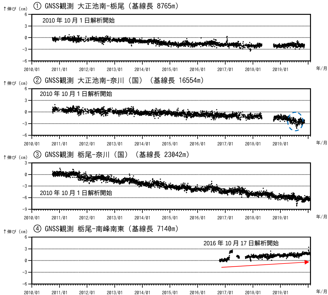
図6 焼岳 GNSS 連続観測による基線長変化 (2010年10月1日～2020年1月31日)
