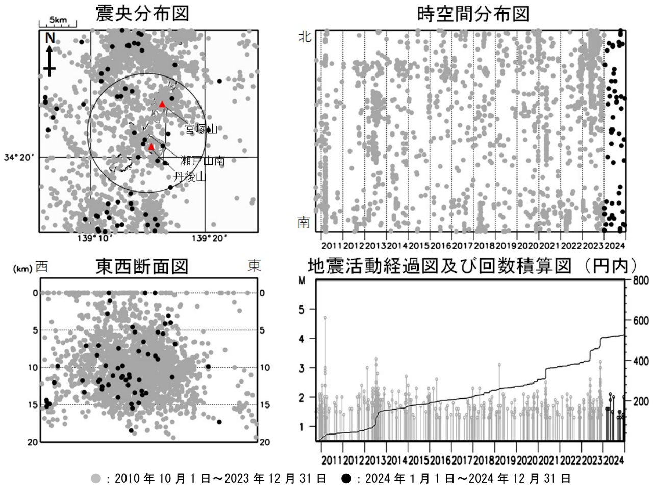
図3 新島 広域地震観測網による山体・周辺の地震活動（2010年10月1日～2024年12月31日） 広域地震観測網により震源決定したもので、深さは全て海面以下として決定しています。 M（マグニチュード）は地震の規模を表し、M1.3以上の地震を示しています。 図中の震源要素は一部暫定値が含まれており、後日変更することがあります。 計数対象（瀬戸山南から半径8km、深さ20km以内）以外の地震が含まれるため、図2-①の日別A型地震回数とは異なります。 震央分布図中の円は火山性地震の回数の計数対象（瀬戸山南から半径8km、深さ20km以内）の範囲を示しています。 この図では、関係機関の地震波形を一元的に処理し、地震観測点の標高を考慮する等した手法で得られた震源を用いています（ただし、2020年8月以前の地震については火山活動評価のための参考震源です）。
