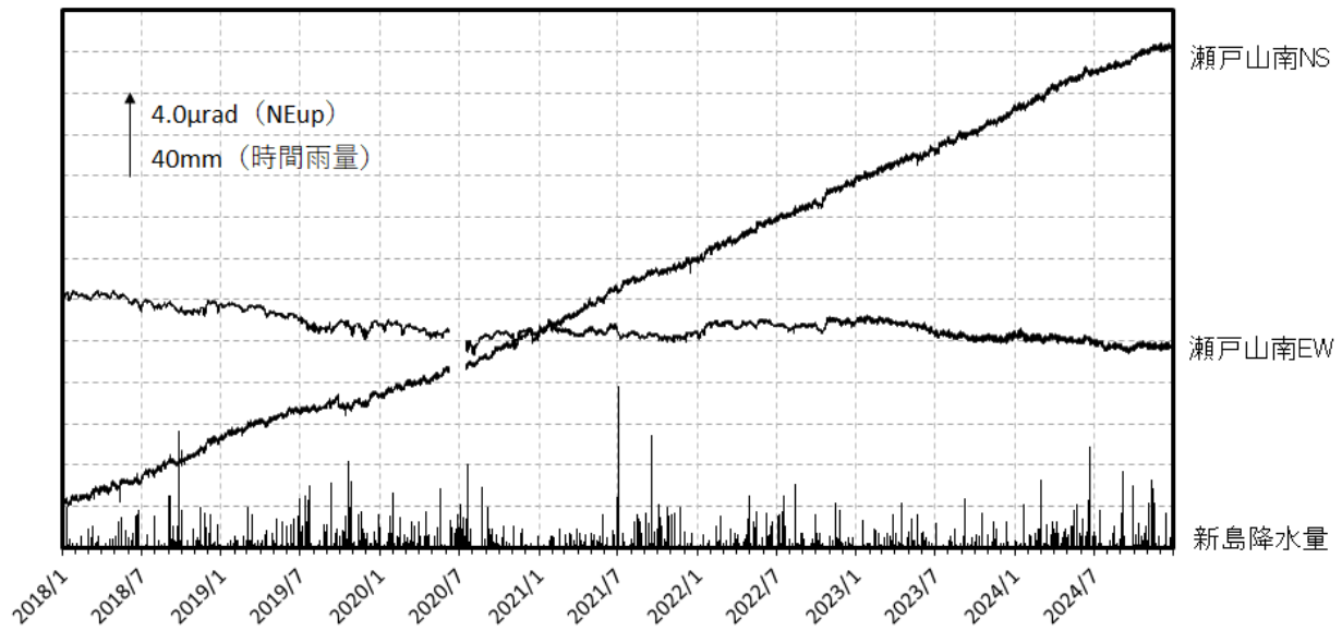
図4 新島 瀬戸山南観測点の傾斜変動（2018年1月1日～2024年12月31日） 図中の空白部分は欠測を示します。
