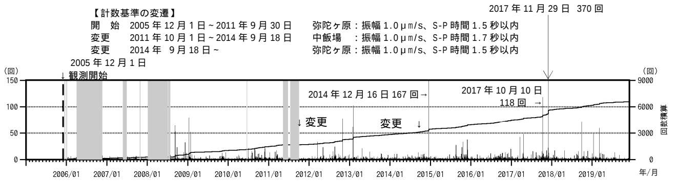
図 3 白山 日別地震回数と積算回数（2005 年 12 月 1 日 ~ 2019 年 11 月 30 日） 図の灰色部分は機器障害による欠測期間
