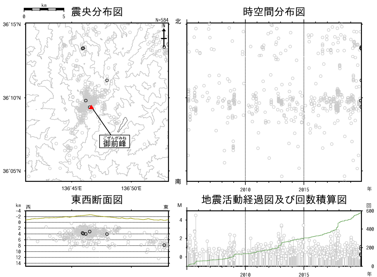
図 4 白山 広域地震観測網による山体・周辺の地震活動（2005 年 1 月 1 日 ~ 2019 年 11 月 30 日）
