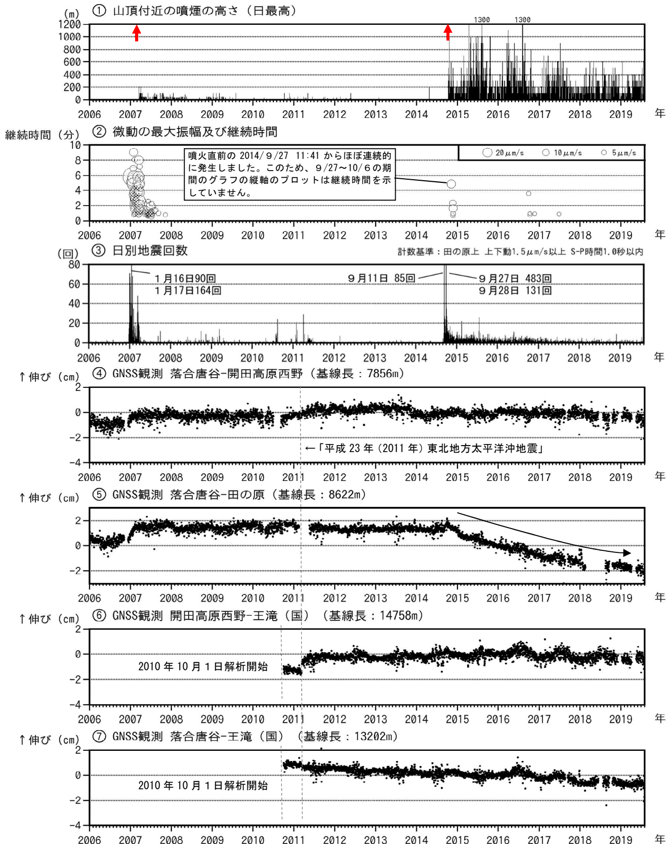
図5 御嶽山 長期間の火山活動経過図（2006年1月1日～2019年7月31日）
