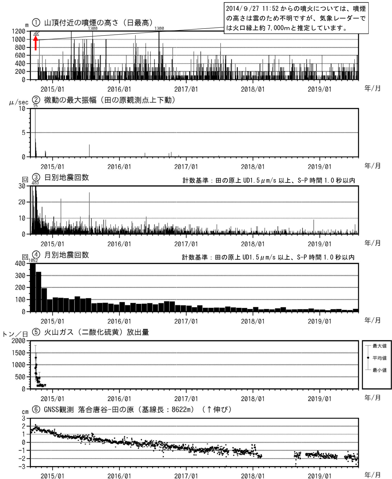
図4 御嶽山 最近の火山活動経過図（2014年9月1日～2019年7月31日）
