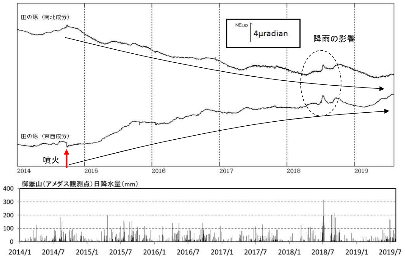
図 7 御嶽山 田の原観測点の傾斜変動（2014 年 1 月 1 日～2019 年 7 月 31 日）
