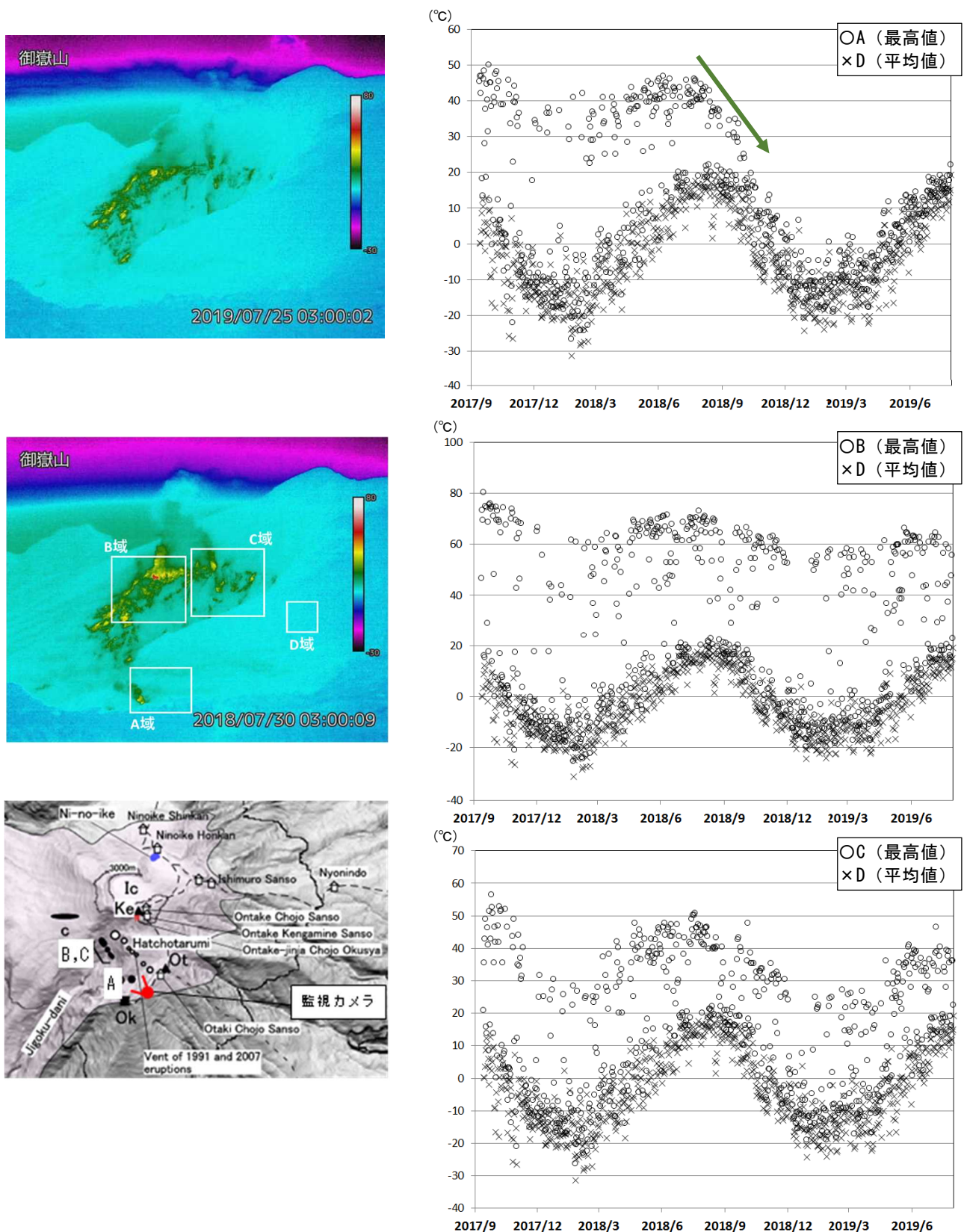
図3 御嶽山 奥の院赤外線熱映像カメラによる剣ヶ峰南西側における最高温度の推移
