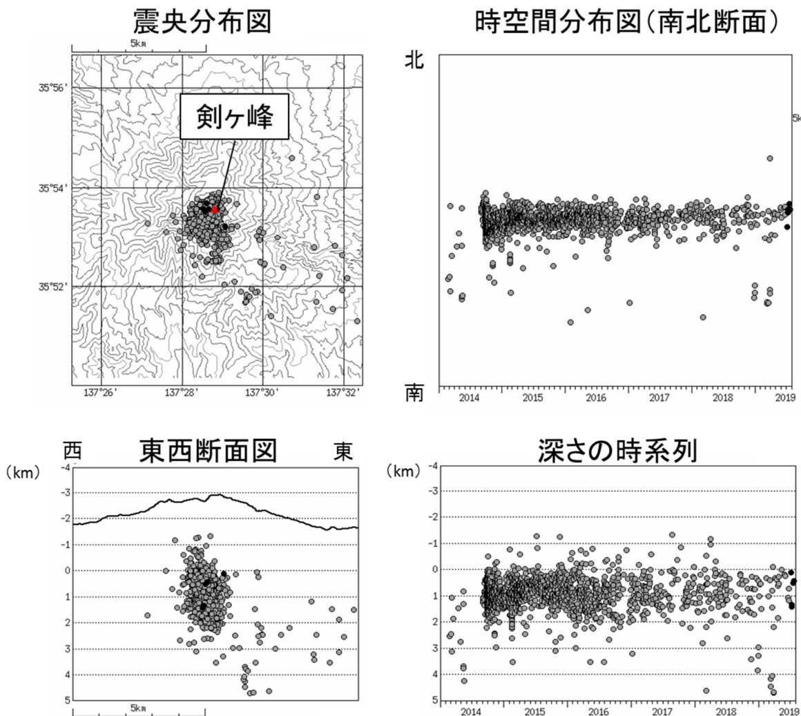
図 2 御嶽山 震源分布図（2014 年 1 月 1 日～2019 年 7 月 31 日）
