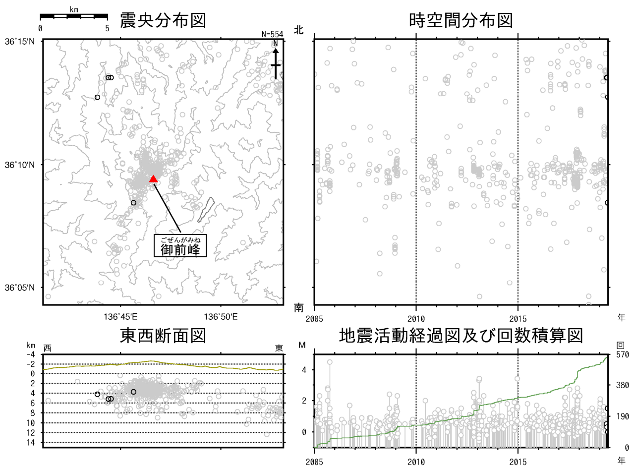
図4 白山 広域地震観測網による山体・周辺の地震活動（2005 年 1 月 1 日～2019 年 5 月 31 日）
