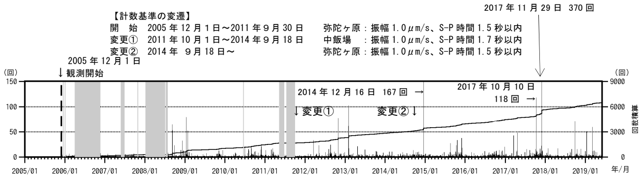
図3 白山 日別地震回数と積算回数（2005 年 12 月 1 日～2019 年 5 月 31 日） 図の灰色部分は機器障害による欠測期間
