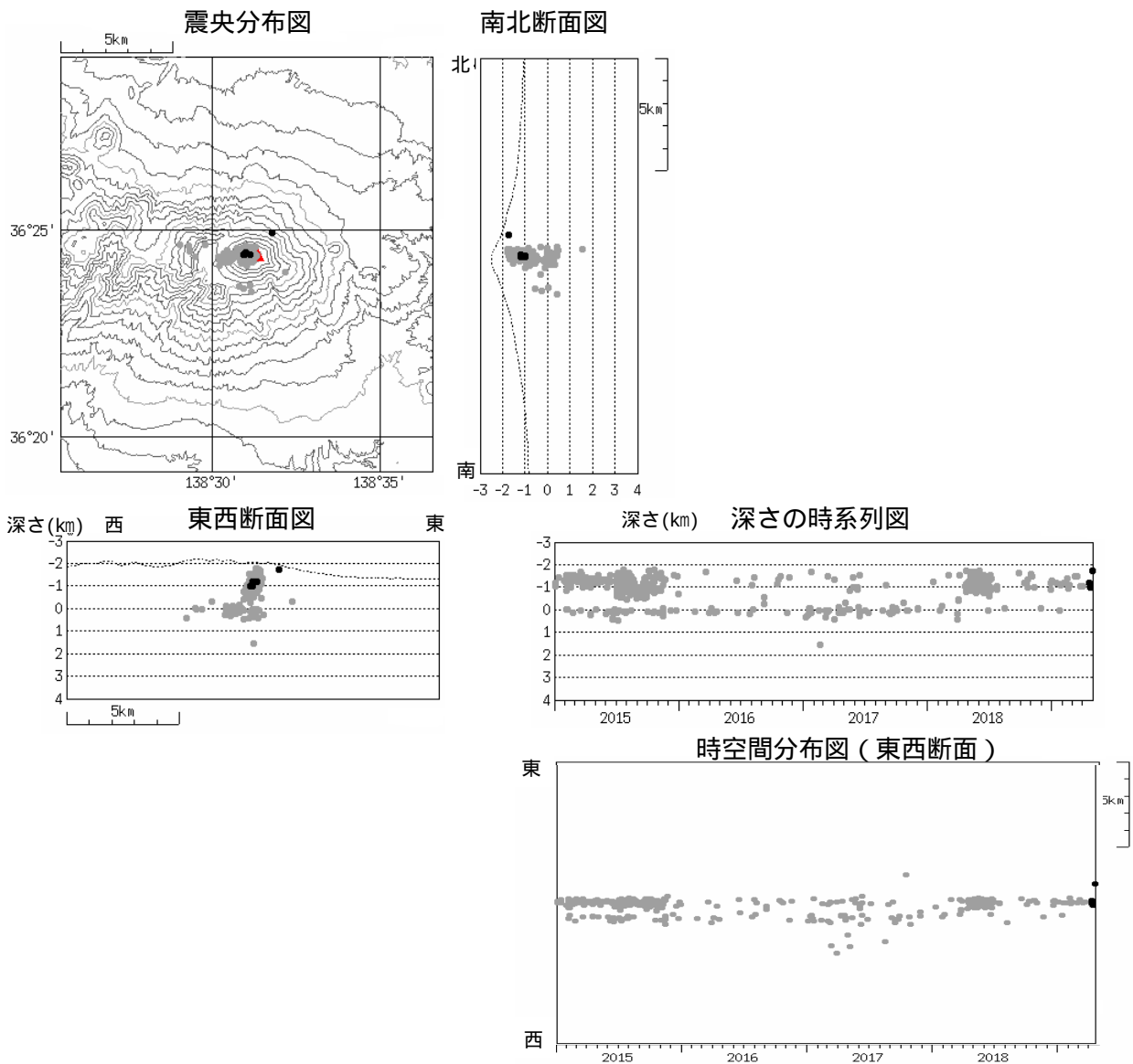
図 6 浅間山 震源分布図（2015 年 1 月 1 日～2019 年 4 月 30 日）
