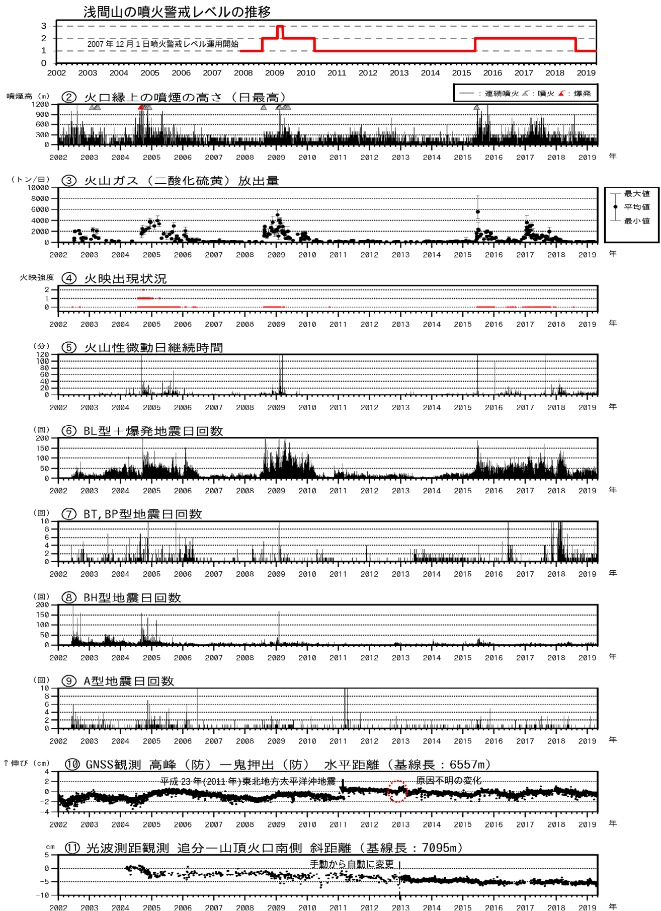
図 3 浅間山 火山活動経過図 (2002 年 1 月 1 日 ~ 2019 年 4 月 30 日)
