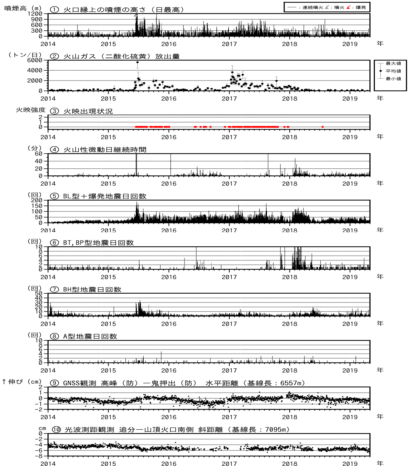
図 4 浅間山 最近の火山活動経過図 (2014 年 1 月 1 日 ~ 2019 年 4 月 30 日)
