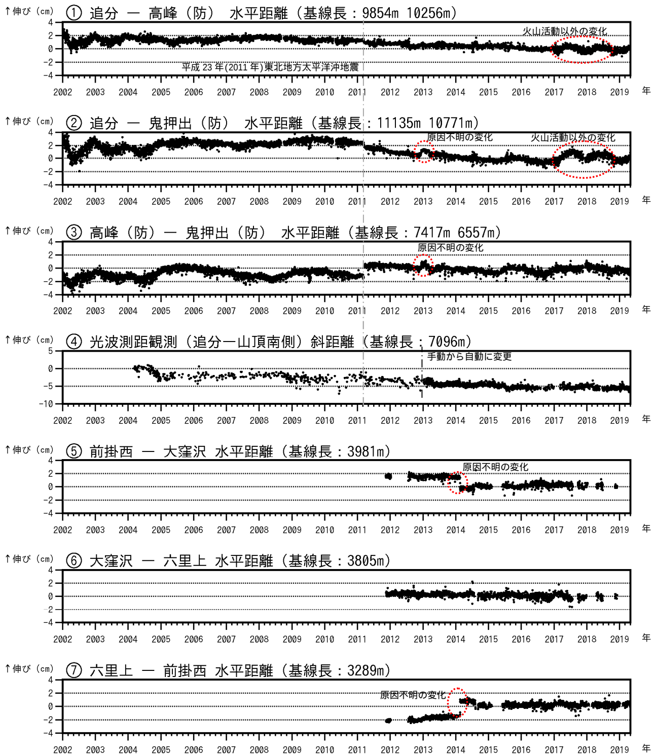
図 7 - 1 浅間山 GNSS 連続観測及び光波測距観測の結果(2002 年 1 月 1 日 ~ 2019 年 4 月 30 日) 2010 年 10 月及び 2016 年 1 月に、解析方法を改良しています。
