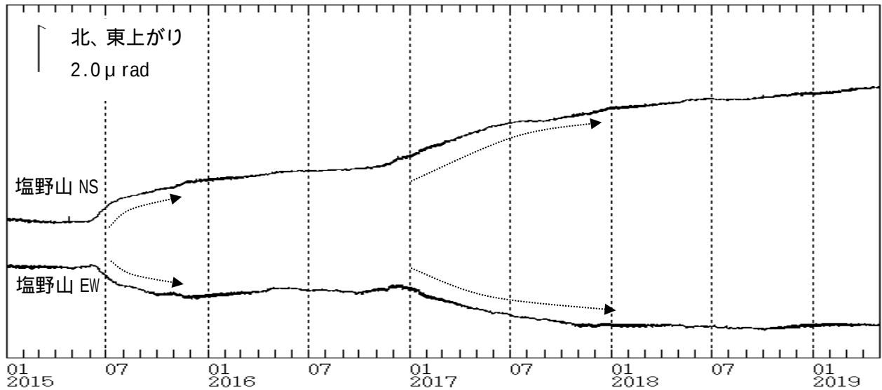
図9 浅間山 塩野山観測点における傾斜データ（2015 年 1 月 1 日～2019 年 4 月 30 日）
