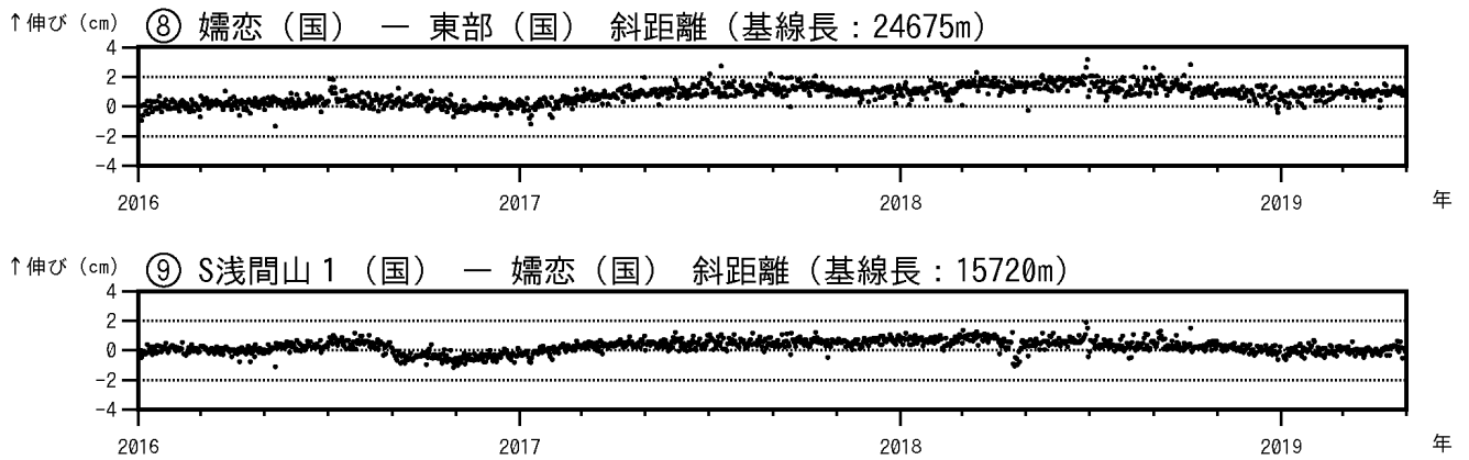
図 7 - 2 浅間山 GNSS 連続観測結果(2016 年 1 月 1 日～2019 年 4 月 30 日)
