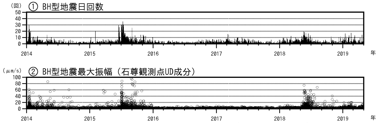
図 5 浅間山 BH型地震の日別回数とその最大振幅（2014 年 1 月 1 日～2019 年 4 月 30 日）
