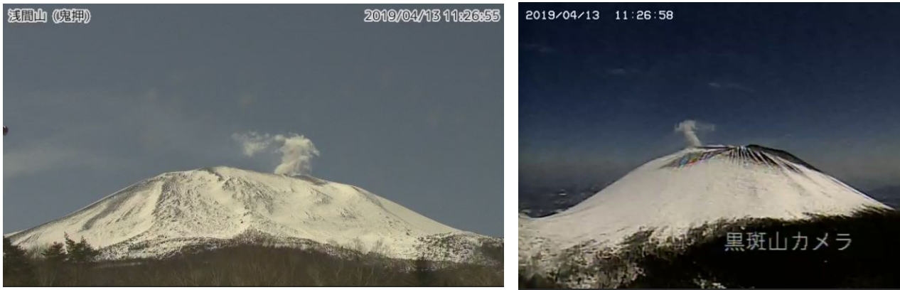
図 1 浅間山 山頂部の状況
