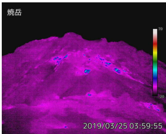
図 6 焼岳 中尾峠赤外熱映像カメラによる焼岳の北側斜面の地表面温度分布（左図）と可視画像（右図） 撮影場所と撮影方向は図 8 を参照下さい。 ・噴気の状態や地表面温度分布に特段の変化は認められません。
