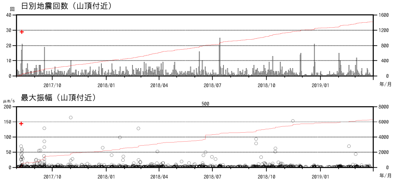
図2 焼岳 山頂付近の地震回数、および南峰南東観測点上下動最大振幅 (2017年8月1日～2019年3月31日)
