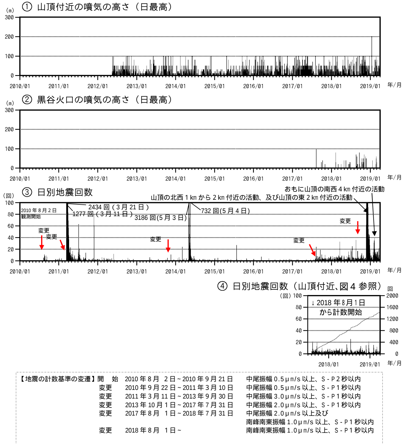
図 1 焼岳 噴気の高さと地震回数の推移(2010 年 1 月 1 日 ~ 2019 年 3 月 31 日)
