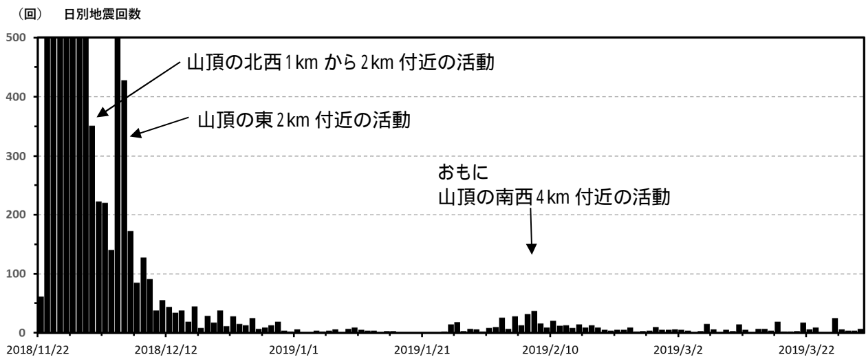
図3 焼岳 焼岳周辺の日別地震回数(2018年11月22日～2019年3月31日)
