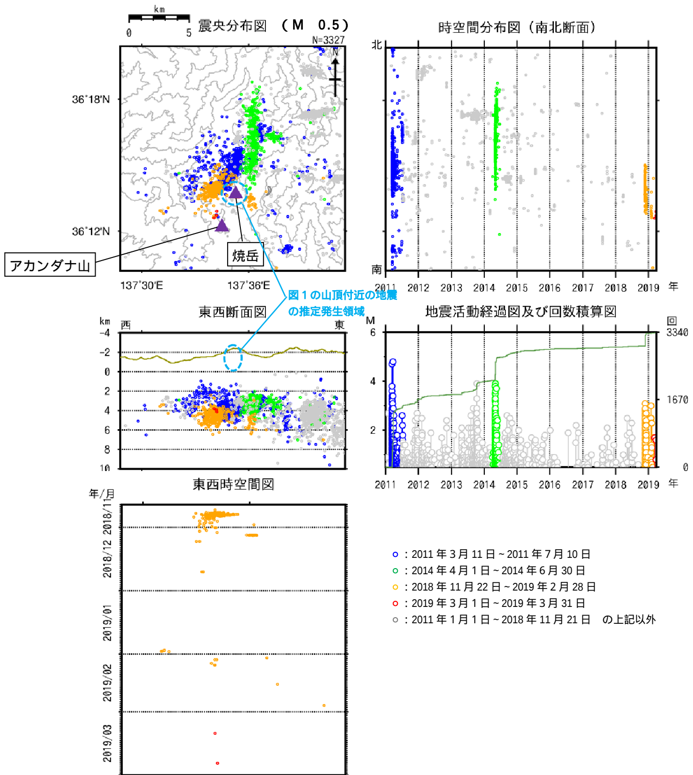
図 4 焼岳 広域地震観測網による山体及び周辺の地震活動(2011年 1 月 1 日 ~ 2019年 3 月 31 日)
