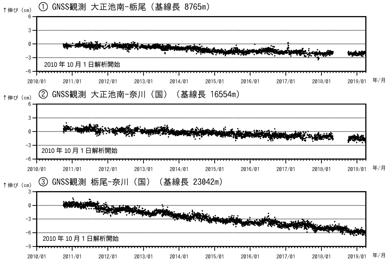
図7 焼岳 GNSS連続観測による基線長変化（2010年10月1日～2019年3月31日）
