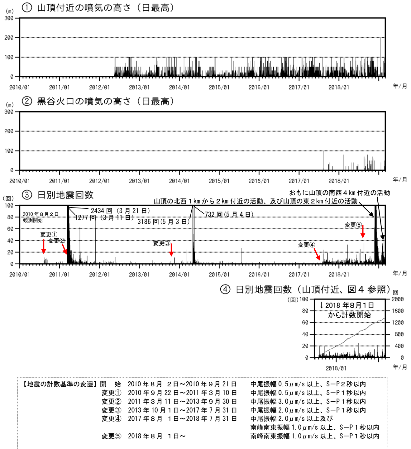
図1 焼岳 噴気の高さと地震回数の推移(2010年1月1日～2019年2月28日)
