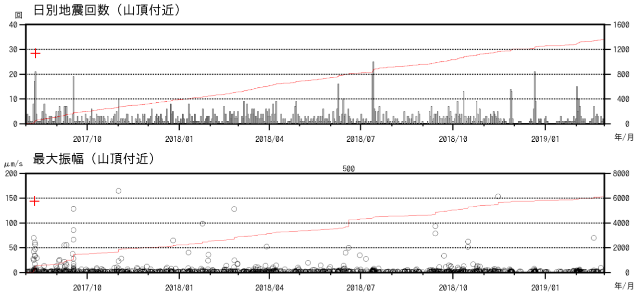
図2 焼岳 山頂付近の地震回数、および南峰南東観測点上下動最大振幅 (2017年8月1日～2019年2月28日)
