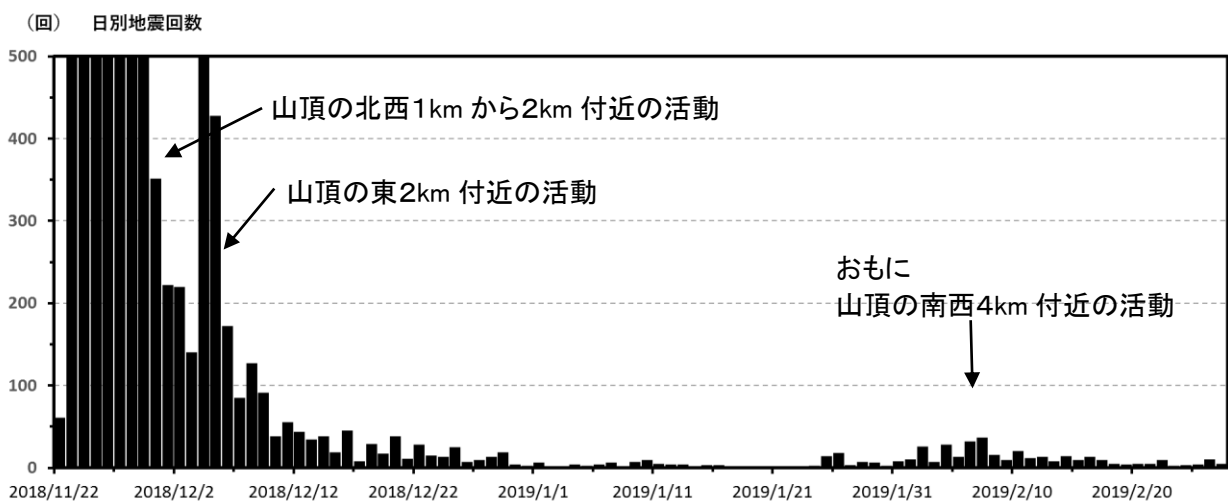
図3 焼岳 焼岳周辺の日別地震回数(2018年11月22日～2019年2月28日)
