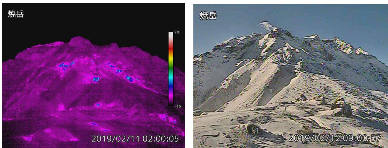
図6 焼岳 中尾峠赤外熱映像カメラによる焼岳の北側斜面の地表面温度分布（左図）と可視画像（右図） 撮影場所と撮影方向は図8を参照下さい。 ・噴気の状態や地表面温度分布に特段の変化は認められません。
