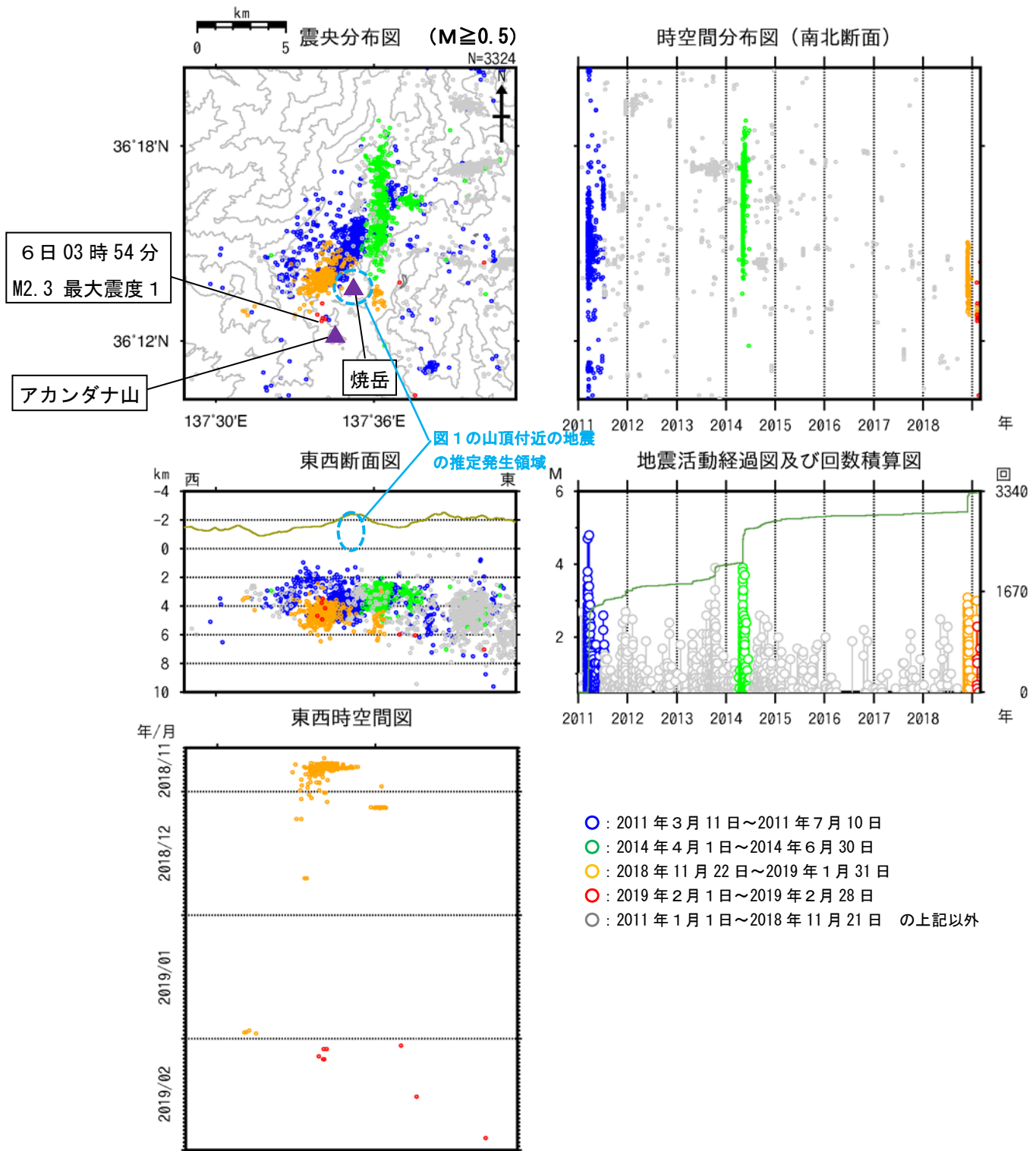
図4 焼岳 広域地震観測網による山体及び周辺の地震活動(2011年1月1日～2019年2月28日)
