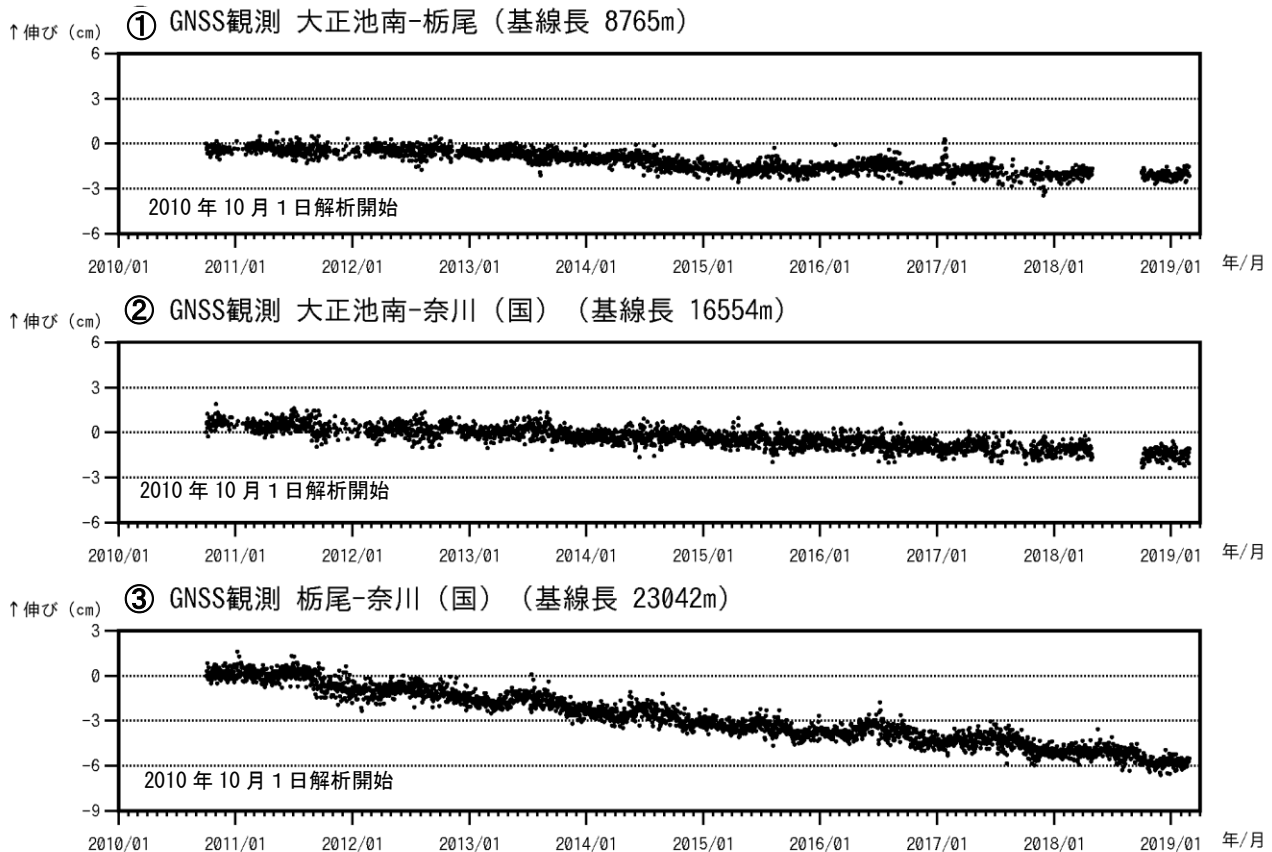
図7 焼岳 GNSS 連続観測による基線長変化（2010 年 10 月 1 日～2019 年 2 月 28 日）
