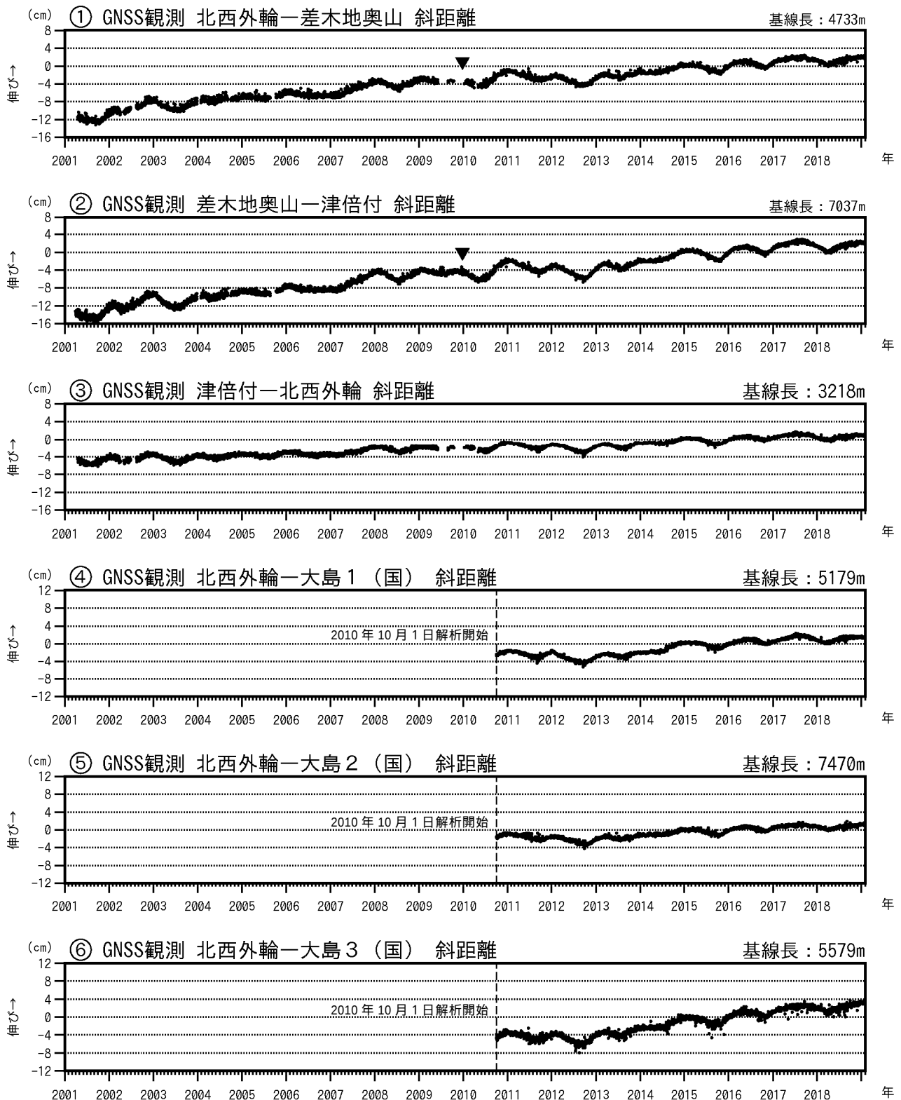
図3 伊豆大島 GNSS連続観測による基線長変化(2001年1月～2019年1月31日)
