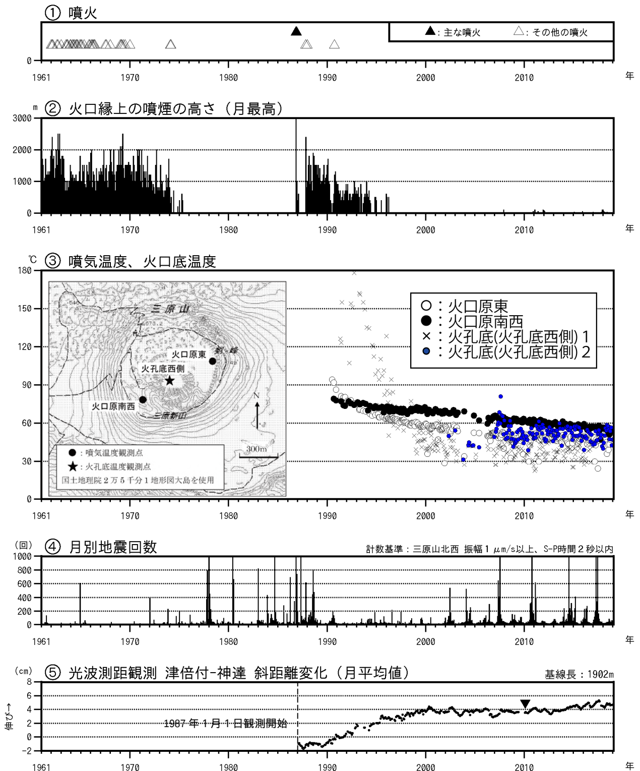
図 1 伊豆大島 長期間の火山活動経過図（1961 年 1 月～2019 年 1 月 31 日）
