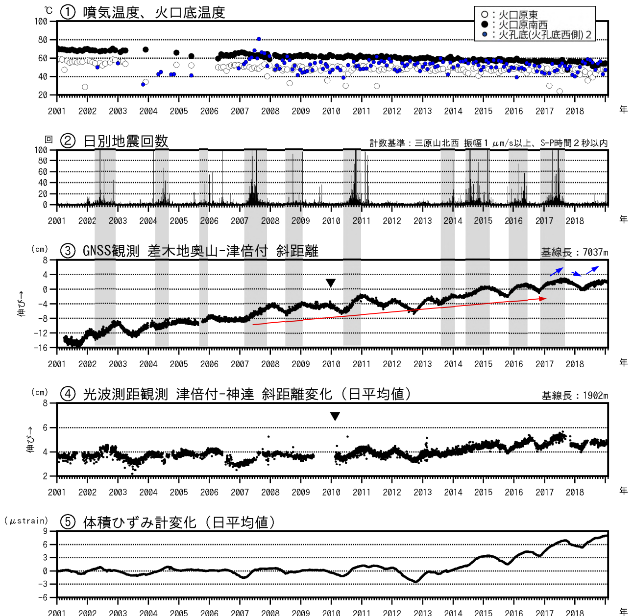
図 2 伊豆大島 最近の火山活動経過図（2001 年 1 月～2019 年 1 月 31 日）
