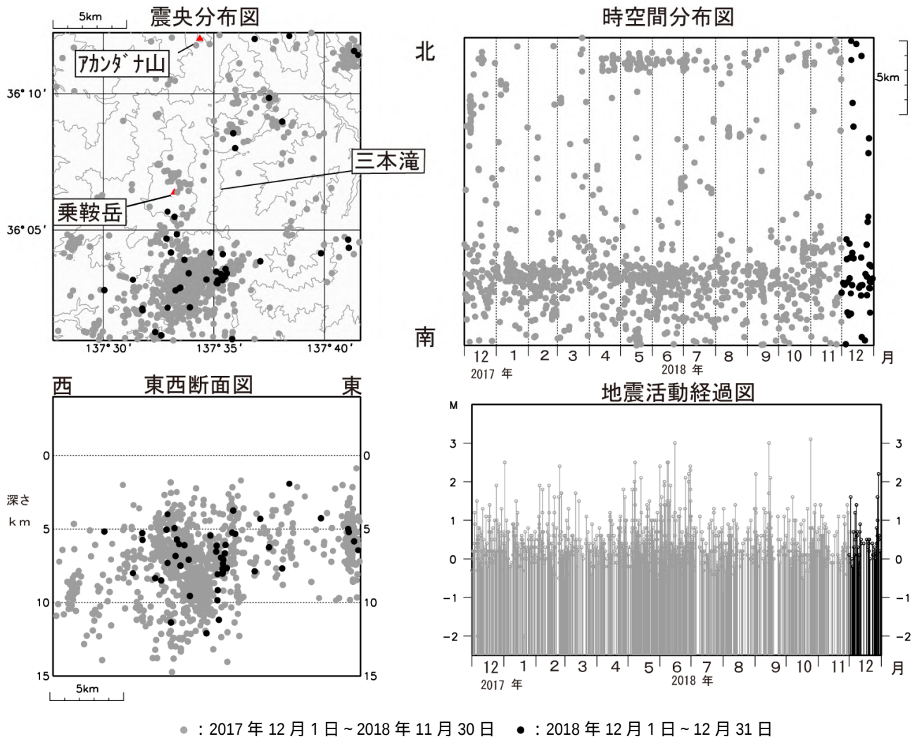
図 3 乗鞍岳 広域地震観測網による山体・周辺の地震活動(2017 年 12 月 1 日～2018 年 12 月 31 日) 広域地震観測網により震源決定したもので、深さは全て海面以下として決定しています。M（マグニチュード） は地震の規模を表します。図中の震源要素は一部暫定値が含まれており、後日変更することがあります。 ・乗鞍岳付近の地震活動は、低調に経過しています。 ・乗鞍岳から南方へ約 6 km 離れたところでまとまった地震活動がみられますが、乗鞍岳の火山活動とは関係ないとみています。
